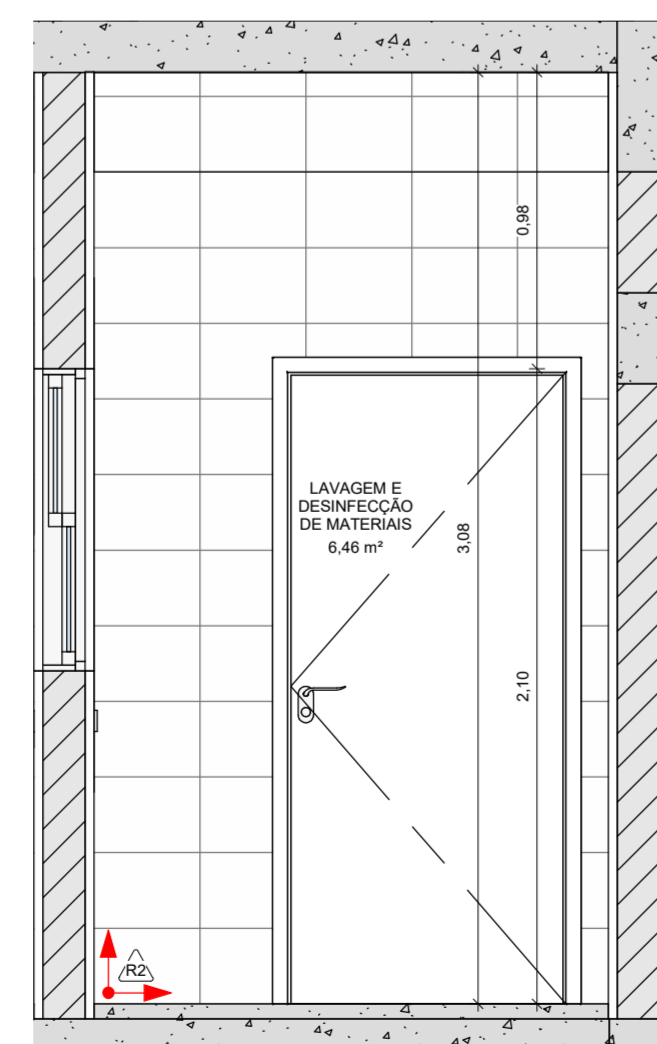
14 PAGINAÇÃO LAVAGEM E DESINFECÇÃO DE MATERIAIS (3) 1 : 25
