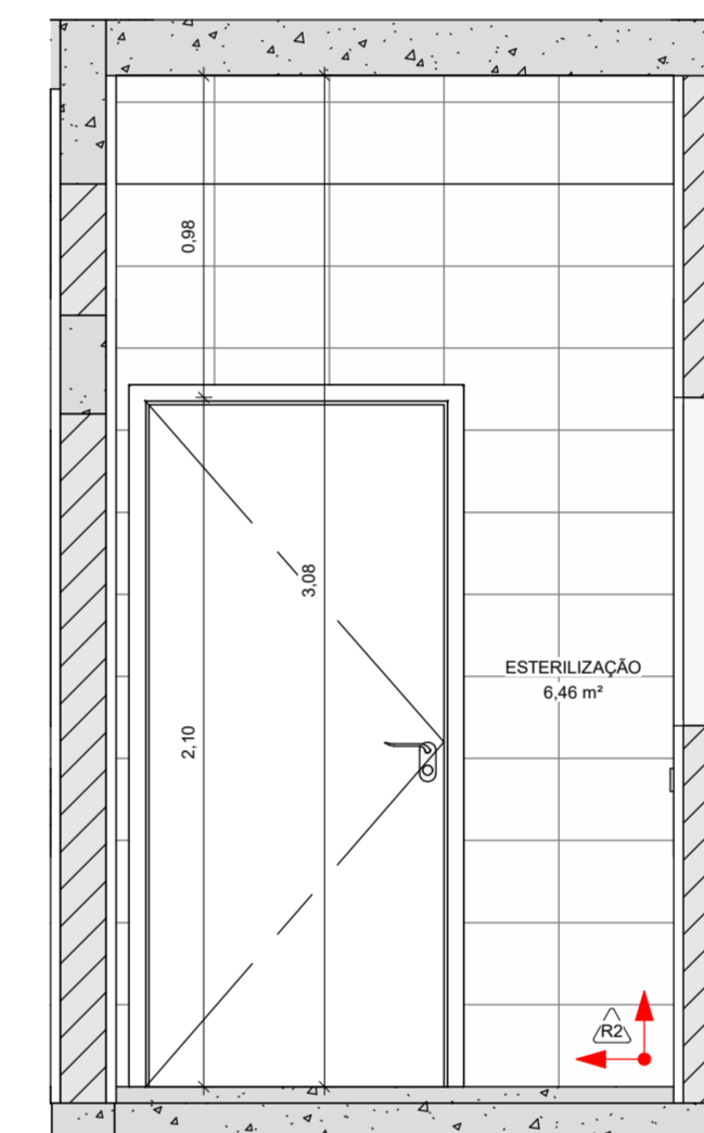
11 PAGINAÇÃO ESTERELIZAÇÃO (3) 1 : 25
