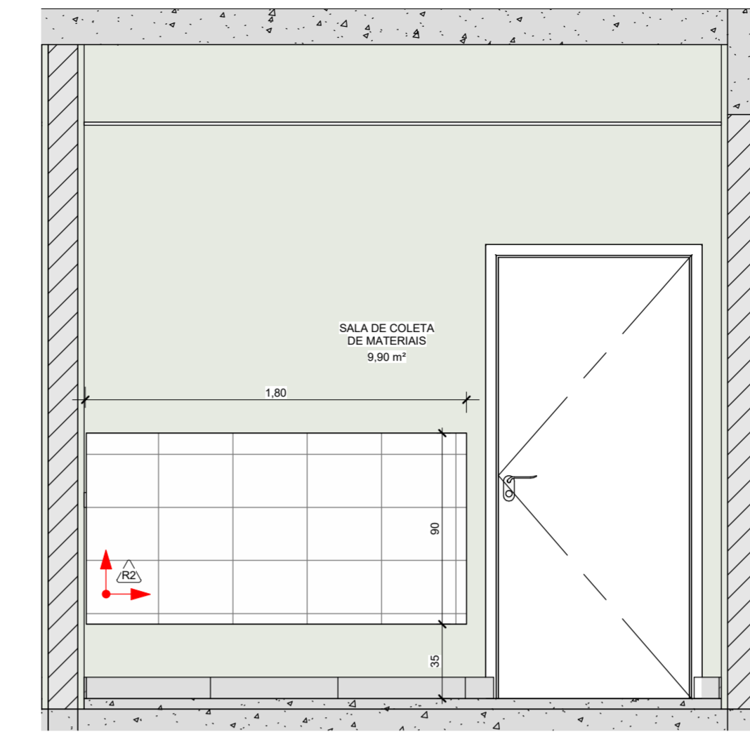
5 PAGINAÇÃO SALA DE COLETA DE MATERIAIS 1 : 25
