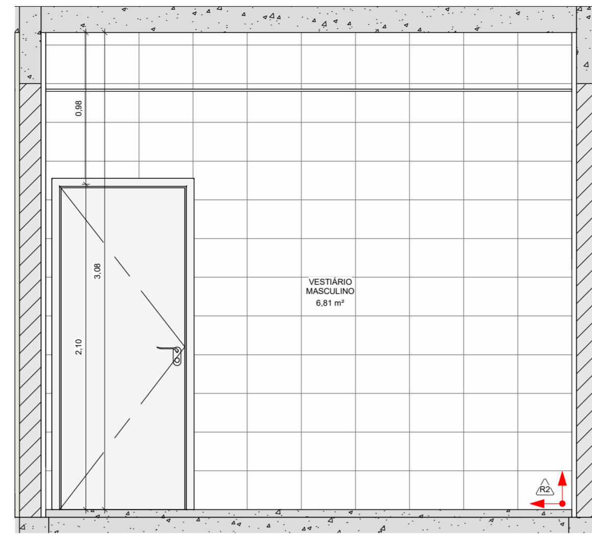
4 PAGINAÇÃO VESTIÁRIO MASCULINO (4) 1 : 25
