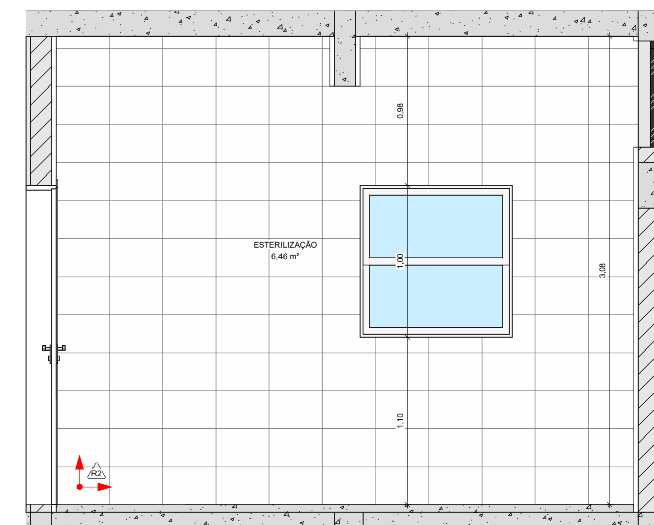
17 PAGINAÇÃO ESTERELIZAÇÃO (4) 1 : 25
