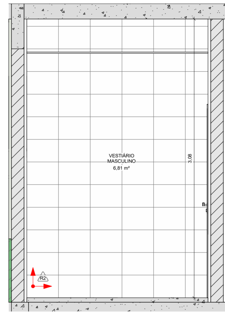
3 PAGINAÇÃO VESTIÁRIO MASCULINO (3) 1 : 25
