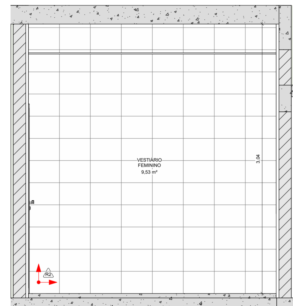
8 PAGINAÇÃO VESTIÁRIO FEMININO (3) 1 : 25
