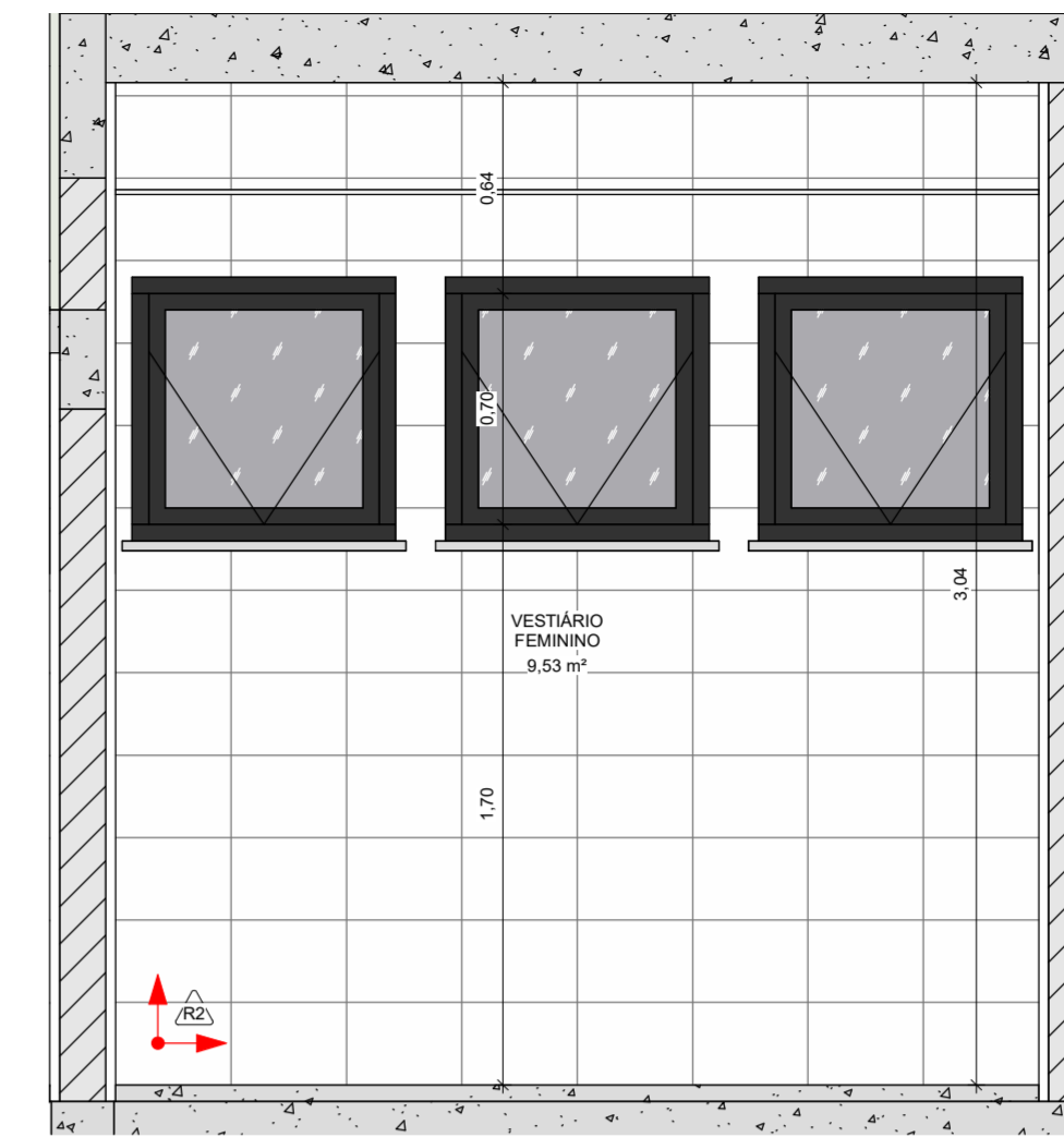
6 PAGINAÇÃO VESTIÁRIO FEMININO (1) 1 : 25
