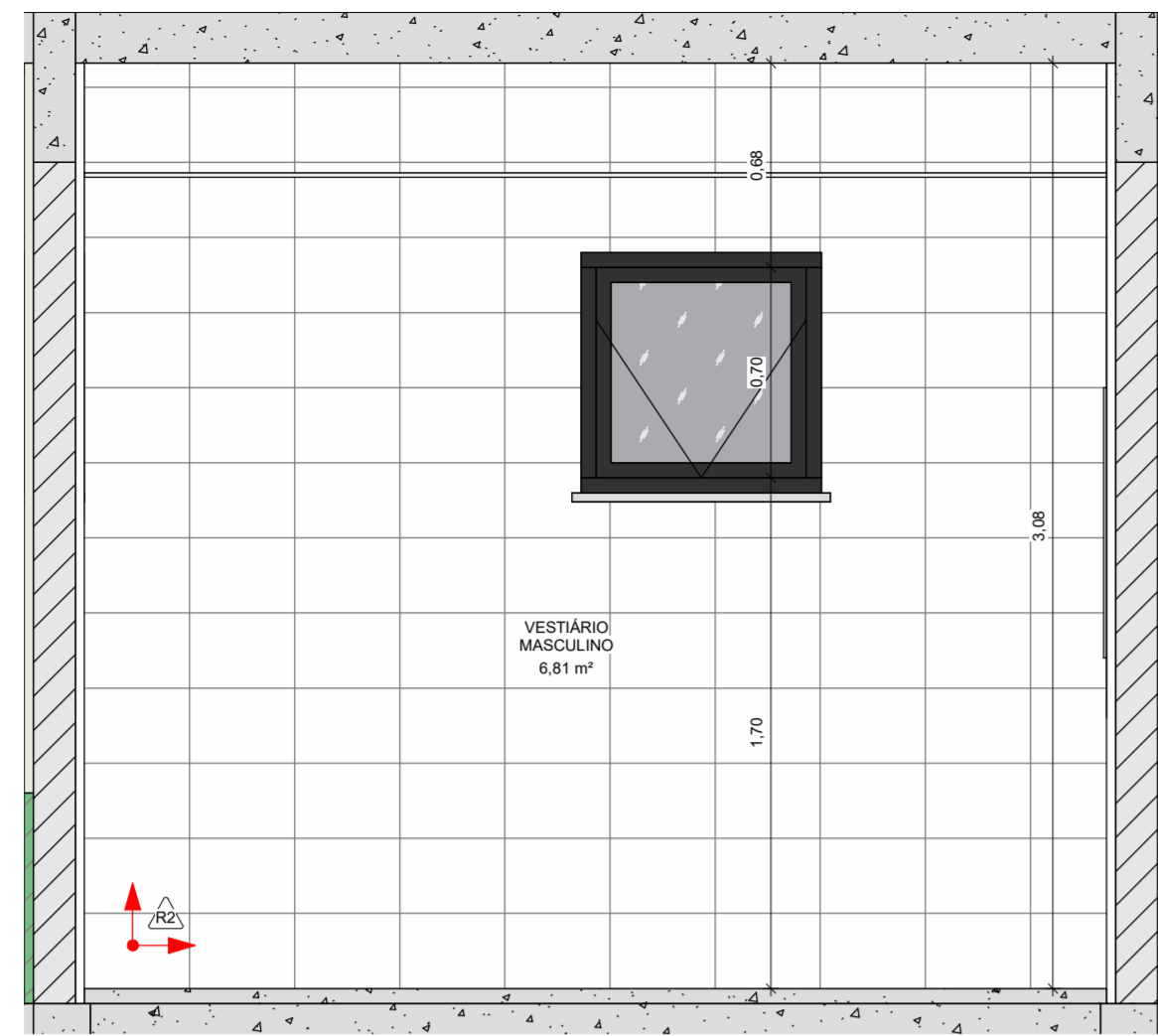
2 PAGINAÇÃO VESTIÁRIO MASCULINO (2) 1 : 25
