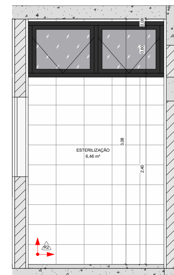
16 PAGINAÇÃO ESTERELIZAÇÃO (1) 1 : 25
