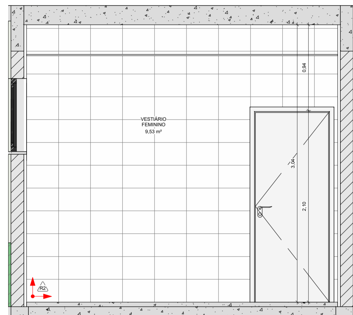
7 PAGINAÇÃO VESTIÁRIO FEMININO (2) 1 : 25
