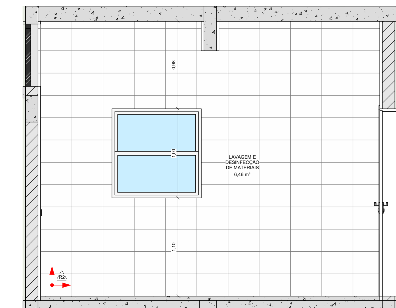
13 PAGINAÇÃO LAVAGEM E DESINFECÇÃO DE MATERIAIS (2) 1 : 25
