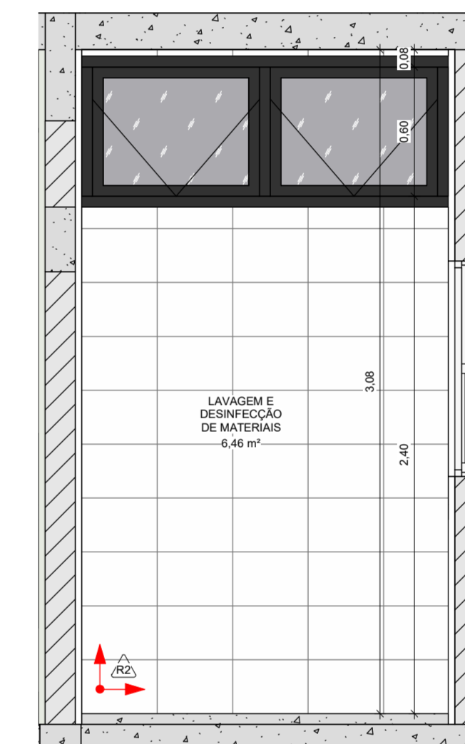
12 PAGINAÇÃO LAVAGEM E DESINFECÇÃO DE MATERIAIS (1) 1 : 25
