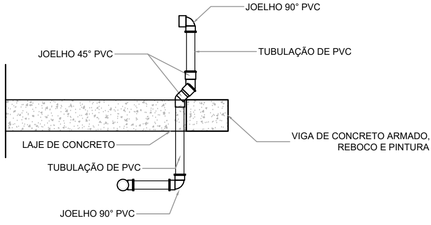
DETALHE DO DESVIO DE VIGAS SEM ESCALA
