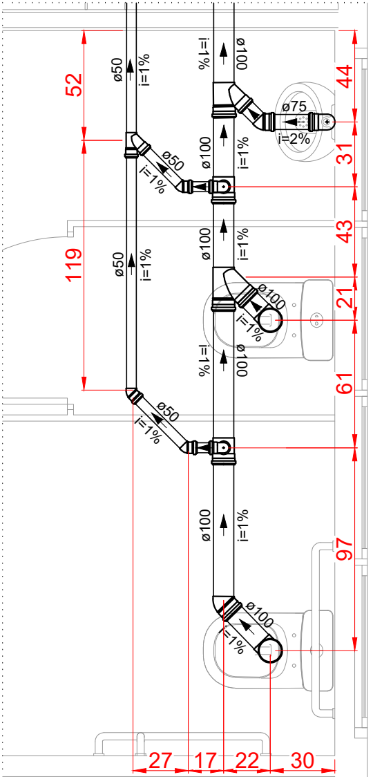
DETALHE SAN-1 ESCALA 1:25
