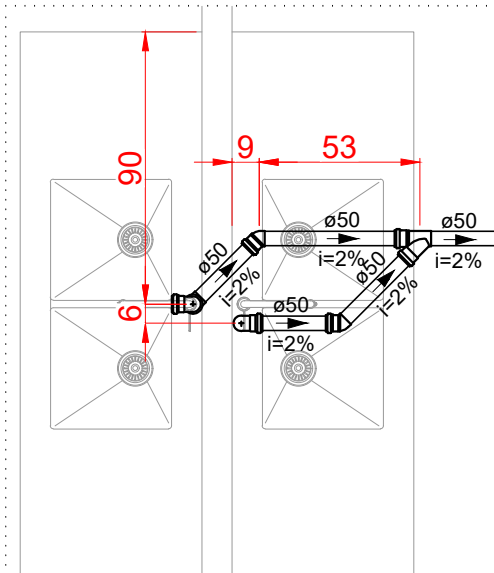
DETALHE SAN-5 ESCALA 1:25
