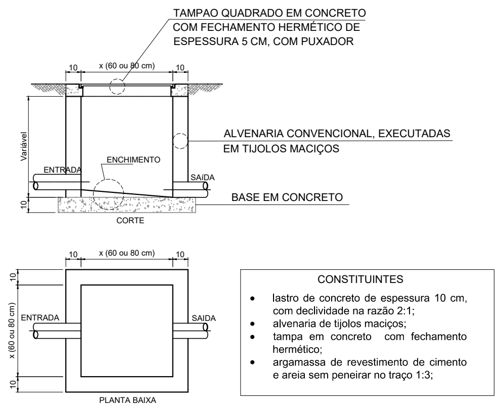
DETALHE DA CAIXA DE INSPEÇÃO SEM ESCALA
