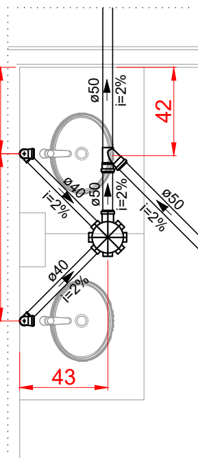
DETALHE SAN-4 ESCALA 1:25
