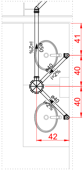
DETALHE SAN-3 ESCALA 1:25
