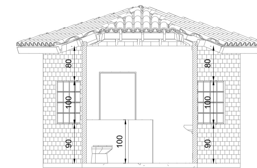
CORTE HH Escala: 1:75
