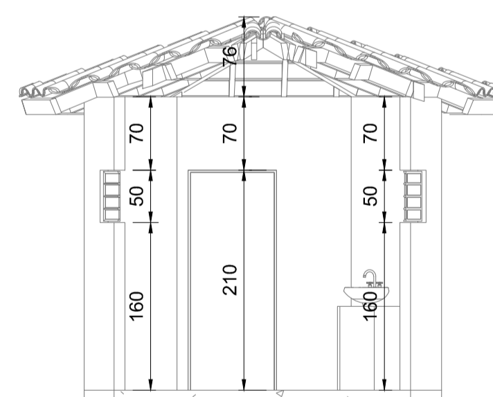
CORTE LL Escala: 1:75
