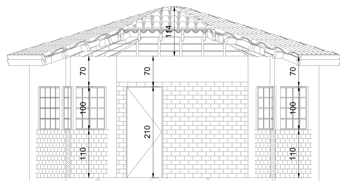
CORTE KK Escala: 1:75
