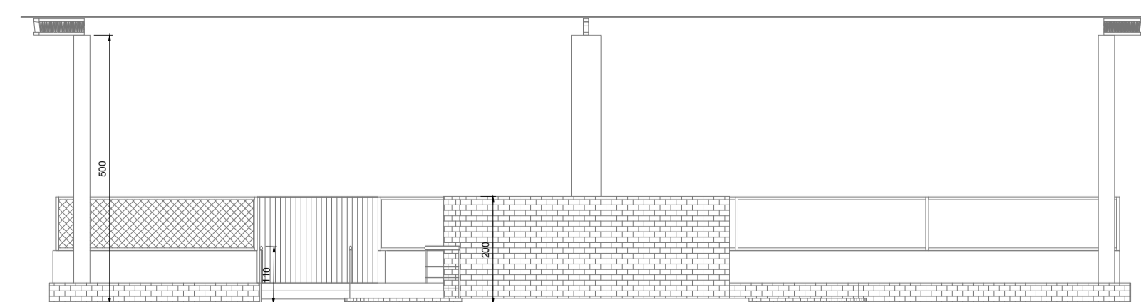
CORTE NN Escala: 1:100
