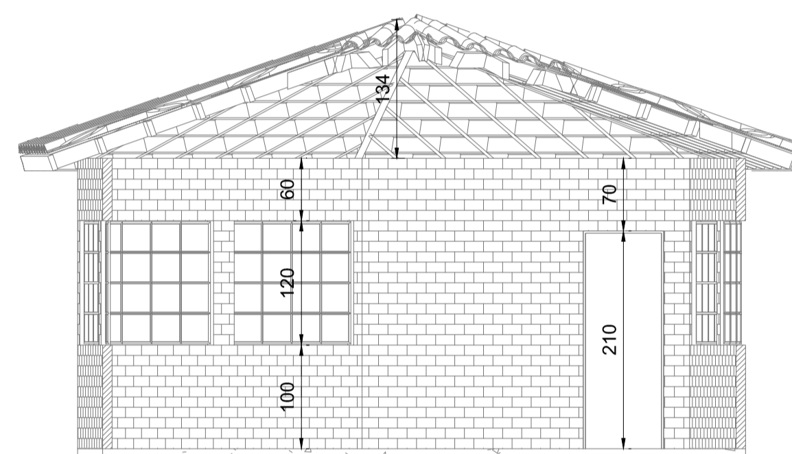
CORTE DD Escala: 1:75
