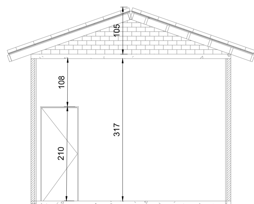
CORTE BB Escala: 1:75
