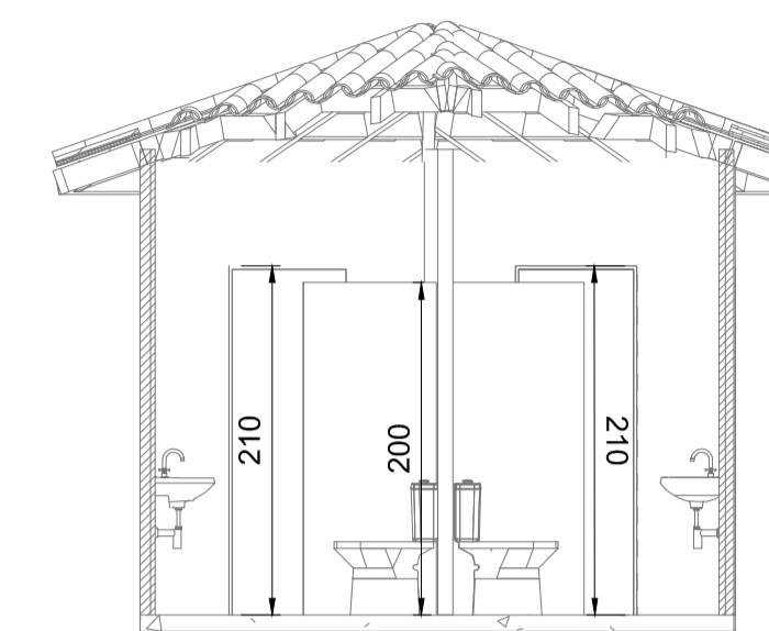
CORTE FF Escala: 1:75
