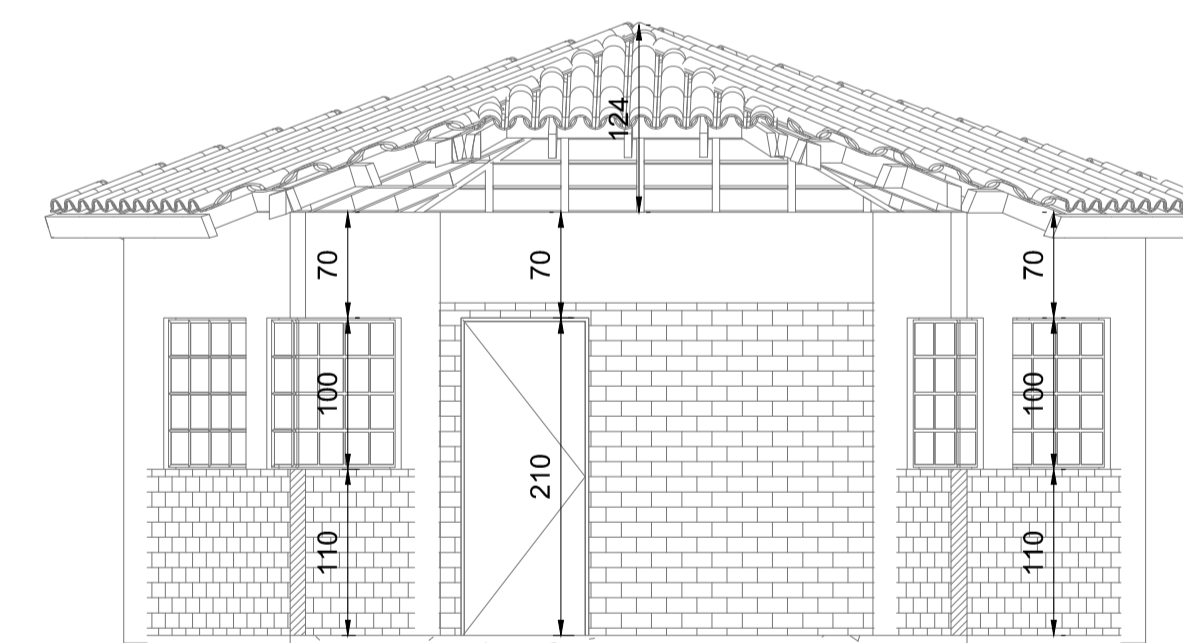
CORTE MM Escala: 1:75
