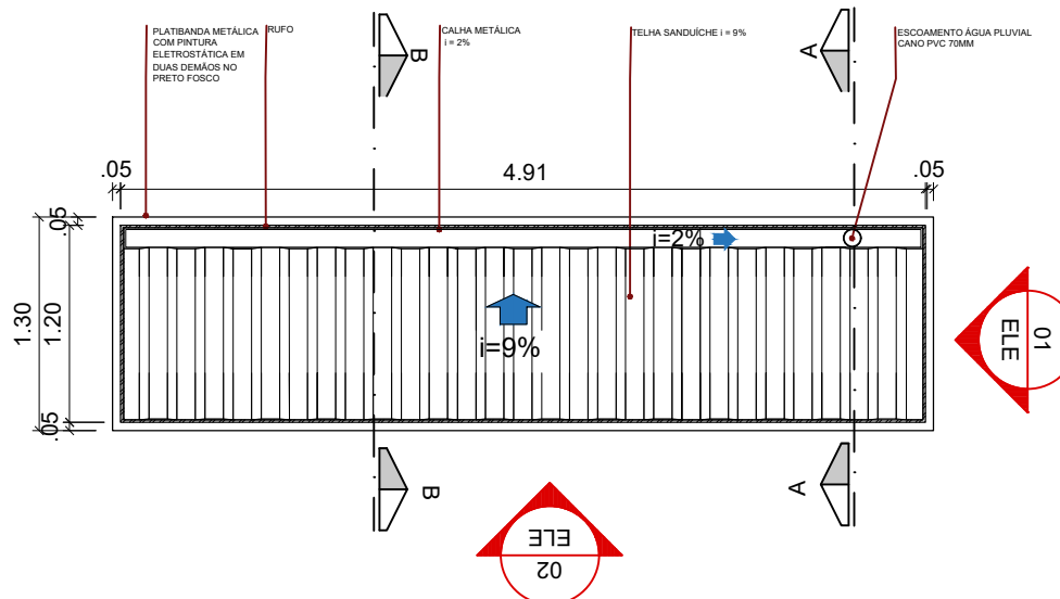
02 PLANTA COBERTURA ABRIGO SIMPLES TIPO 01 ESC. 1:50
