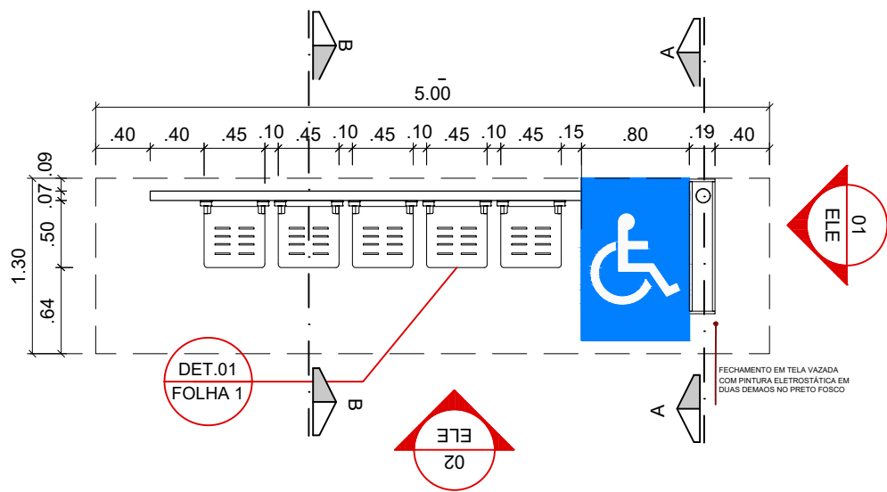
01 PLANTA ABRIGO SIMPLES TIPO 01 ESC. 1:50
