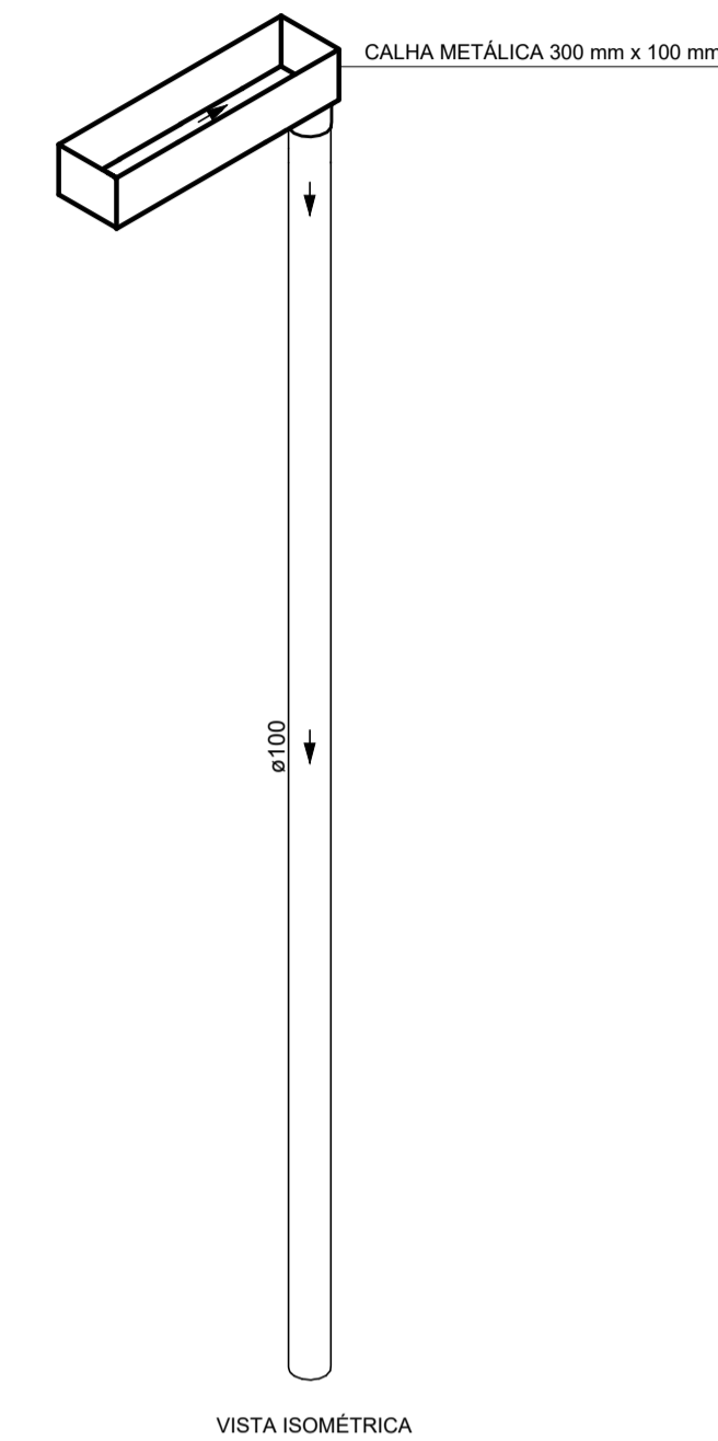
DETALHE DE INSTALAÇÃO DA CALHA ESCALA 1:25
