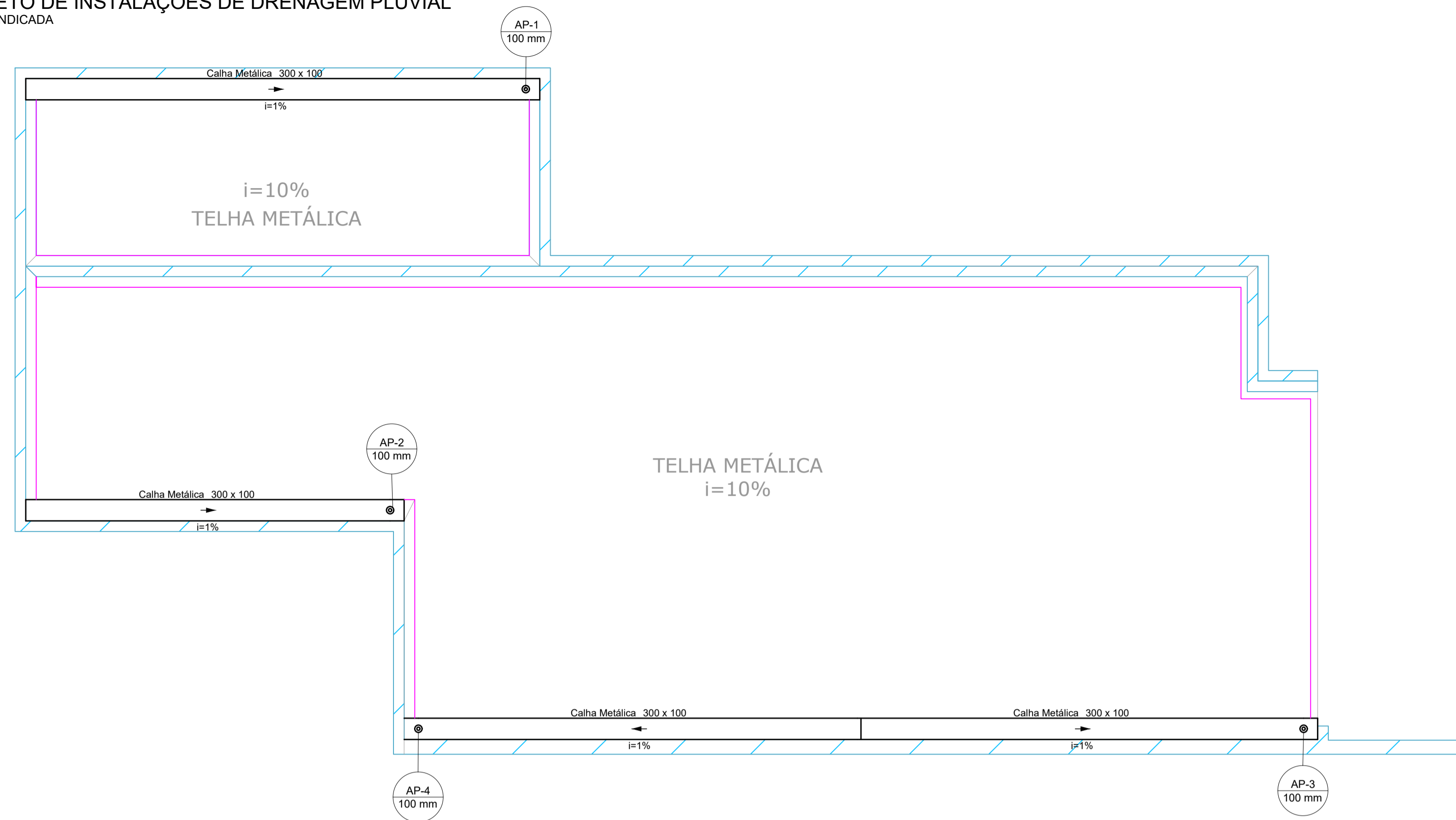
PLANTA BAIXA - COBERTURA ESCALA 1:50
