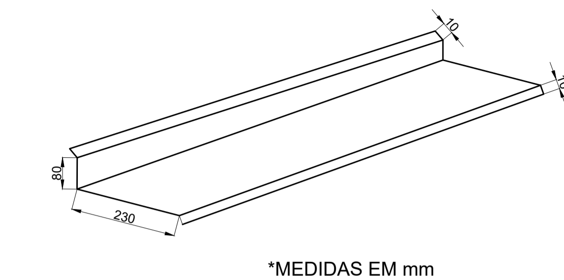
DETALHE DO RUFO EXTERNO SEM ESCALA
