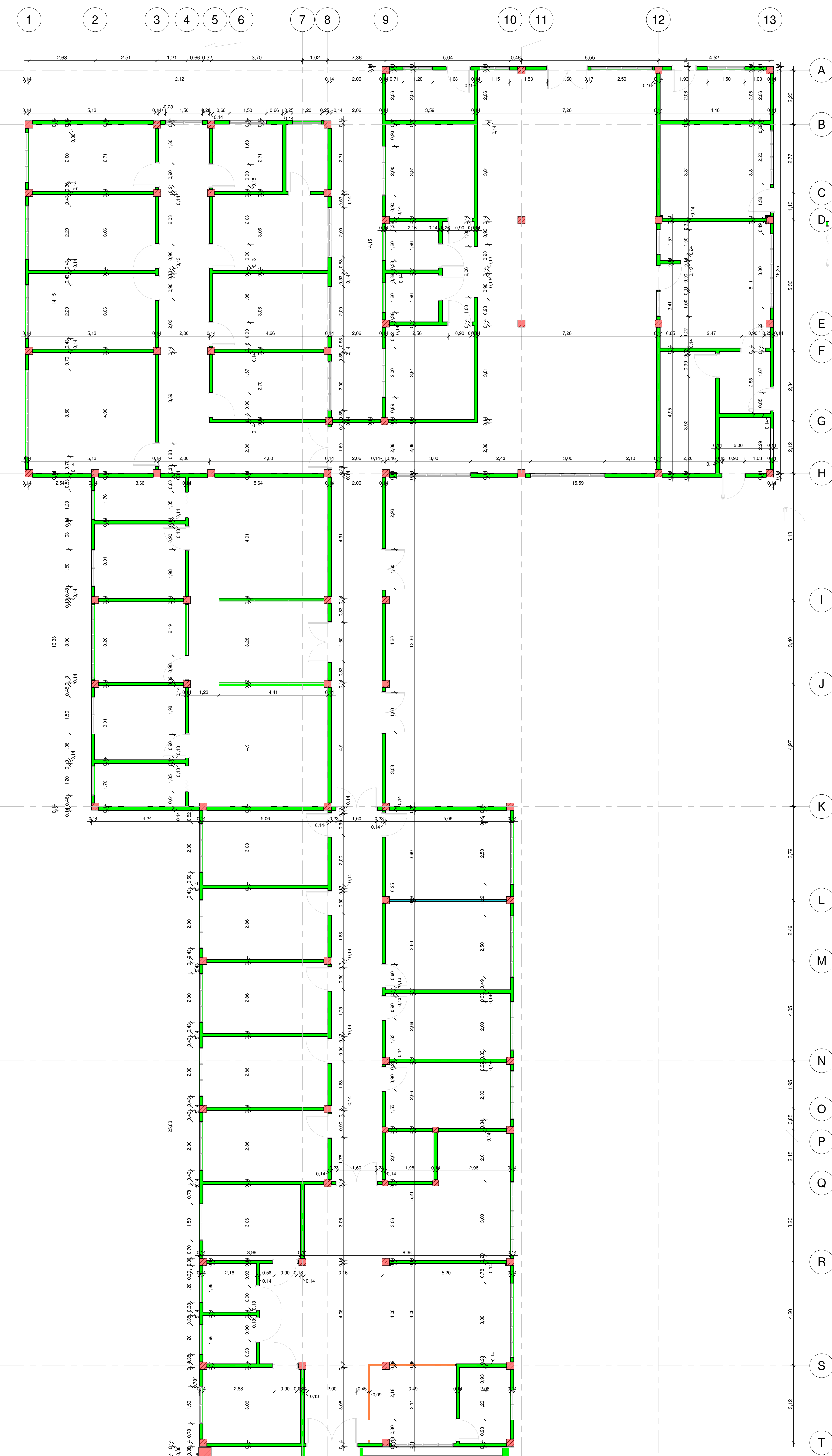
2 PLANTA DE ALVENARIA TÉRREO 1 : 75
