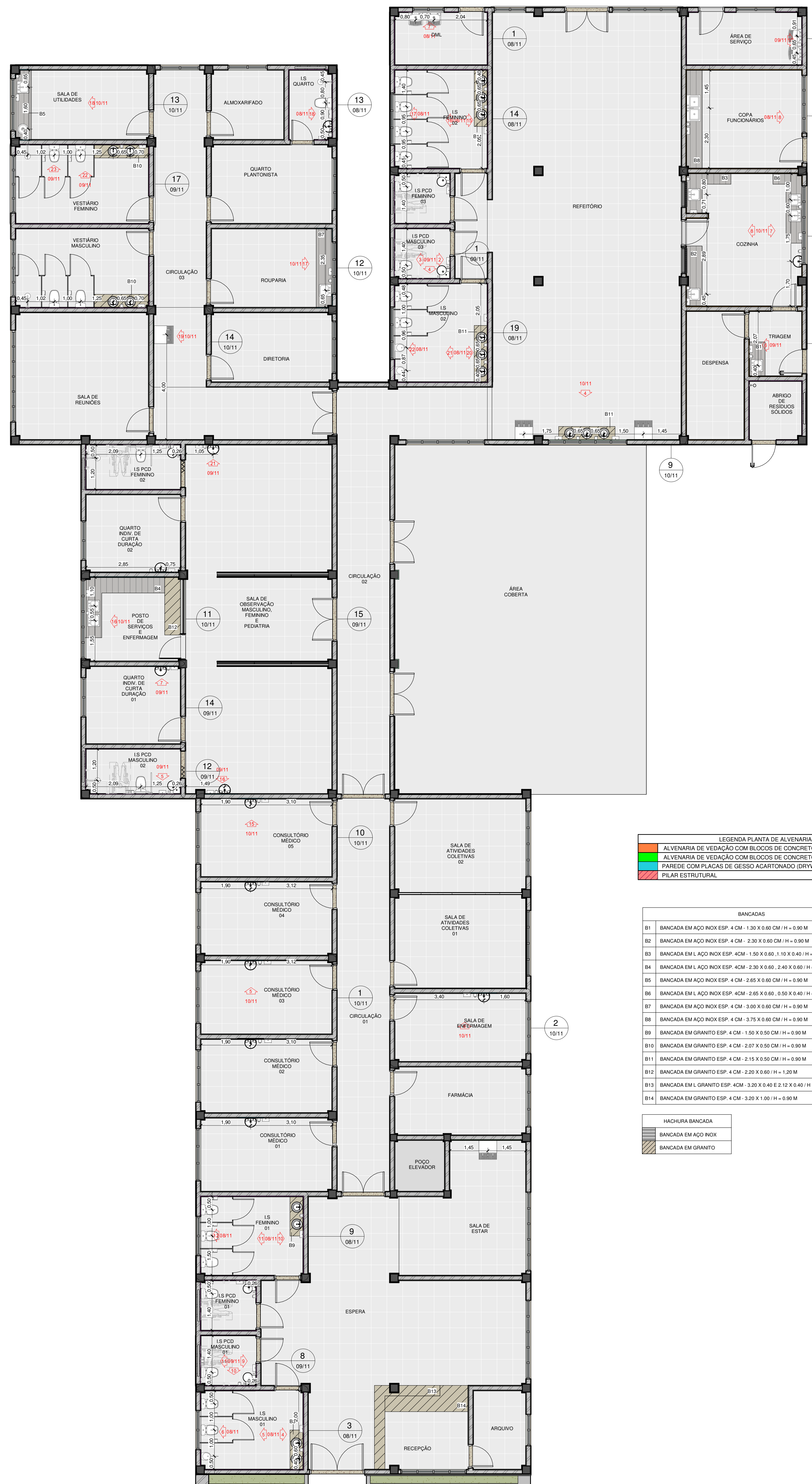
1 PLANTA DE EIXO HIDRÁULICO 1 : 75
