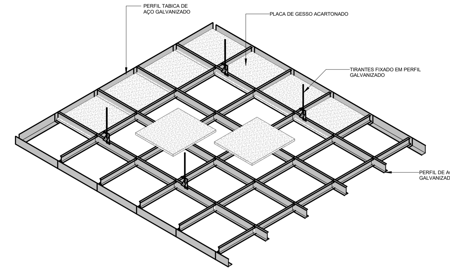
2 DETALHE DE FORRO 1 : 25
