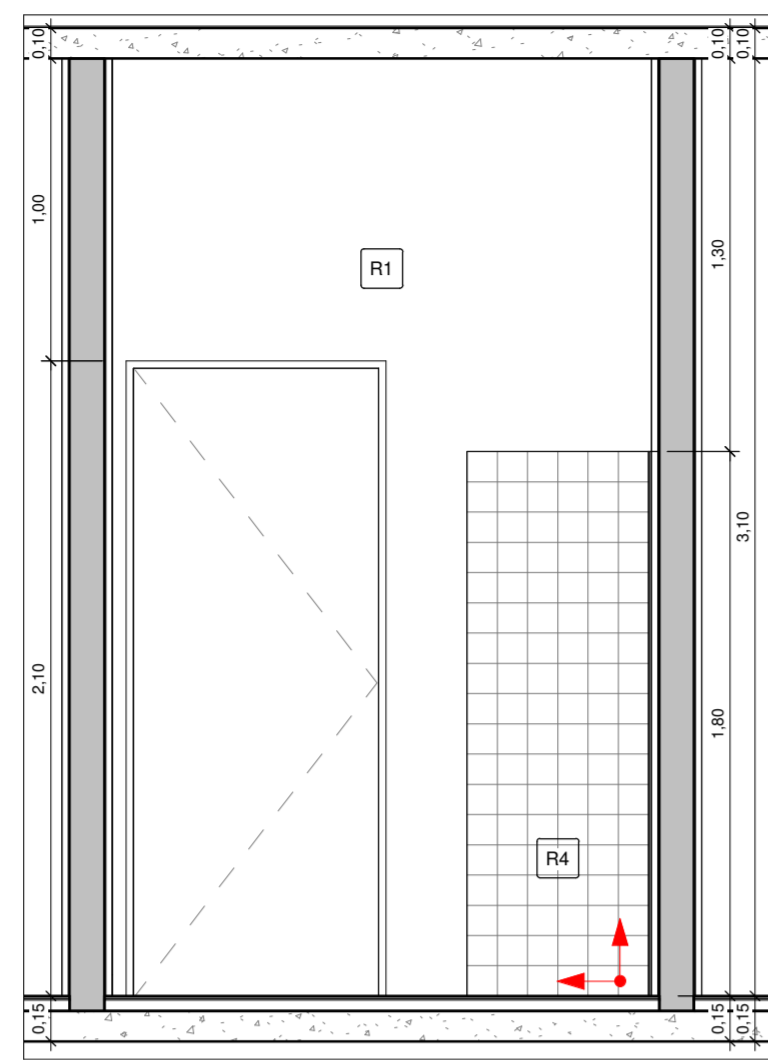
2 ESCOVÓDROMO VISTA 3 1 : 25
