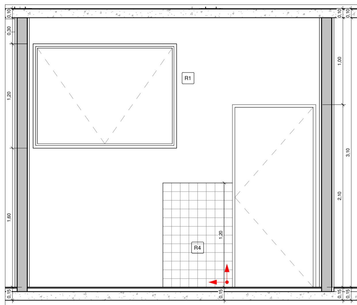
7 CONSULTÓRIO GINECOLÓGICO VISTA 1 1 : 25
