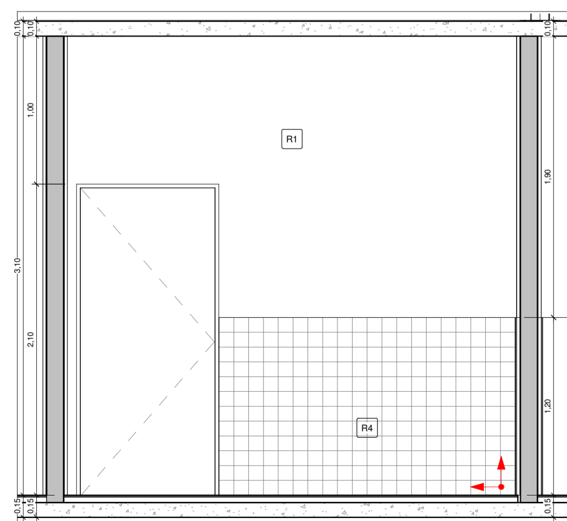
11 VACINAÇÃO VISTA 2 1 : 25
