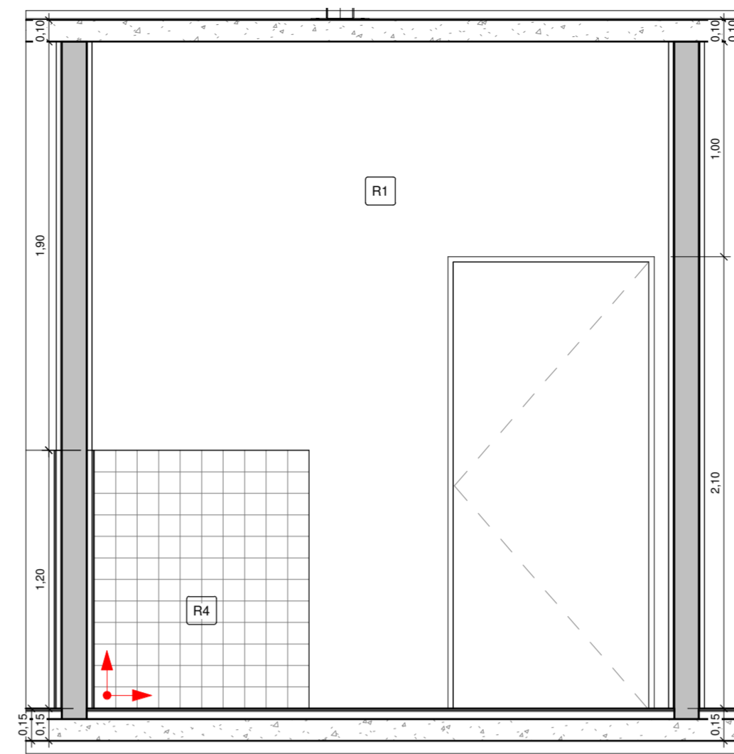
4 CONSULTÓRIO 5 VISTA 2 1 : 25
