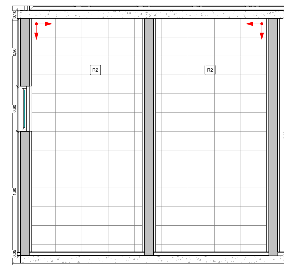
14 BANHEIROS RECEPÇÃO VISTA 3 1 : 25
