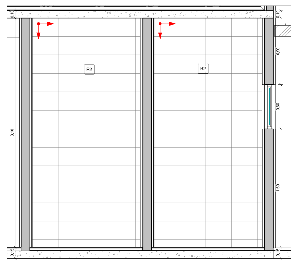
12 BANHEIROS RECEPÇÃO VISTA 1 1 : 25
