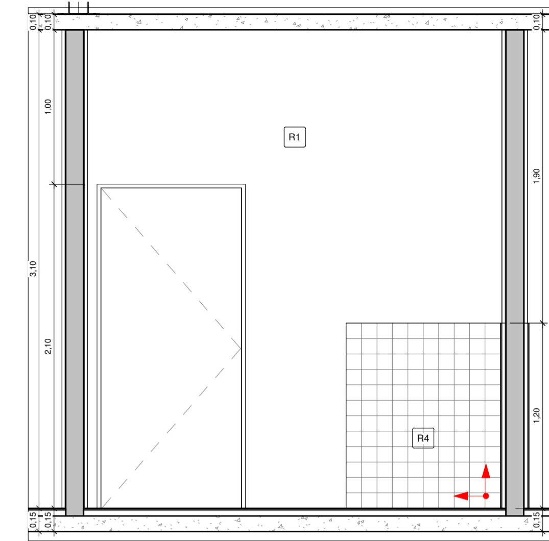
6 CONSULTÓRIO 6 VISTA 2 1 : 25
