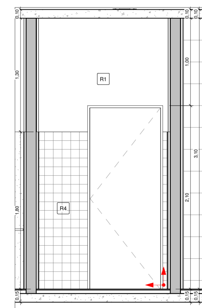
15 LAVAGEM E DESINFECÇÃO VISTA 4 1 : 25
