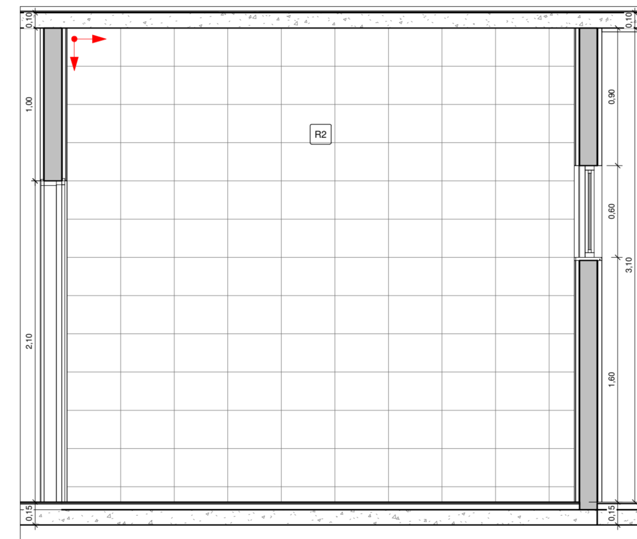
8 VEST. F. VISTA 1 1 : 25
