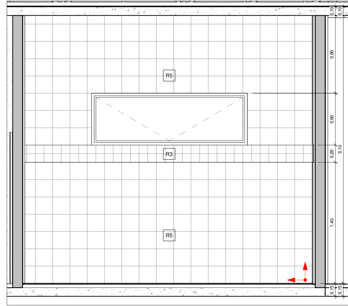
1 COPA VISTA 1 1 : 25
