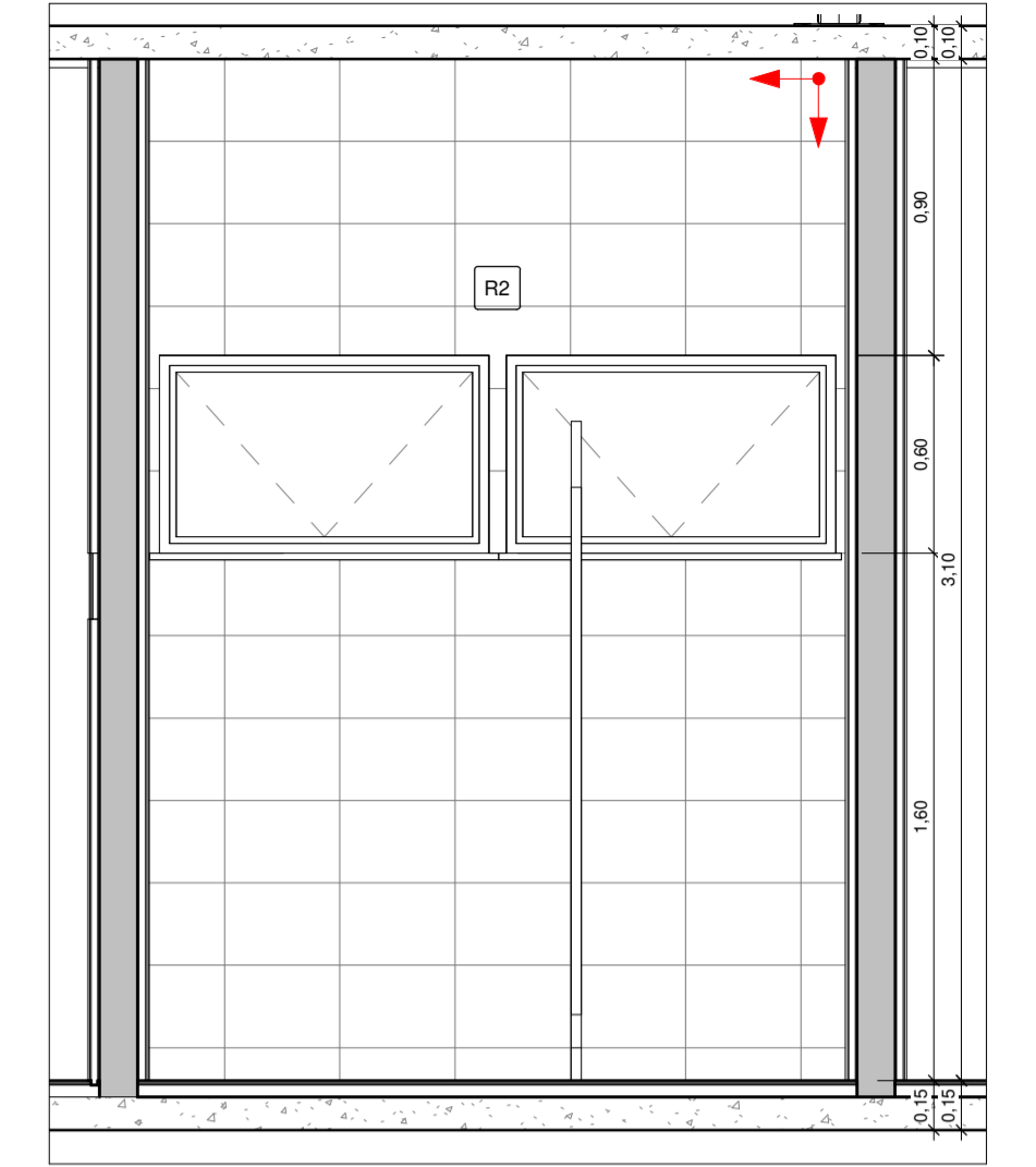
5 VEST. M. VISTA 2 1 : 25
