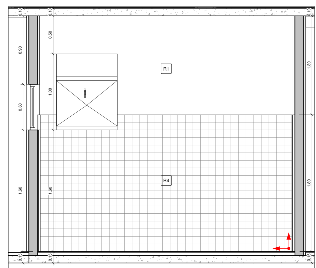
14 LAVAGEM E DESINFECÇÃO VISTA 3 1 : 25
