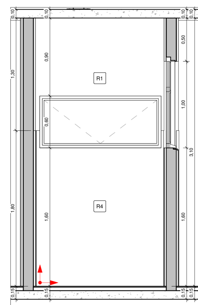
13 LAVAGEM E DESINFECÇÃO VISTA 2 1 : 25
