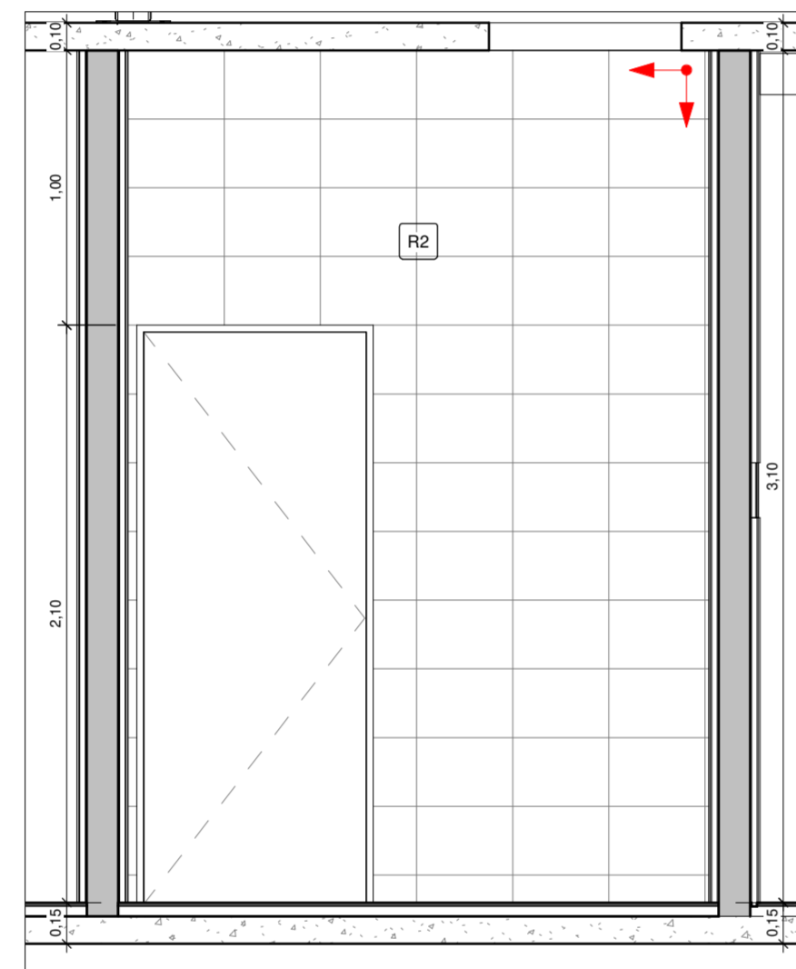
7 VEST. M. VISTA 4 1 : 25
