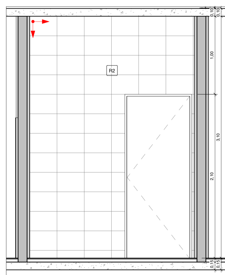
11 VEST. F. VISTA 4 1 : 25
