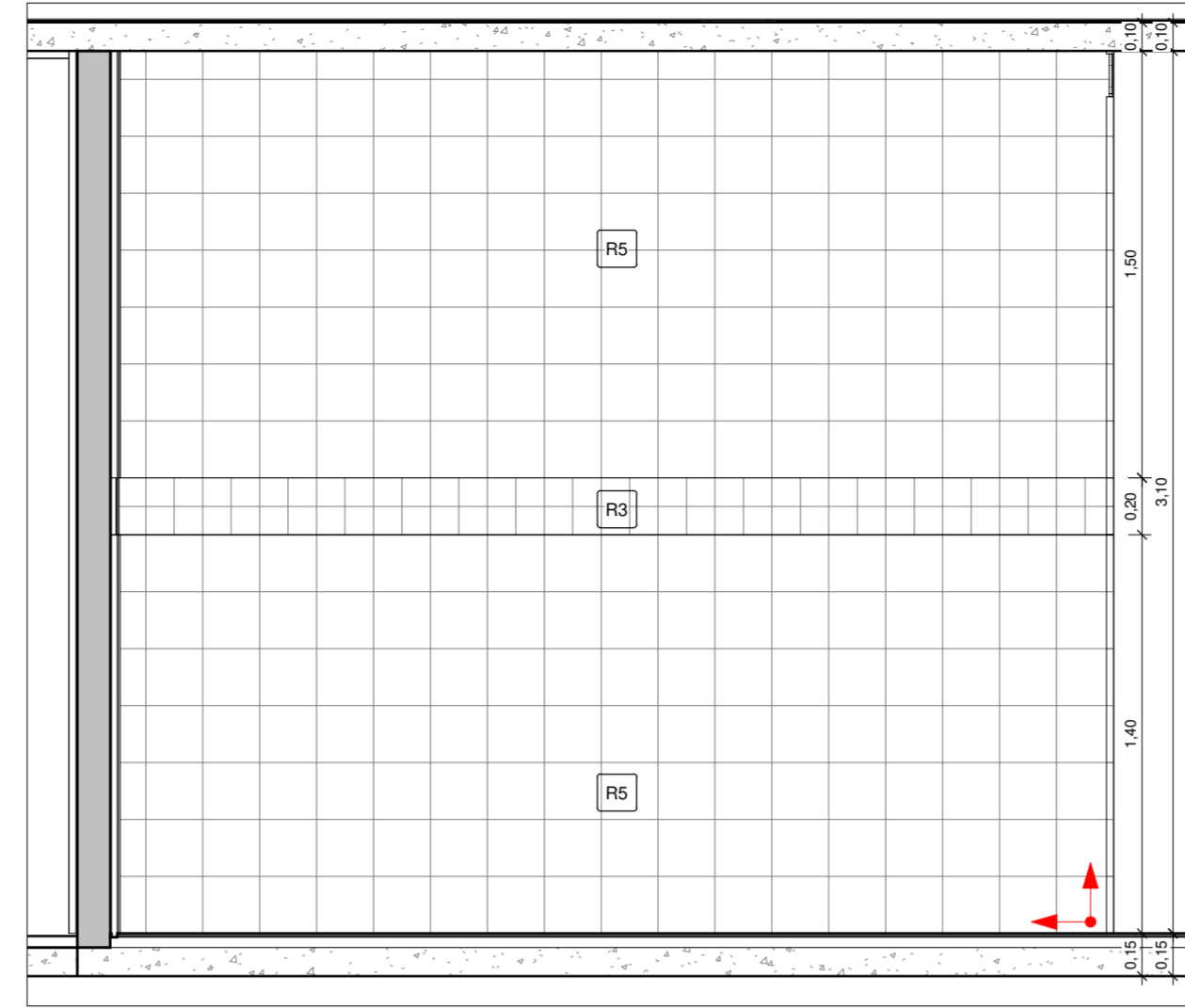
3 COPA VISTA 3 1 : 25
