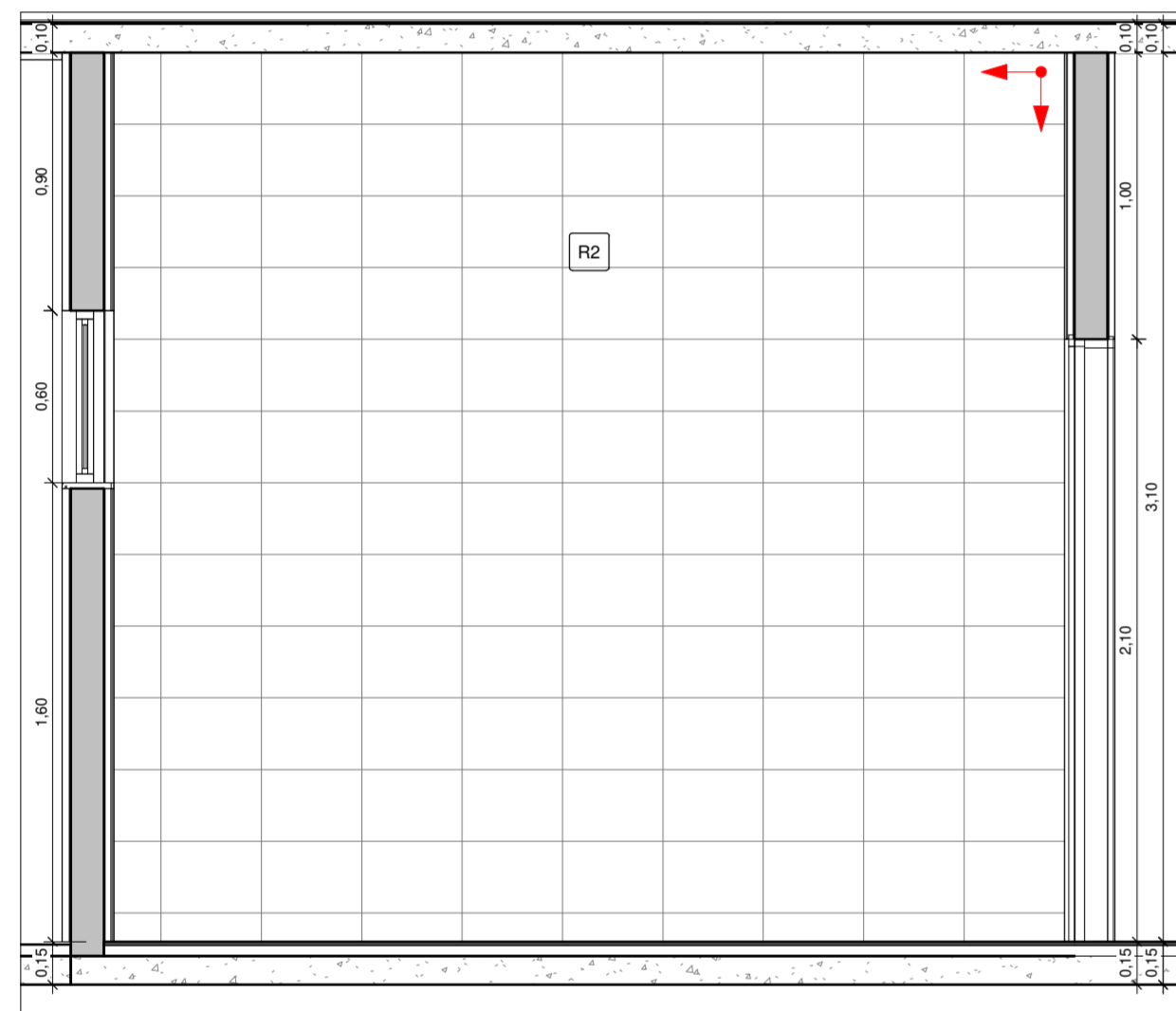
6 VEST. M. VISTA 3 1 : 25
