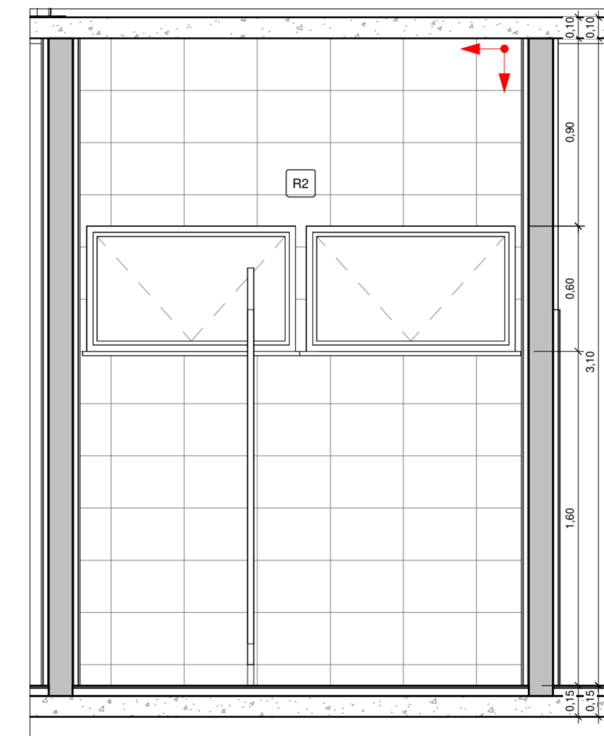
9 VEST. F. VISTA 2 1 : 25
