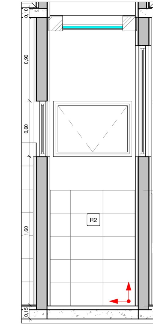
3 A.S./TANQUE VISTA 2 1 : 25
