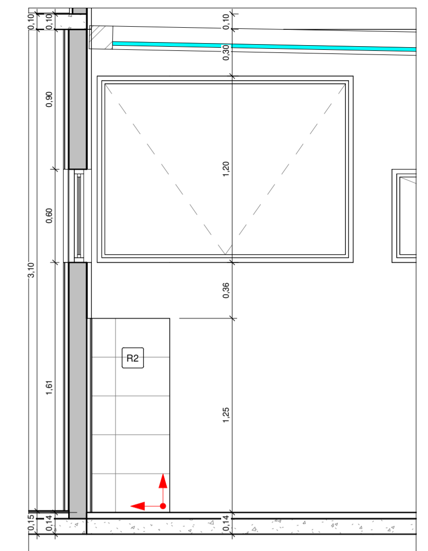
4 A.S./TANQUE VISTA 3 1 : 25
