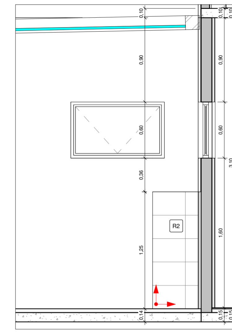
2 A.S./TANQUE VISTA 1 1 : 25
