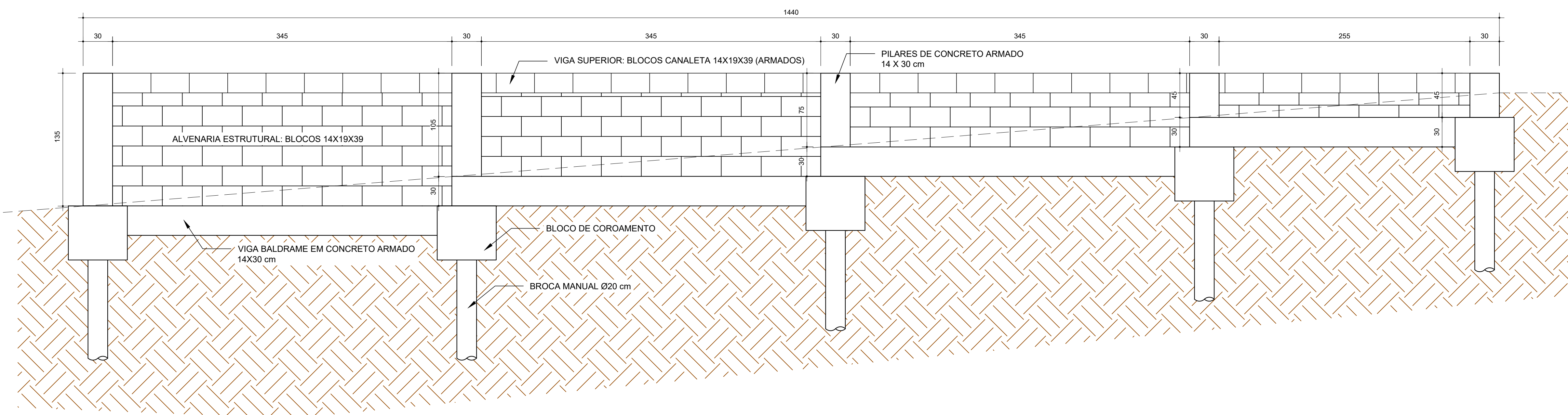
DETALHAMENTO DO MURO ESCALA 1:25
