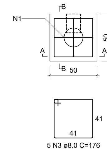
B2 1xC20 PLANTA ESC 1:25
