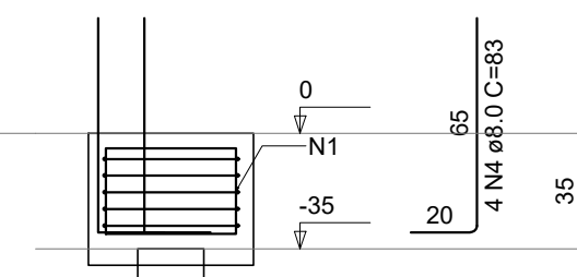
CORTE B-B ESC 1:25
