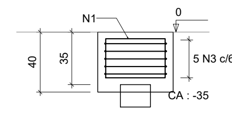
CORTE ESC 1:25
