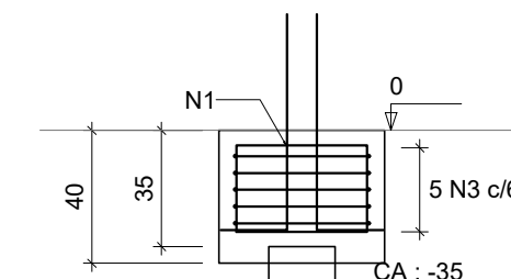
CORTE A-A ESC 1:25
