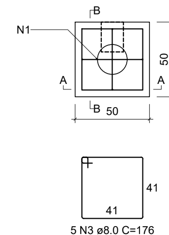
B11 1xC20 PLANTA ESC 1:25
