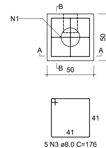
B1 1xC20 PLANTA ESC 1:25
