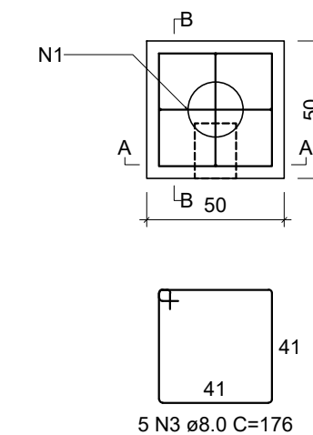
B3 1xC20 PLANTA ESC 1:25
