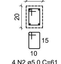
DETALHE DO PILAR ESC 1:20
