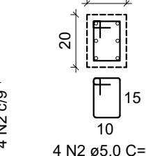
DETALHE DO PILAR ESC 1:20
