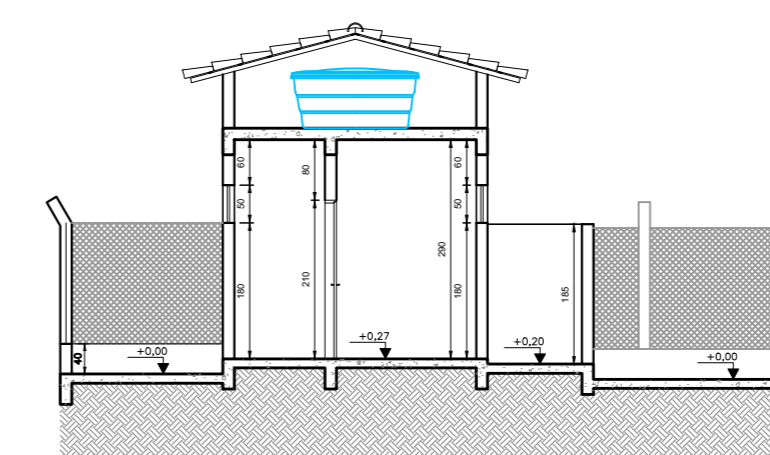
CORTE BB Escala: 1:100
