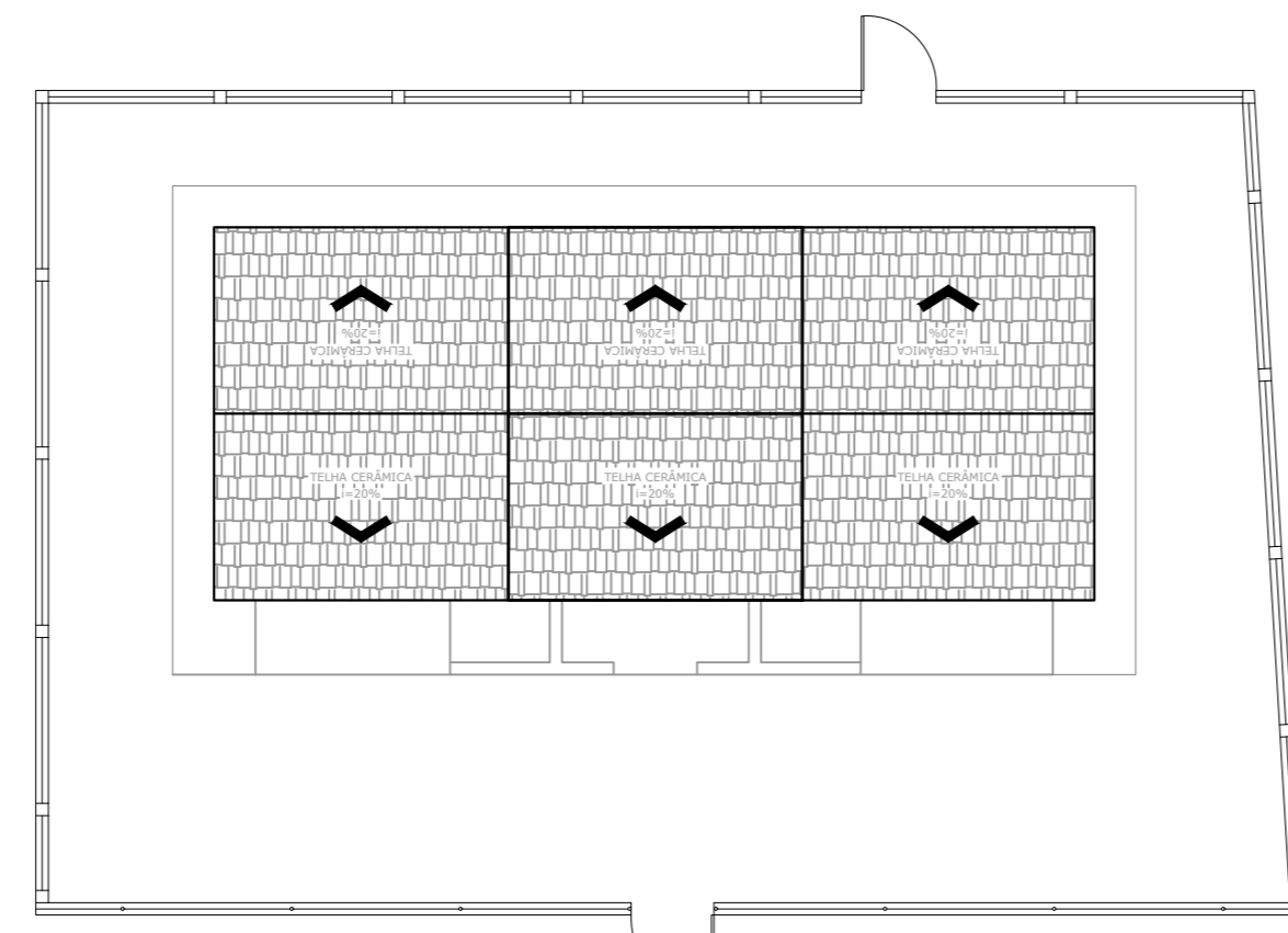
PLANTA COBERTURA Escala: 1:100
