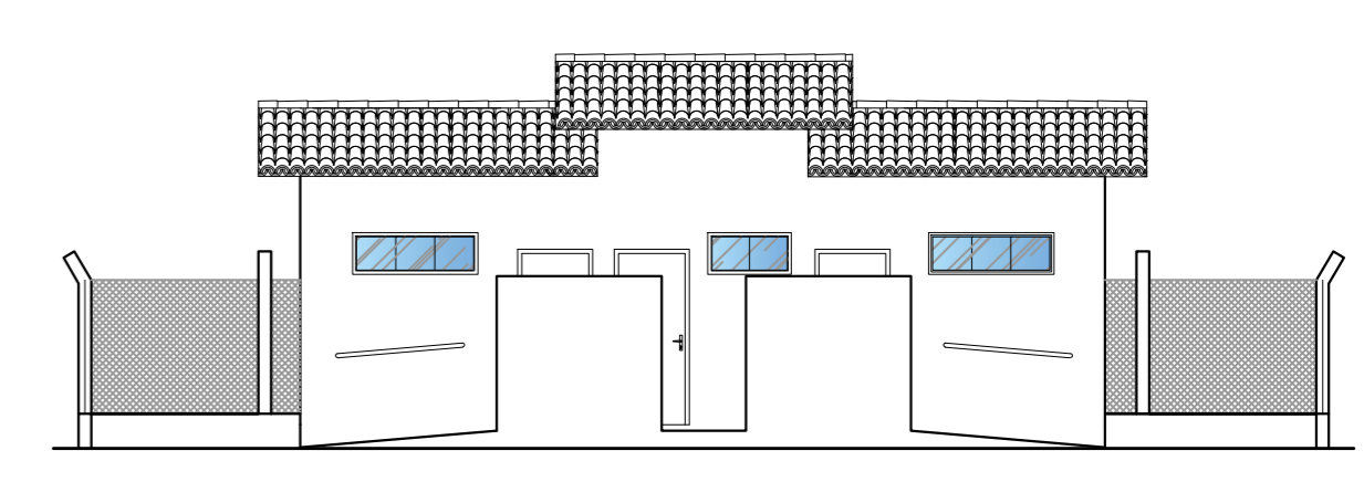
FACHADA Escala: 1:100
