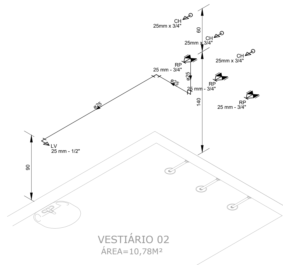
DETALHE HID-3 ESCALA 1:25
