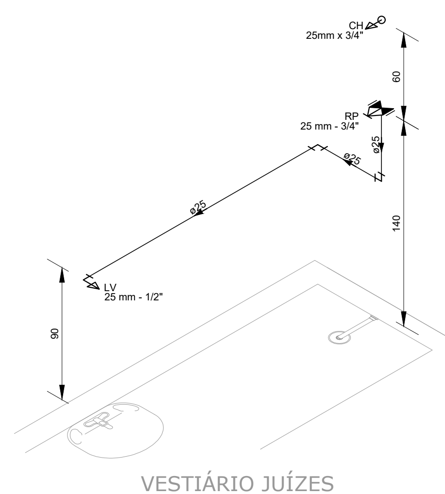
DETALHE HID-2 ESCALA 1:25
