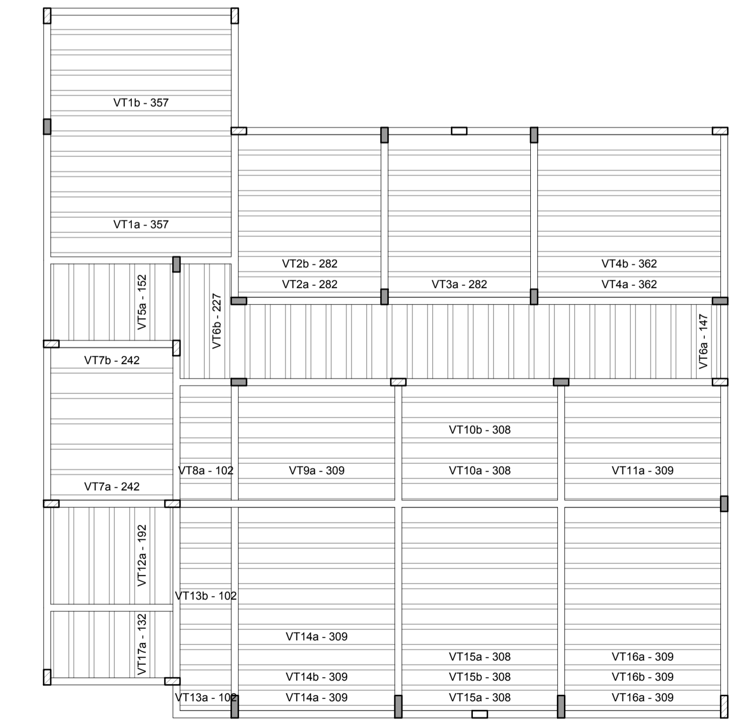
Planta de vigotas pré-moldadas escala 1:75
