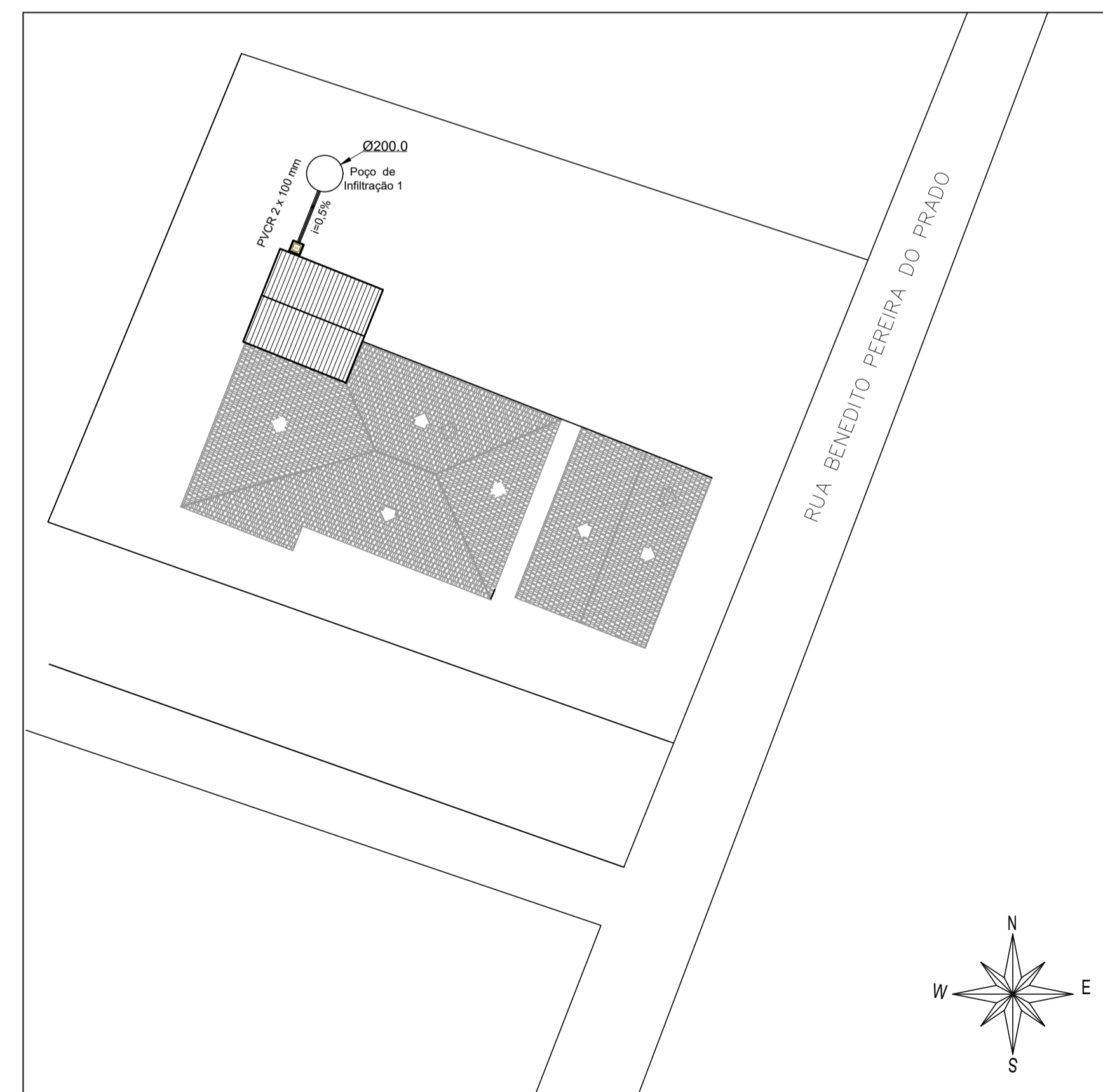
PLANTA DE LOCALIZAÇÃO DAS CAIXAS Escala 1:350
