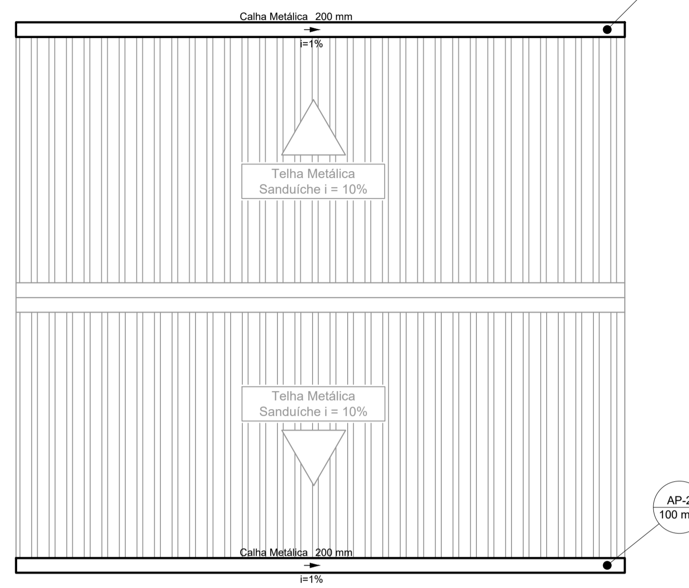
PLANTA COBERTURA Escala 1:50
