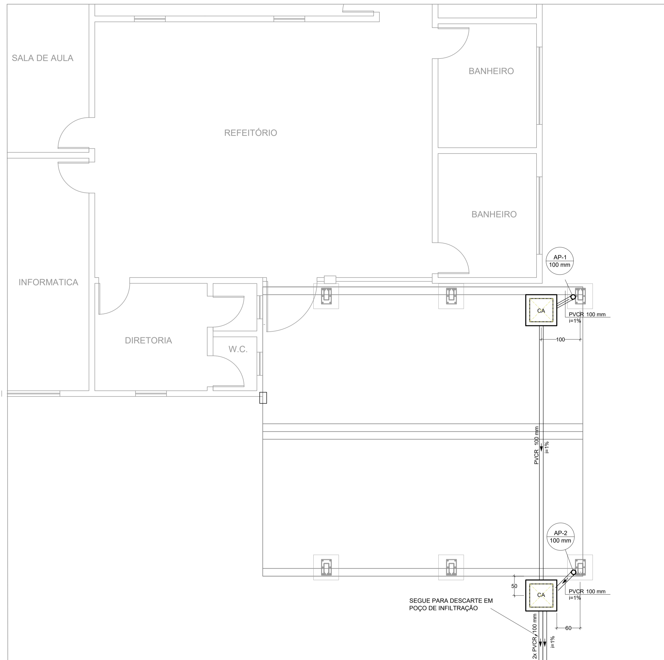
PLANTA TÉRREO Escala 1:50
