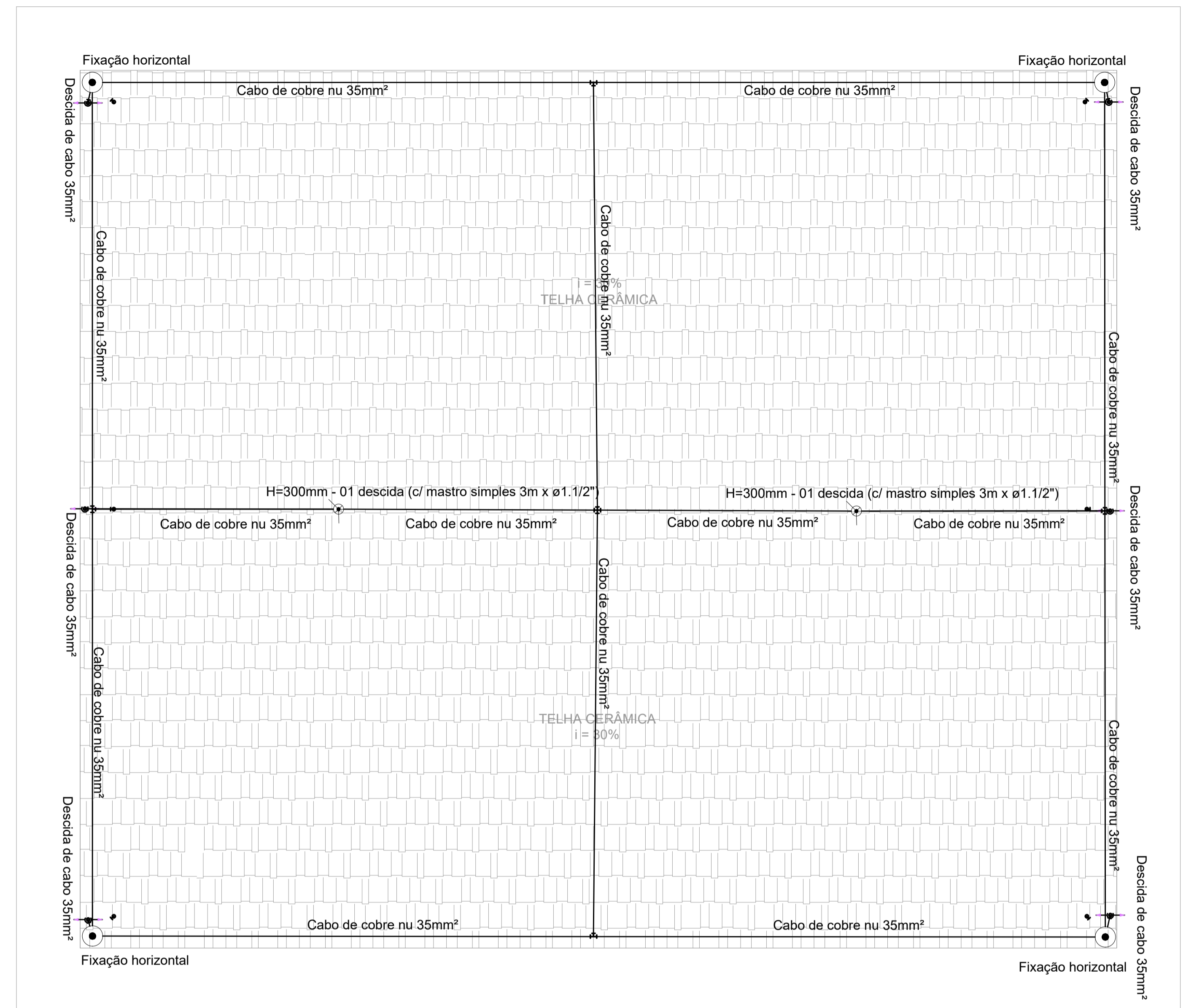
PLANTA BAIXA COBERTURA 1:50
