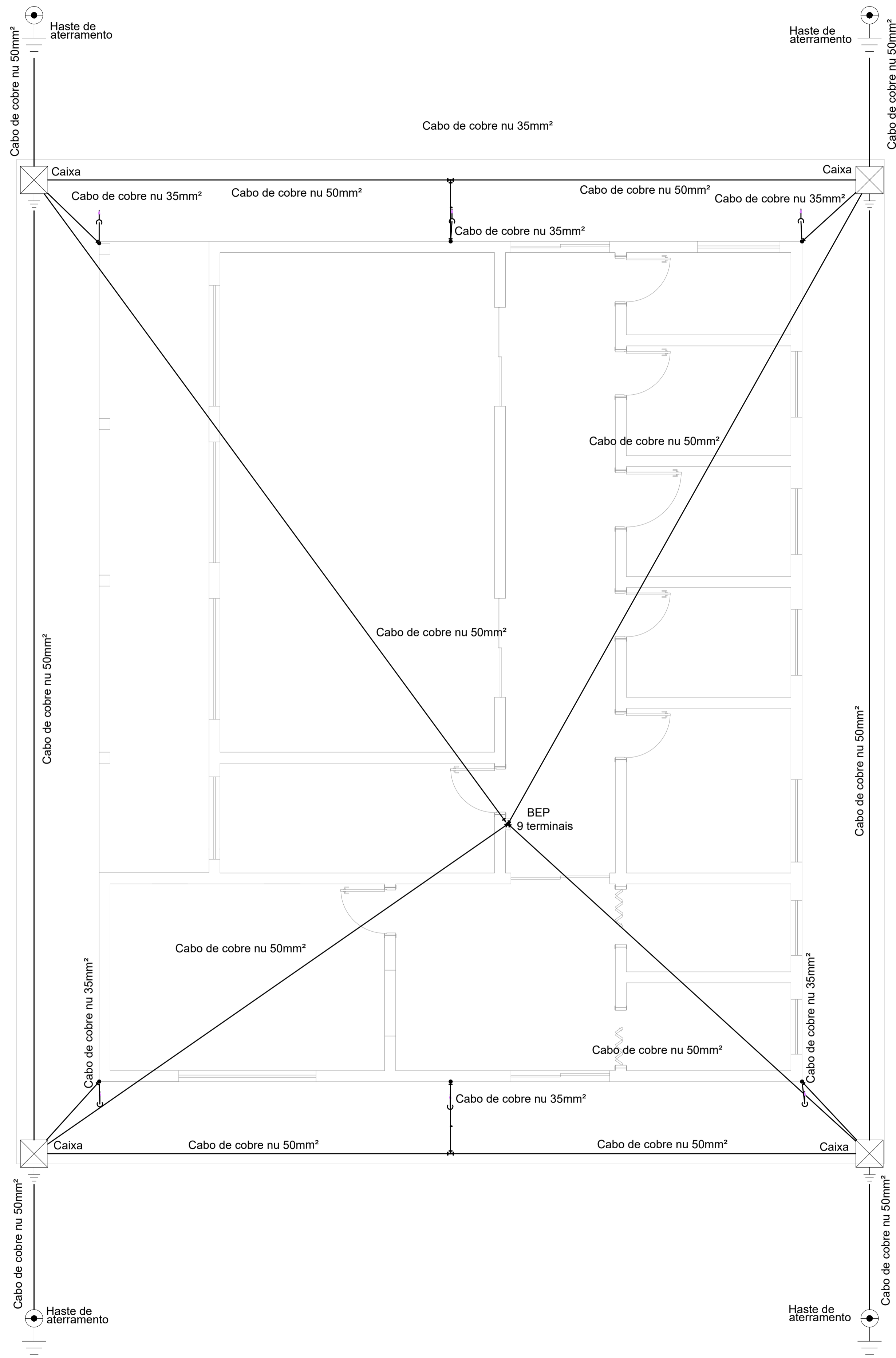
PLANTA BAIXA PAVIMENTO 1:50
