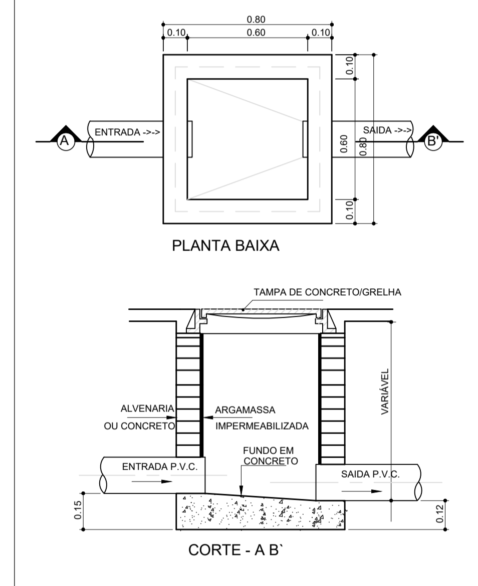
DETALHE DAS CAIXAS DE PASSAGEM SEM ESCALA
