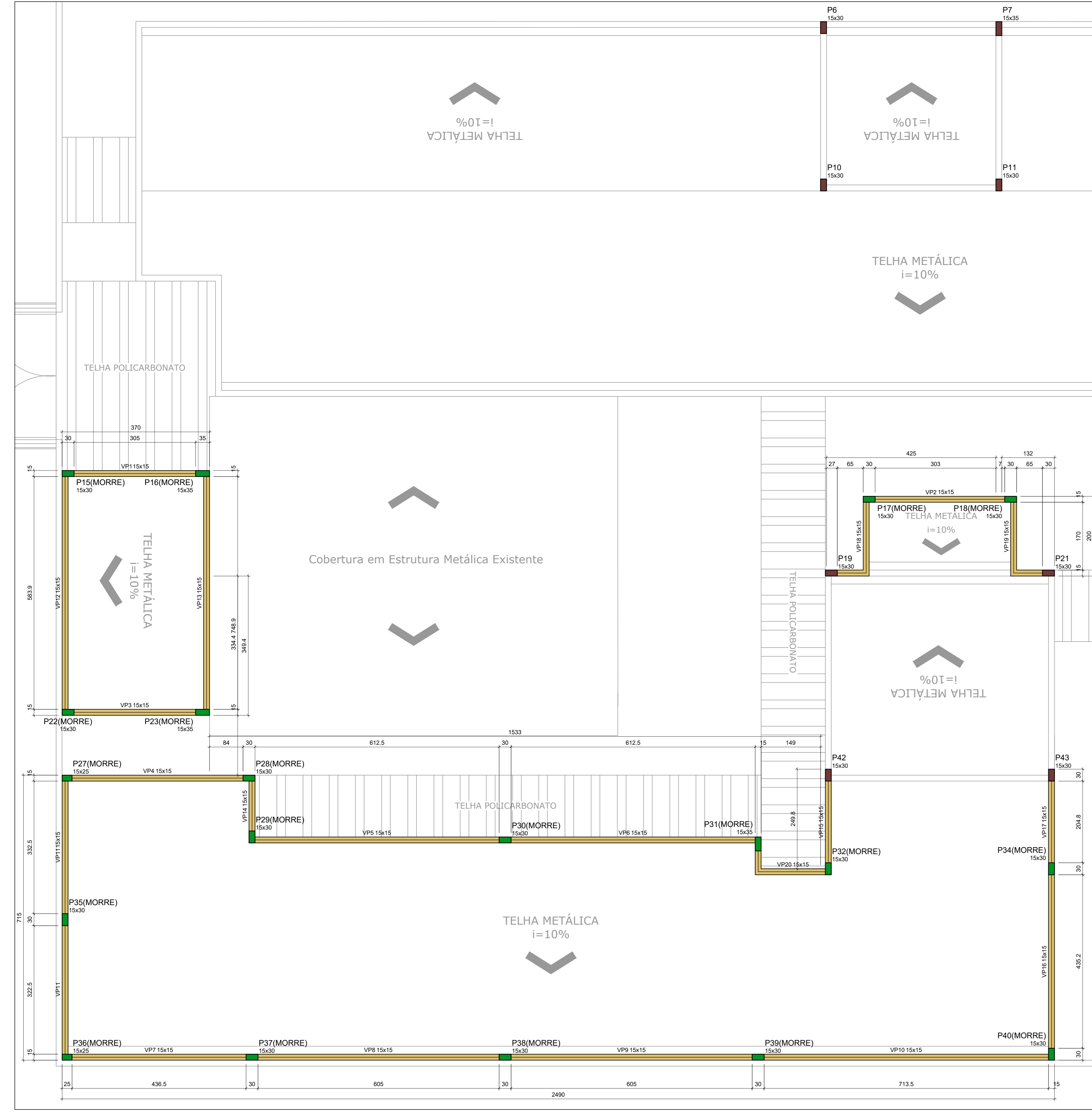
Forma do pavimento Platibanda (Nível 4.80) escala 1:50
