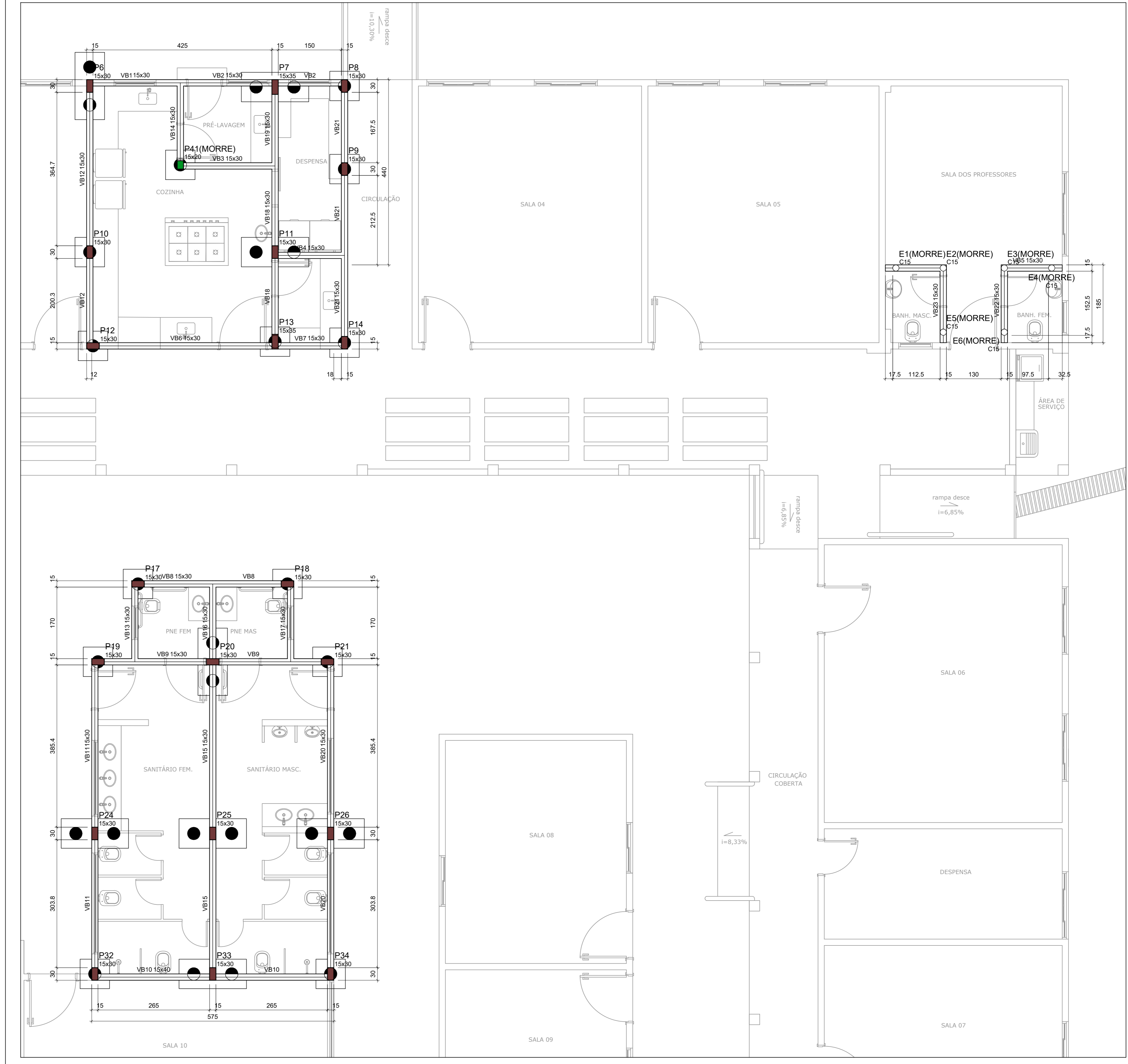
Forma nível da Fundação (Nível 0.00) escala 1:50
