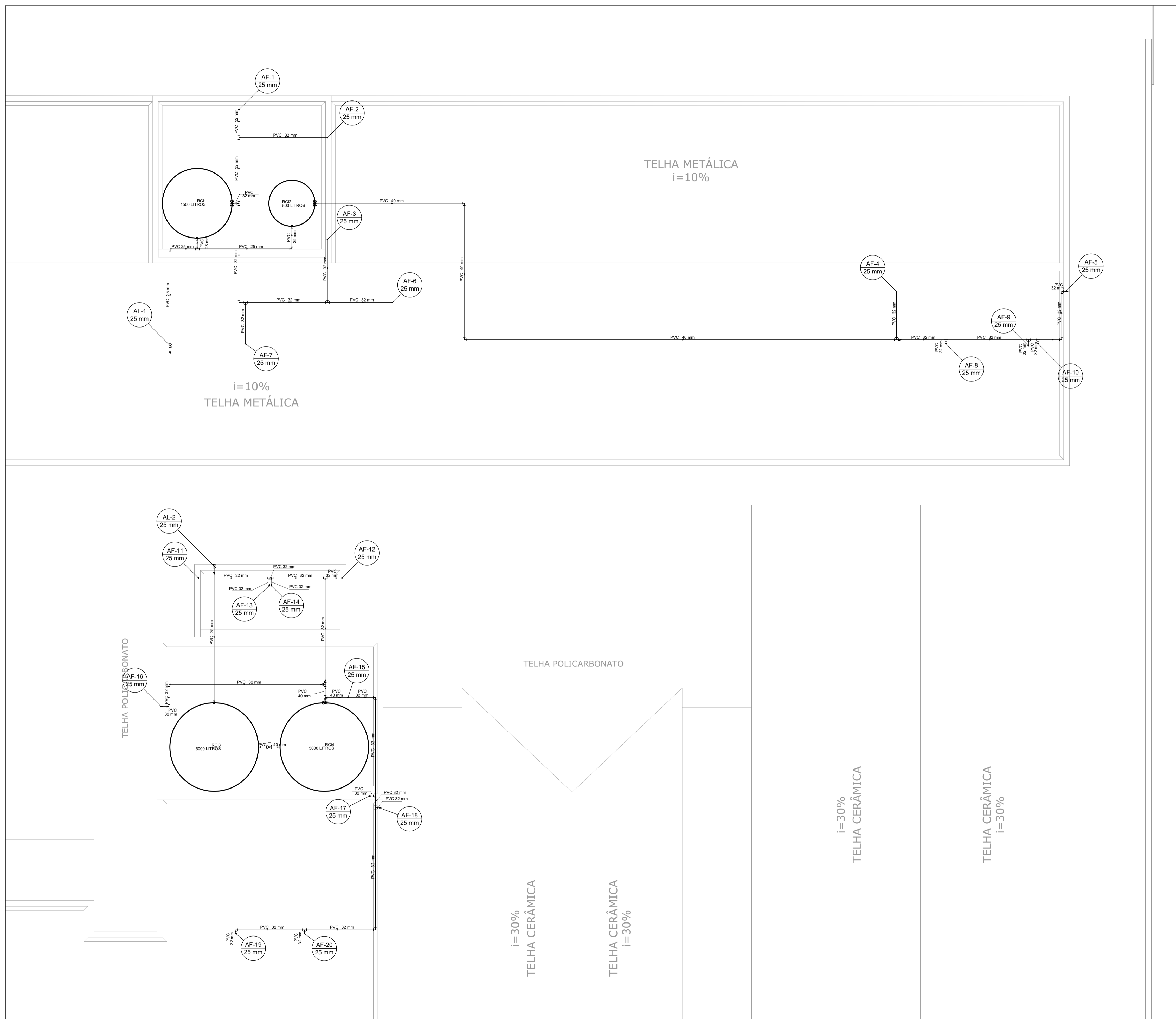
PLANTA BAIXA INSTALAÇÕES HIDRÁULICAS COBERTURA PARTE 1-1 ESCALA 1:50
