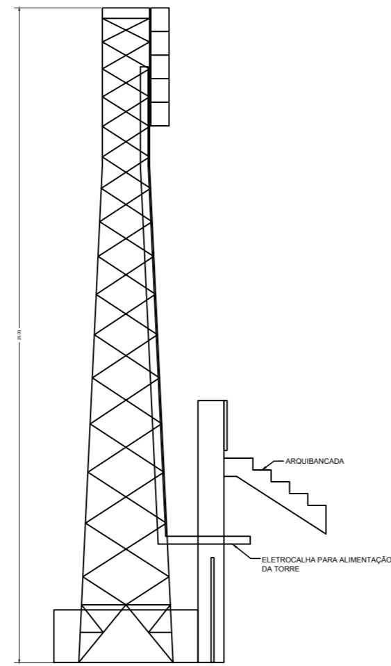
CORTE BB ESCALA 1:200
