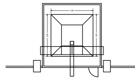
PLANTA BAIXA TORRE 02 ESCALA 1:200
