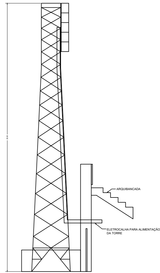
CORTE AA ESCALA 1:200
