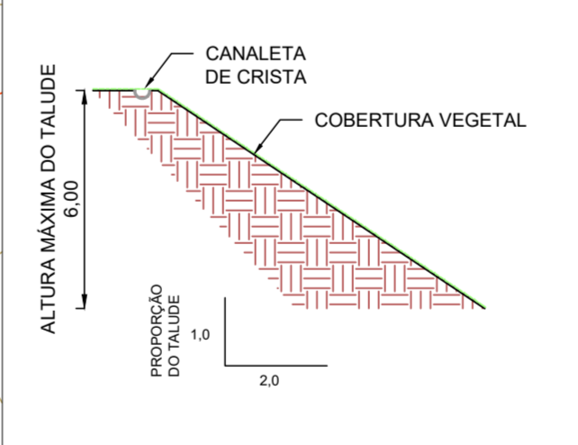
DETALHE DOS TALUDES DE CORTE SEM ESCALA
