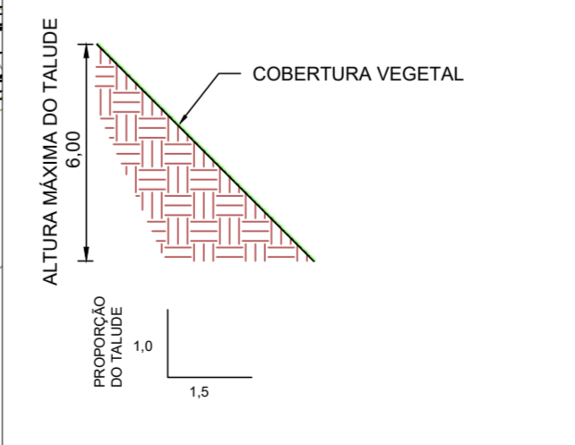
DETALHE DOS TALUDES DE CORTE SEM ESCALA
