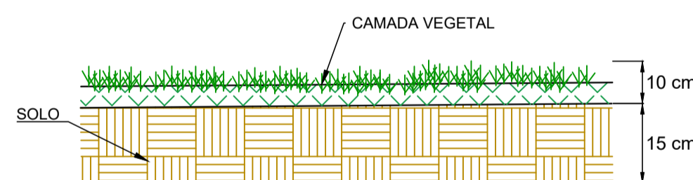
DETALHE 2 - REMOÇÃO DE CAMADA VEGETAL SEM ESCALA
