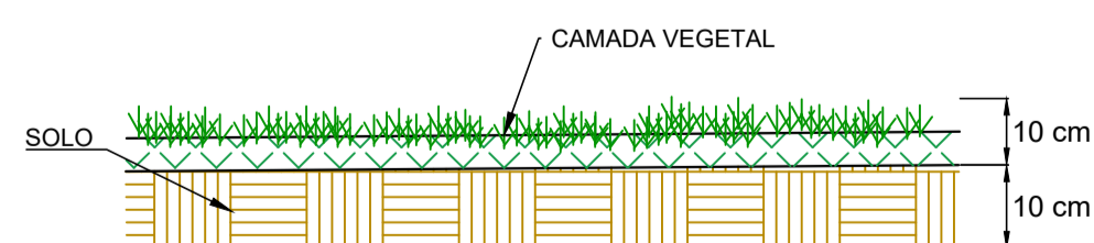
DETALHE 3 - REMOÇÃO DE CAMADA VEGETAL ACESSO SEM ESCALA
