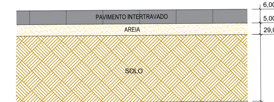
DETALHE 03 - DEMOLIÇÃO PAVIMENTO SEXTAVADO LEITO CARROÇAVEL - SEM ESCALA
