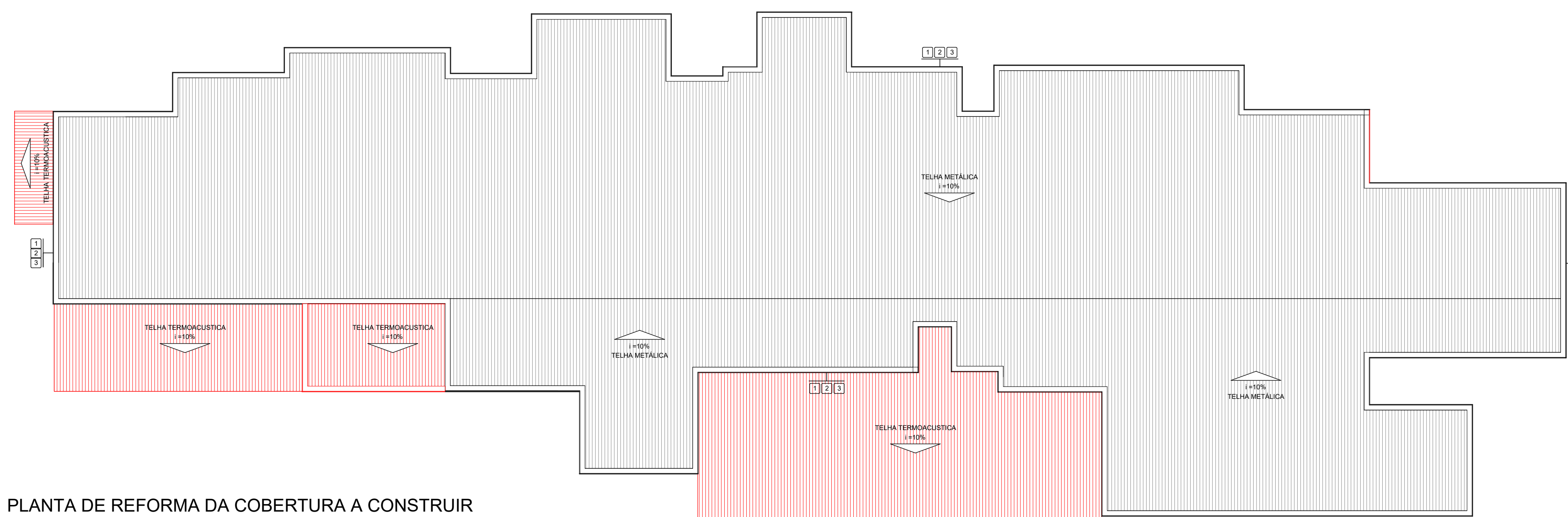
4 PLANTA DE REFORMA DA COBERTURA A CONSTRUIR 1 : 100
