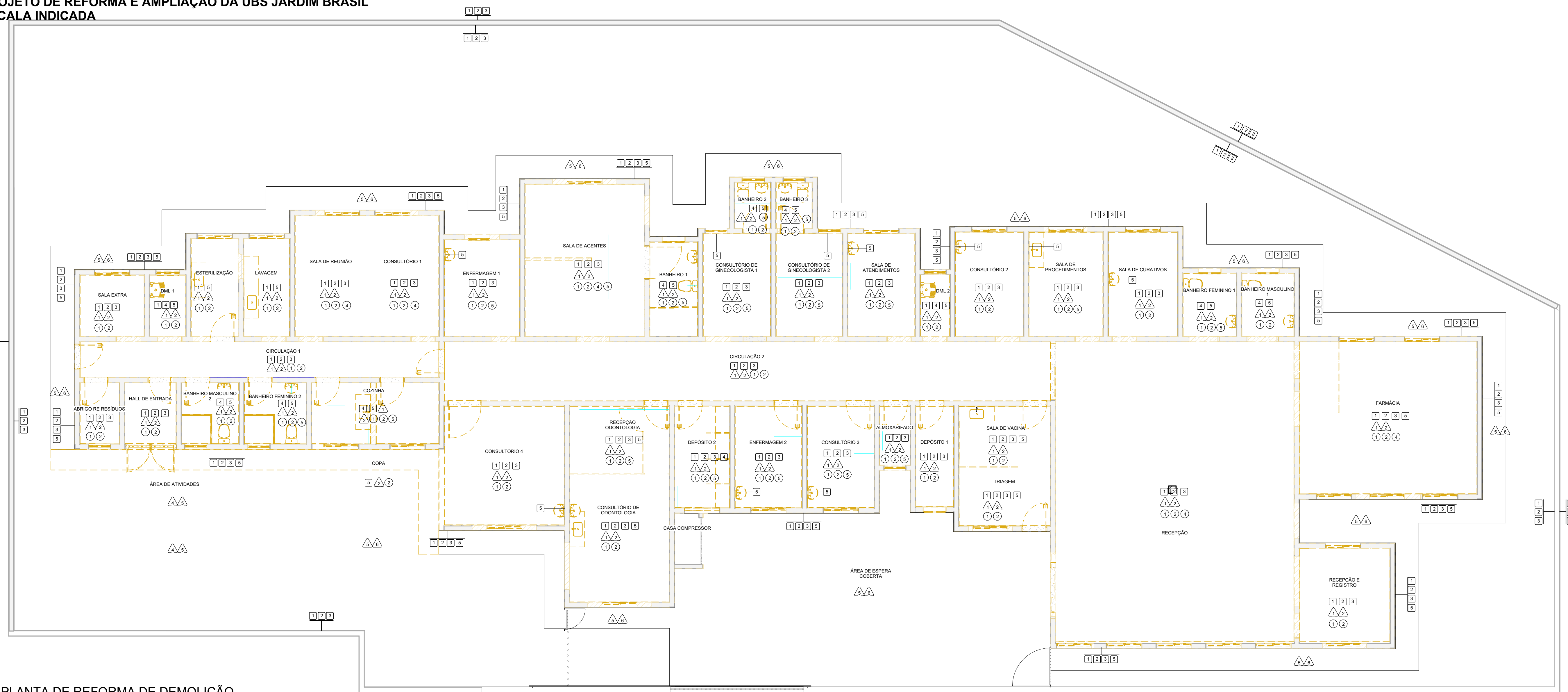
1 PLANTA DE REFORMA DE DEMOLIÇÃO 1 : 75
