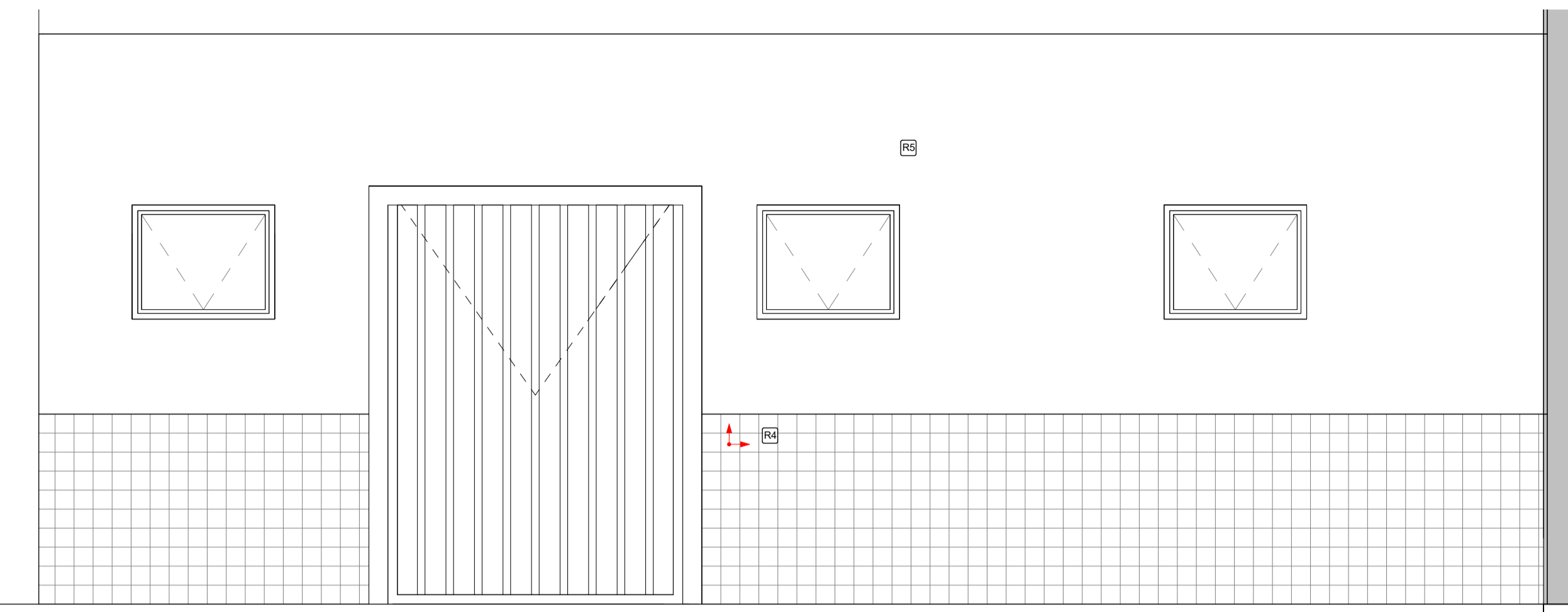
1 Fachada Vista 01 1 : 25
