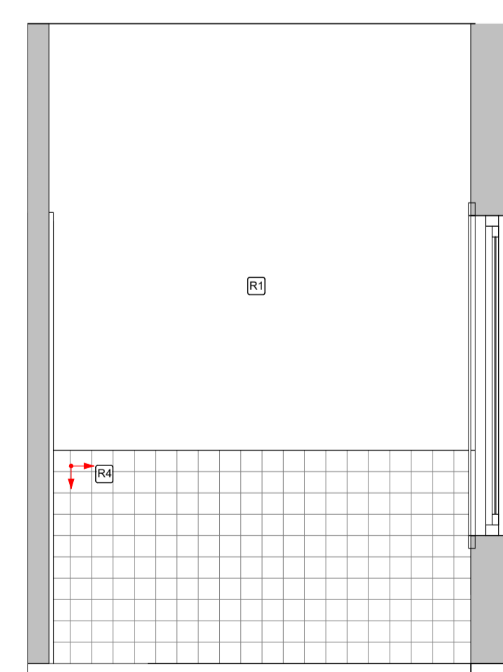
10 Triagem Vista 02 1 : 25
