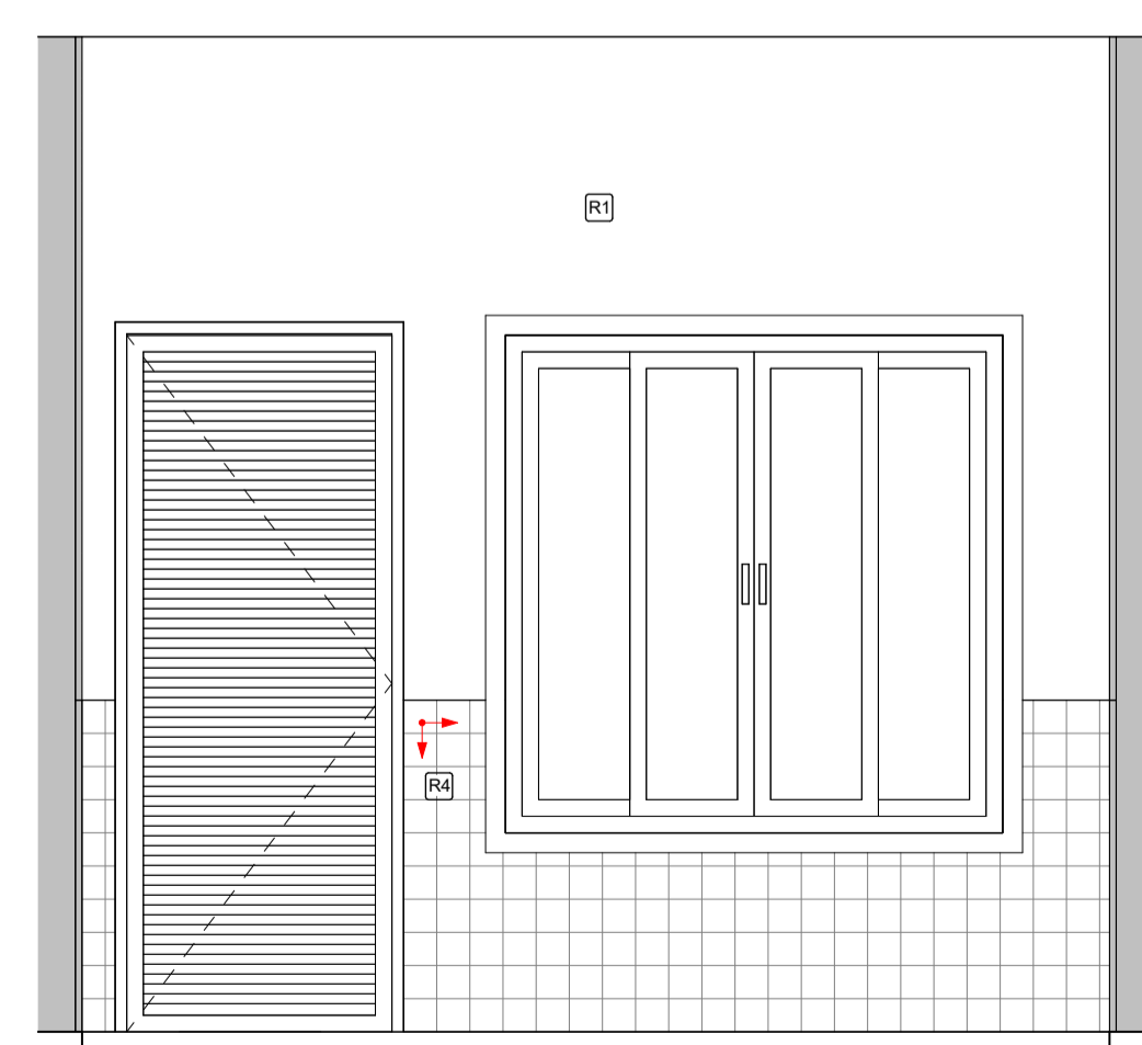
11 Triagem Vista 03 1 : 25
