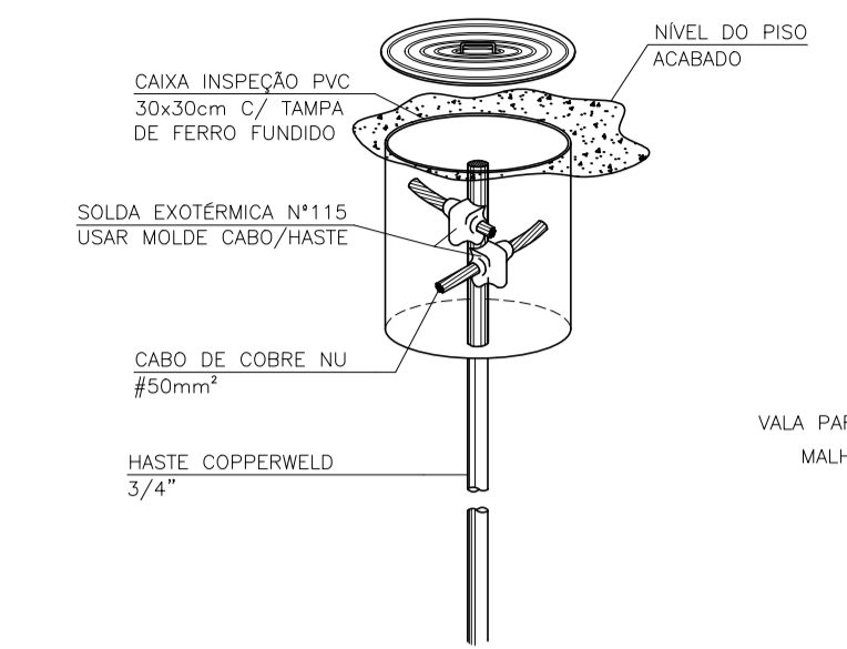
CAIXA DE INSPEÇÃO 30X30 CM
