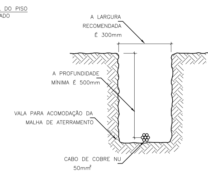
VALA DE ATERRAMENTO
