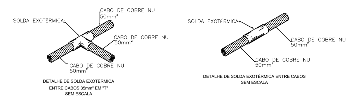
SOLDAS EXOTÉRMICAS
