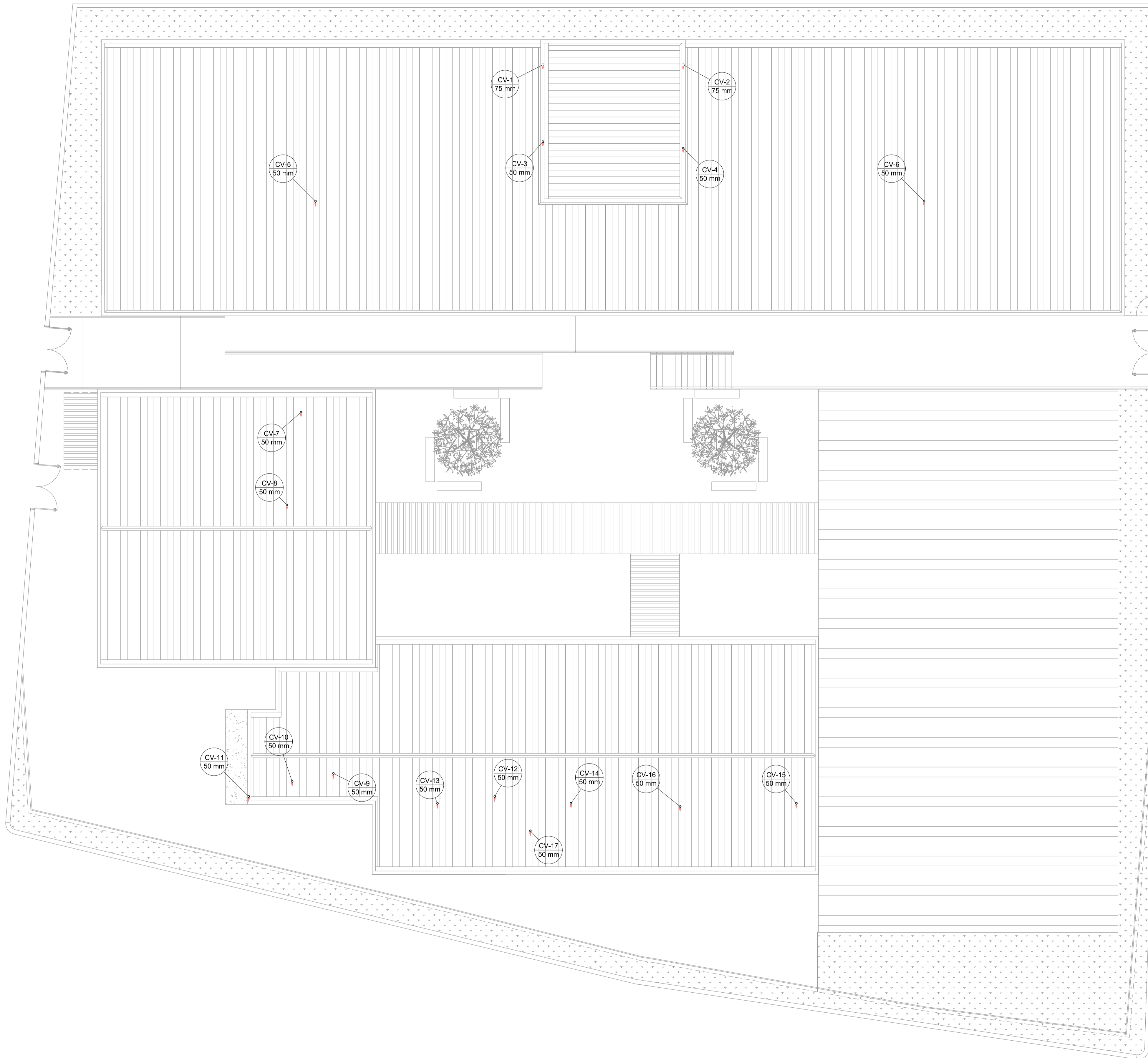
PLANTA BAIXA COBERTURA Esc 1:100
