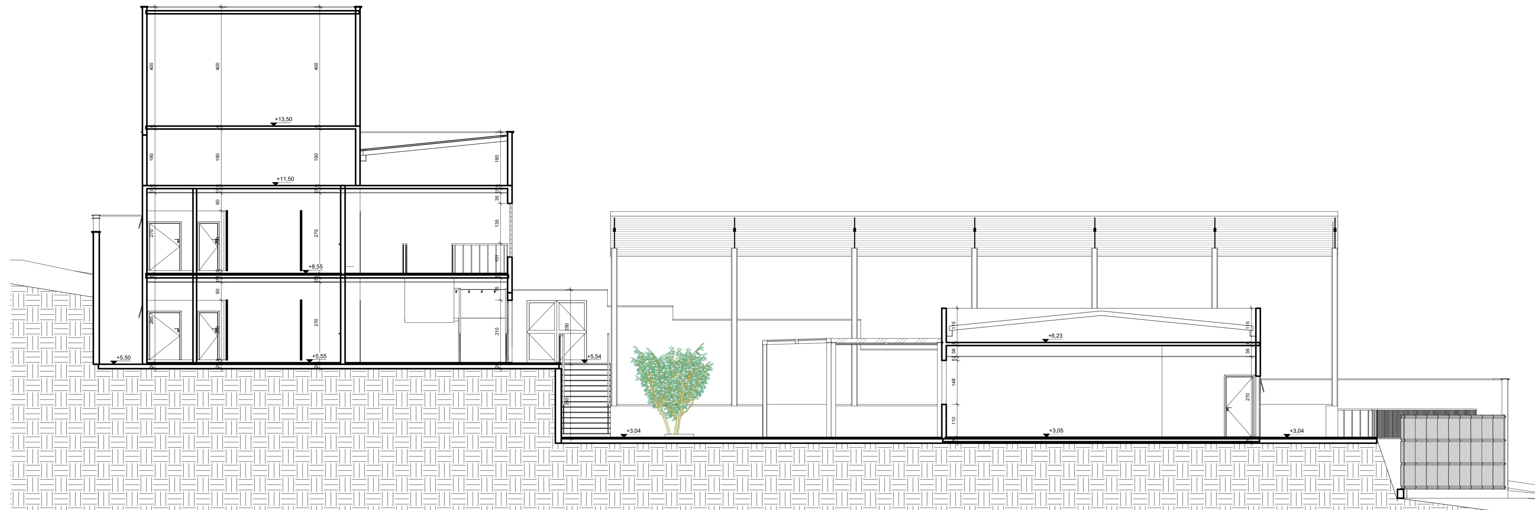
1 EE 1:75
