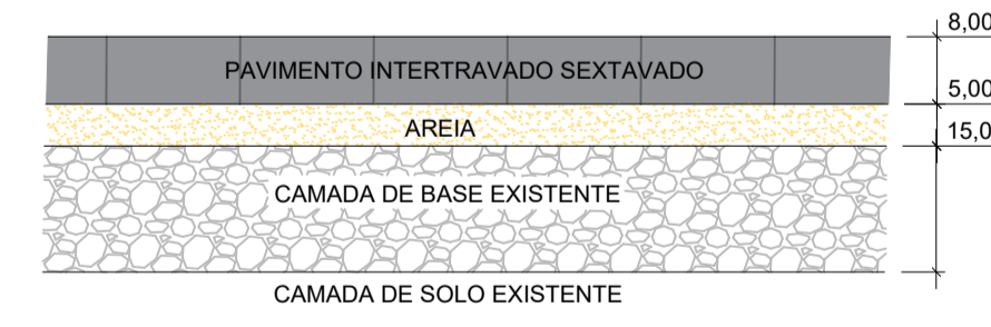
DETALHE 01 - DEMOLIÇÃO DE PAVIMENTO SEXTAVADO SEM ESCALA
