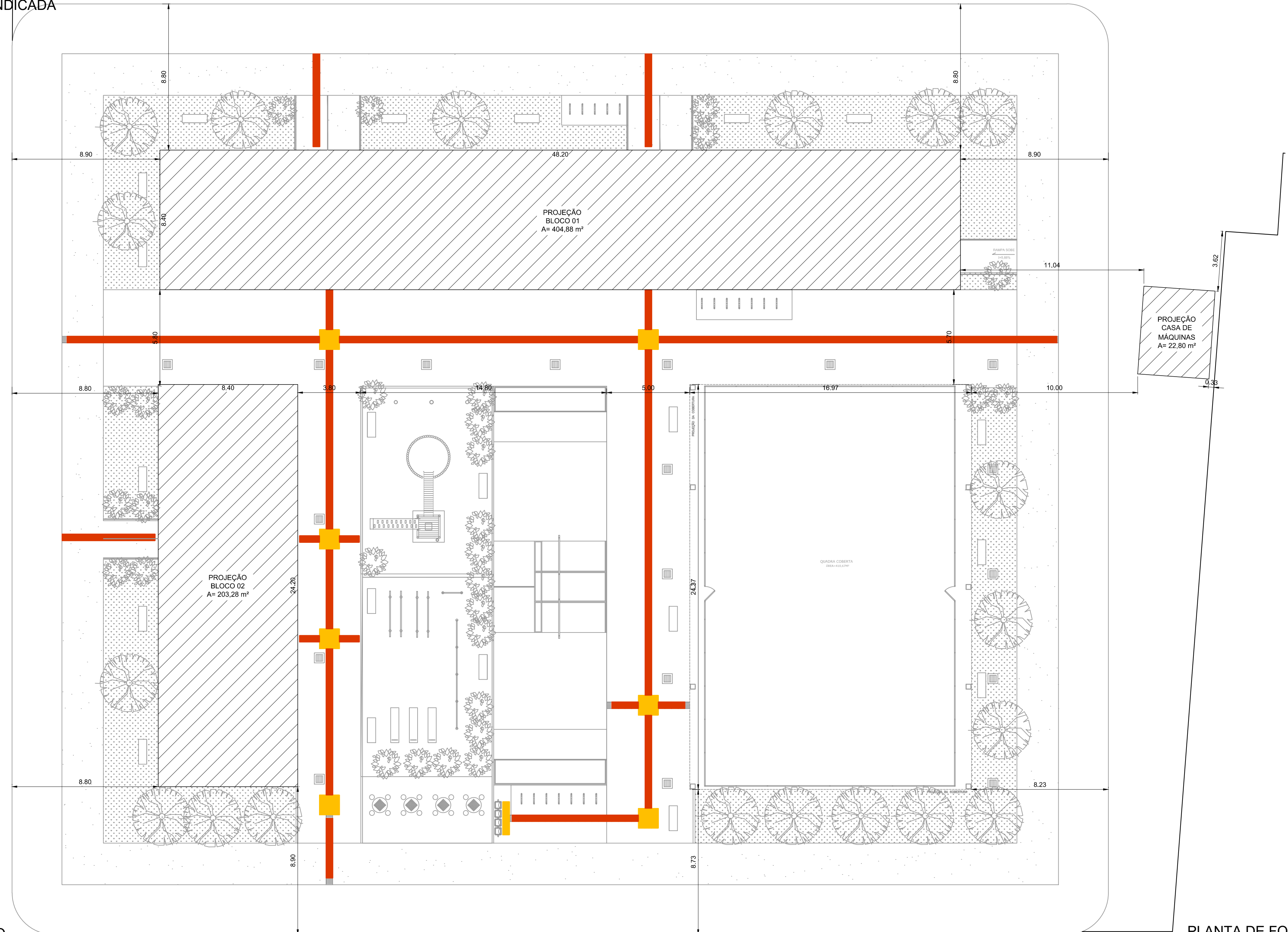
PLANTA DE FORRO Escala: 1:150
