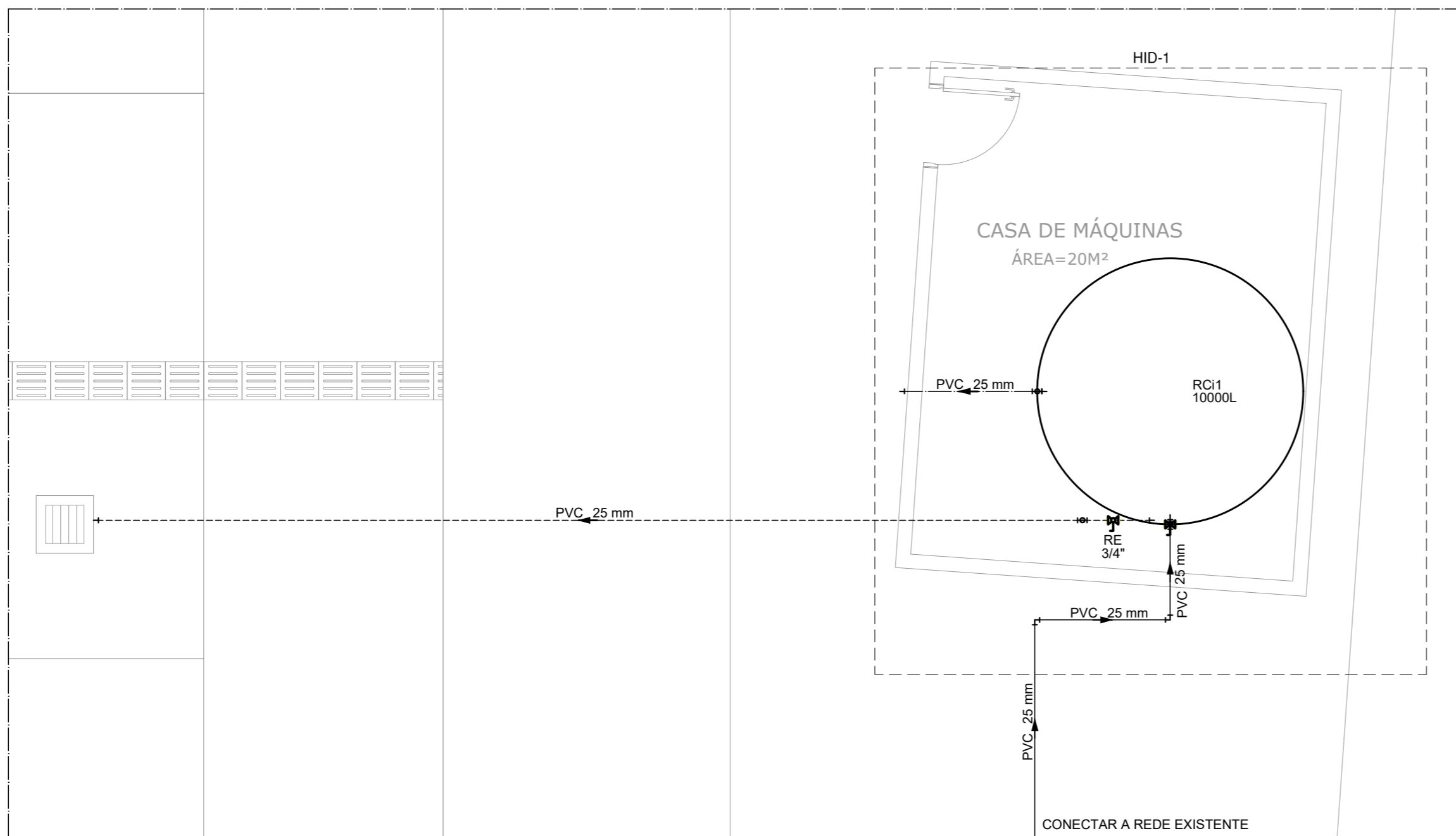
PLANTA BAIXA Escala 1:50
