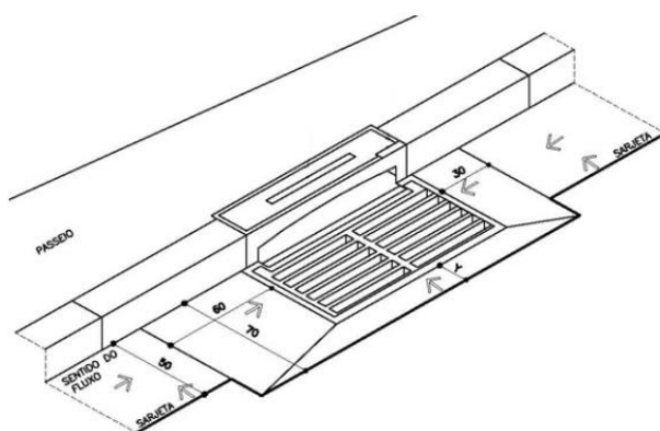
Figura 10-2 – Depressão de bocas de lobo em greide contínuo
