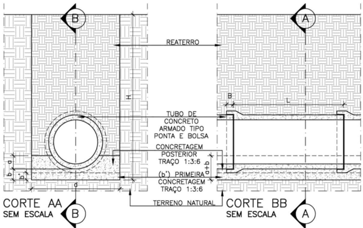
Figura 8-1 – Rede tubular de concreto
