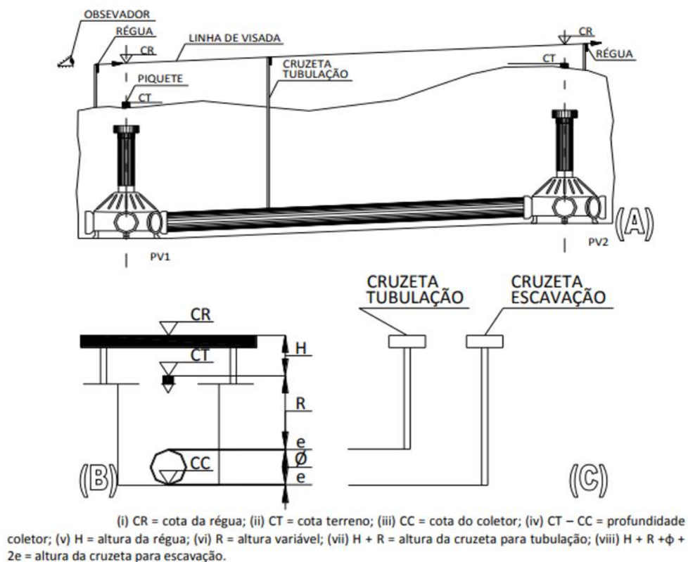
Figura 5-1 - Indicações de apoio para os cálculos
