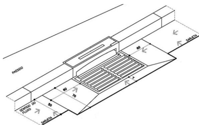
Figura 10-1 – Depressão de boca de lobo em ponto baixo
