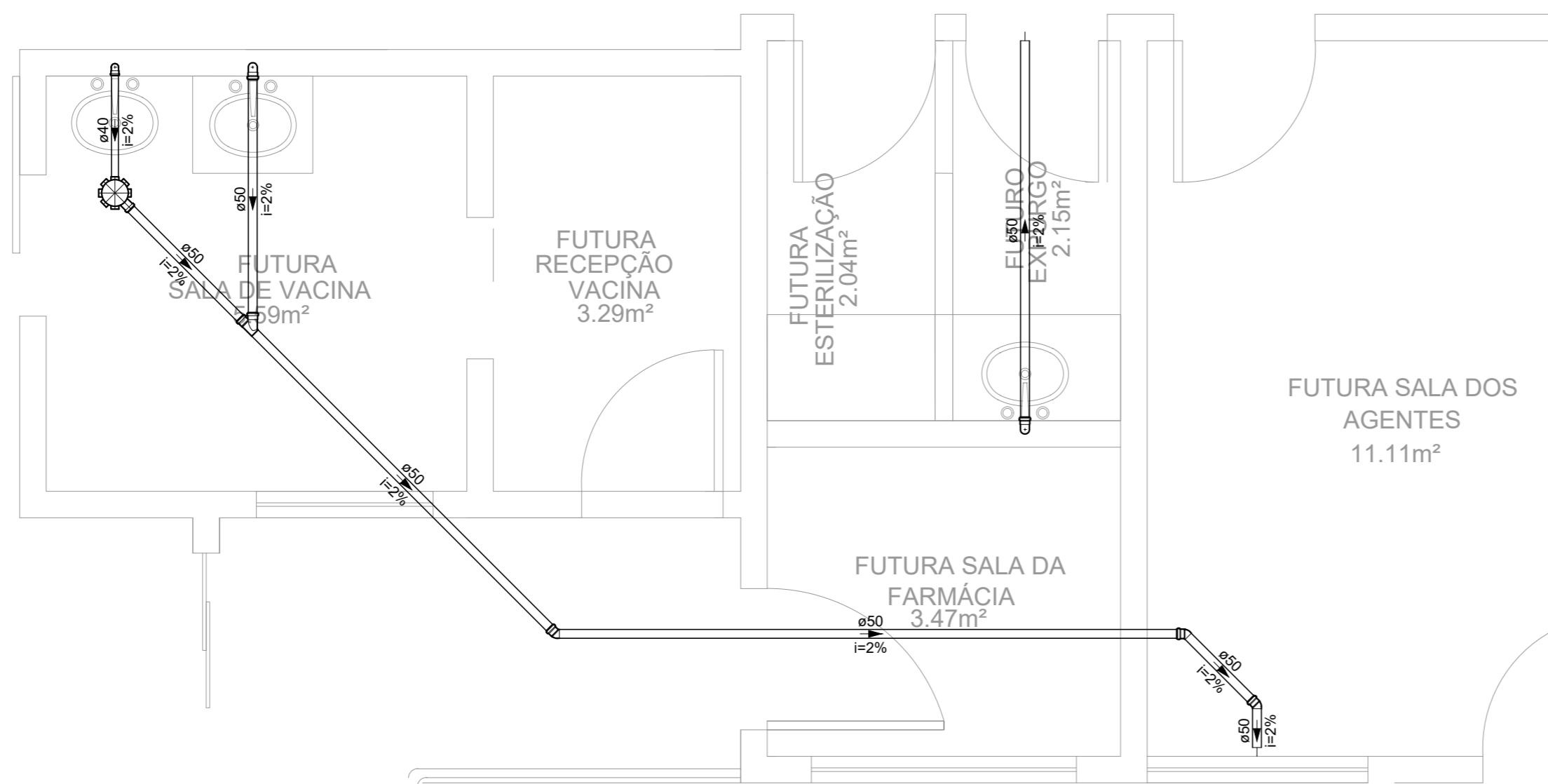
Detalhe S2 Escala 1:30
