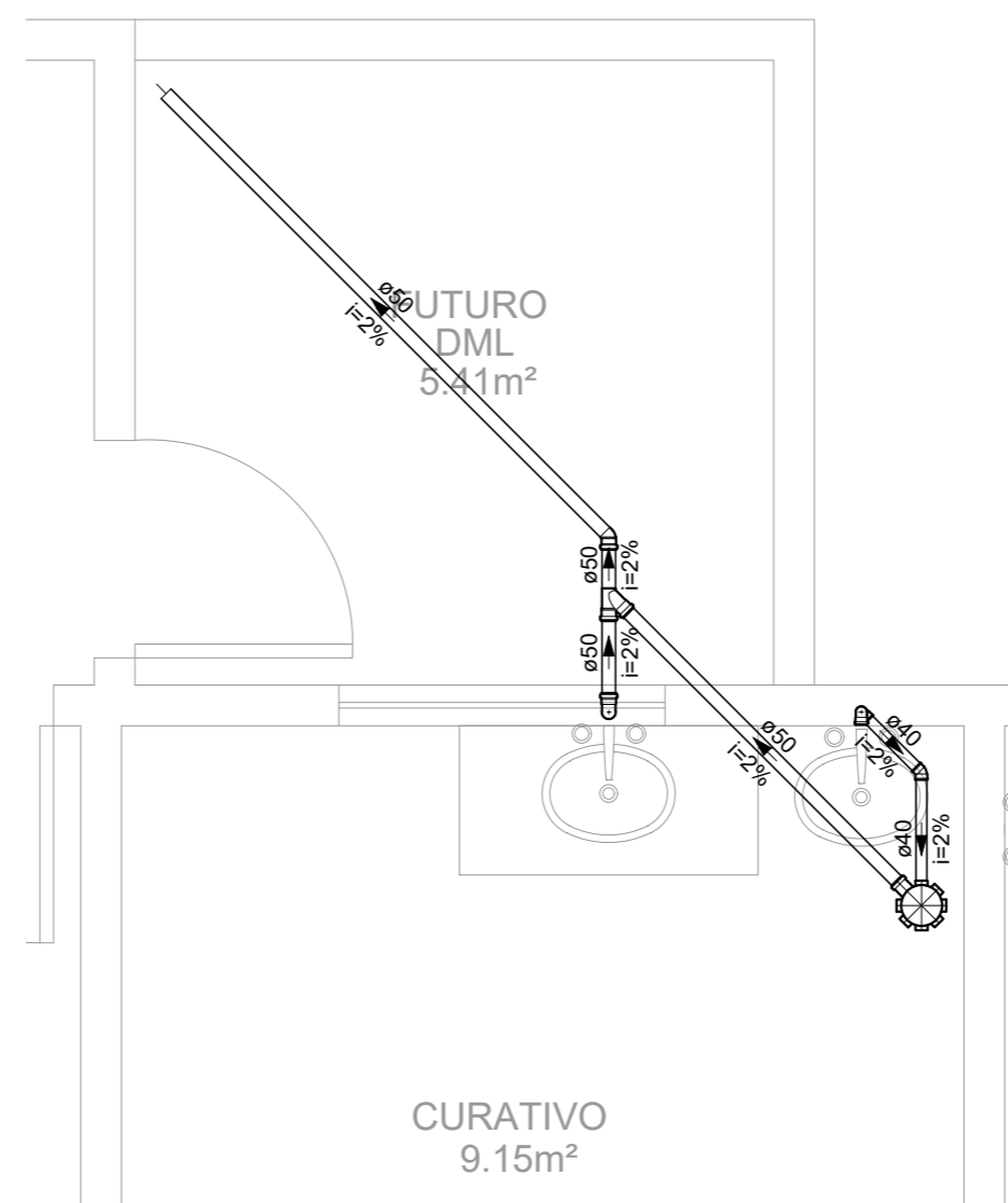
Detalhe S1 Escala 1:30
