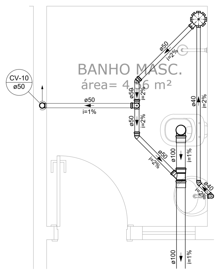
Detalhe SAN-10 Escala 1:25
