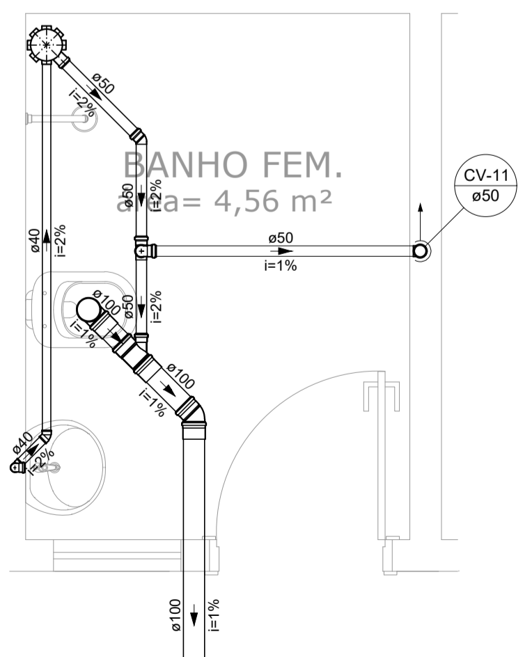
Detalhe SAN-11 Escala 1:25
