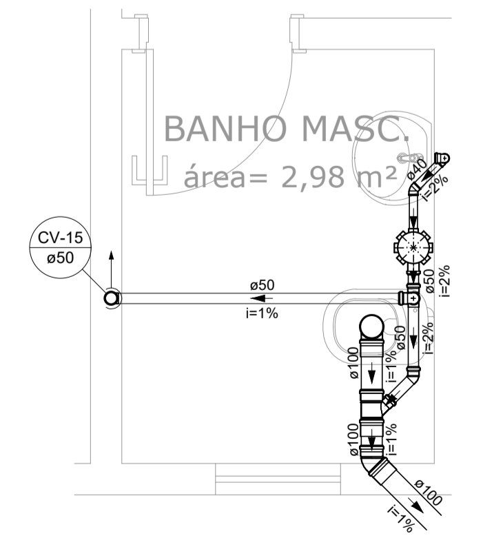
Detalhe SAN-12 Escala 1:25
