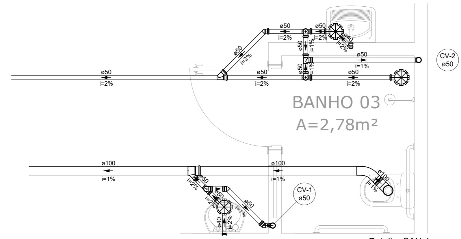
Detalhe SAN-1 Escala 1:25
