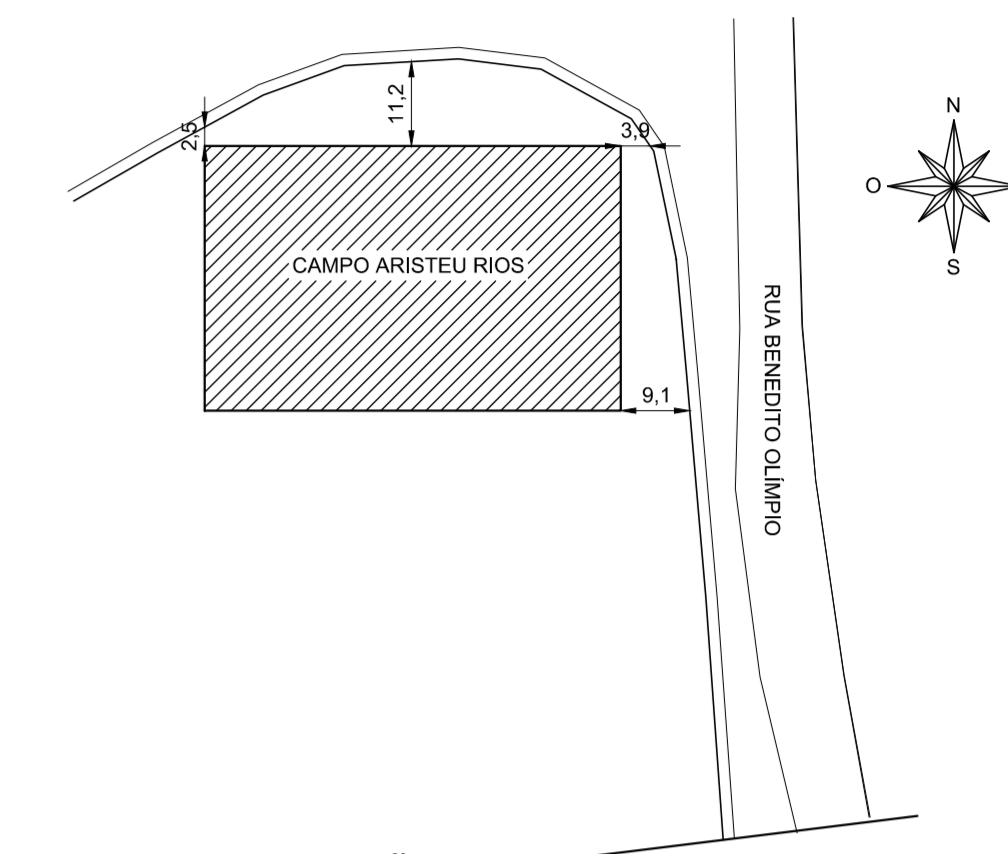
IMPLANTAÇÃO Escala: 1:1000
