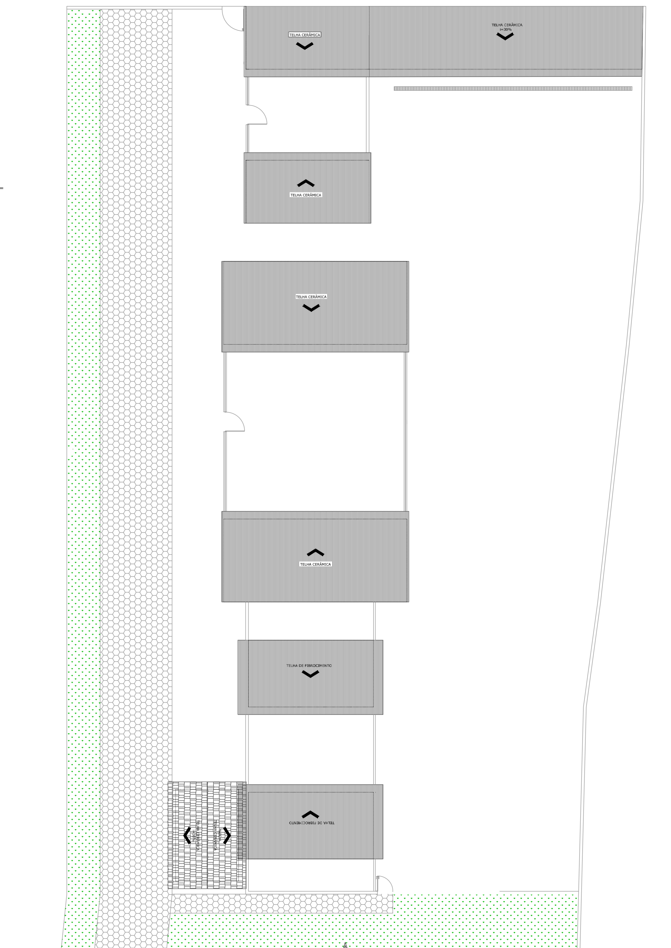
PLANTA DE COBERTURA - PARTE 2 Escala: 1:100
