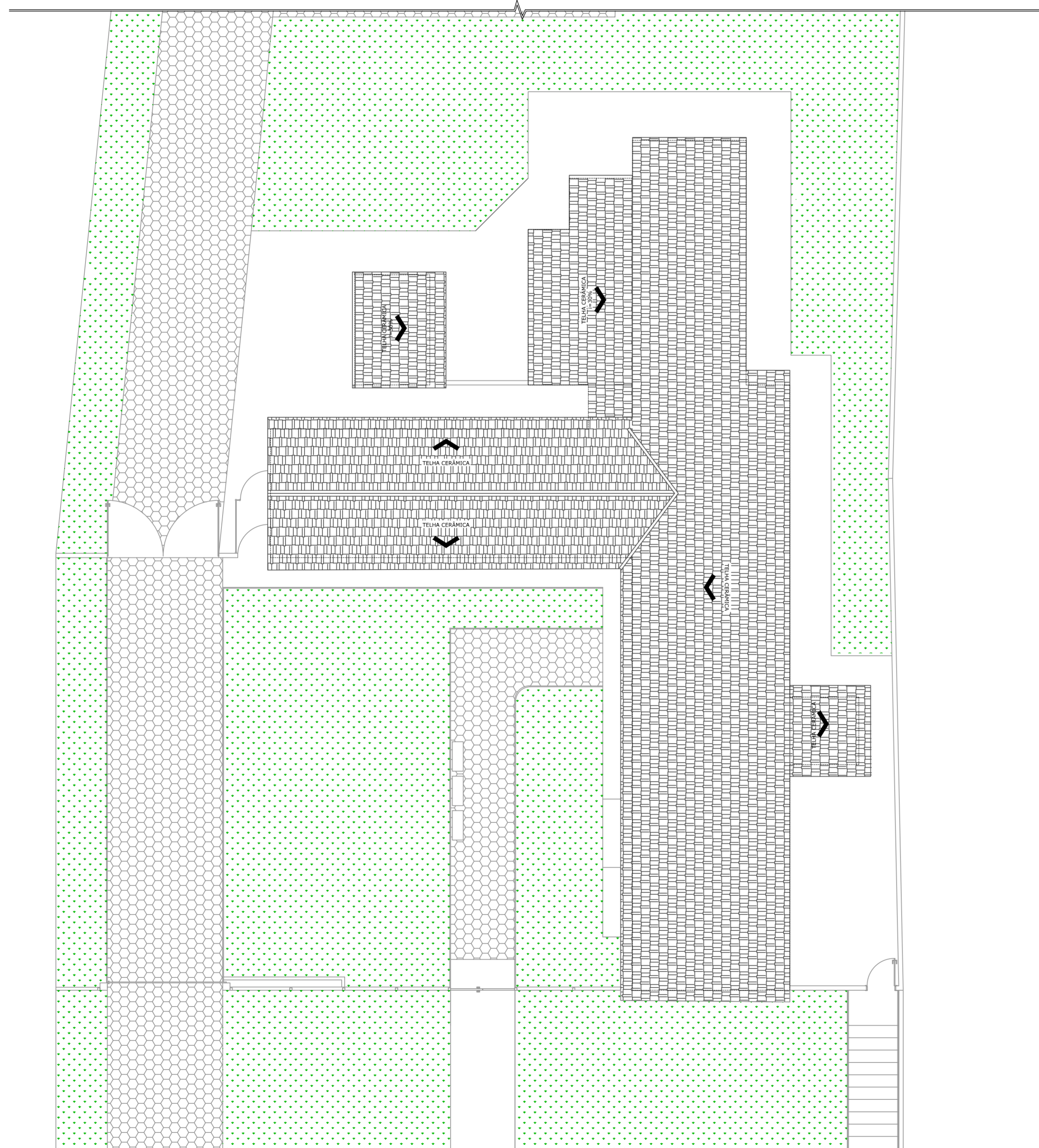
PLANTA DE COBERTURA - PARTE 1 Escala: 1:100
