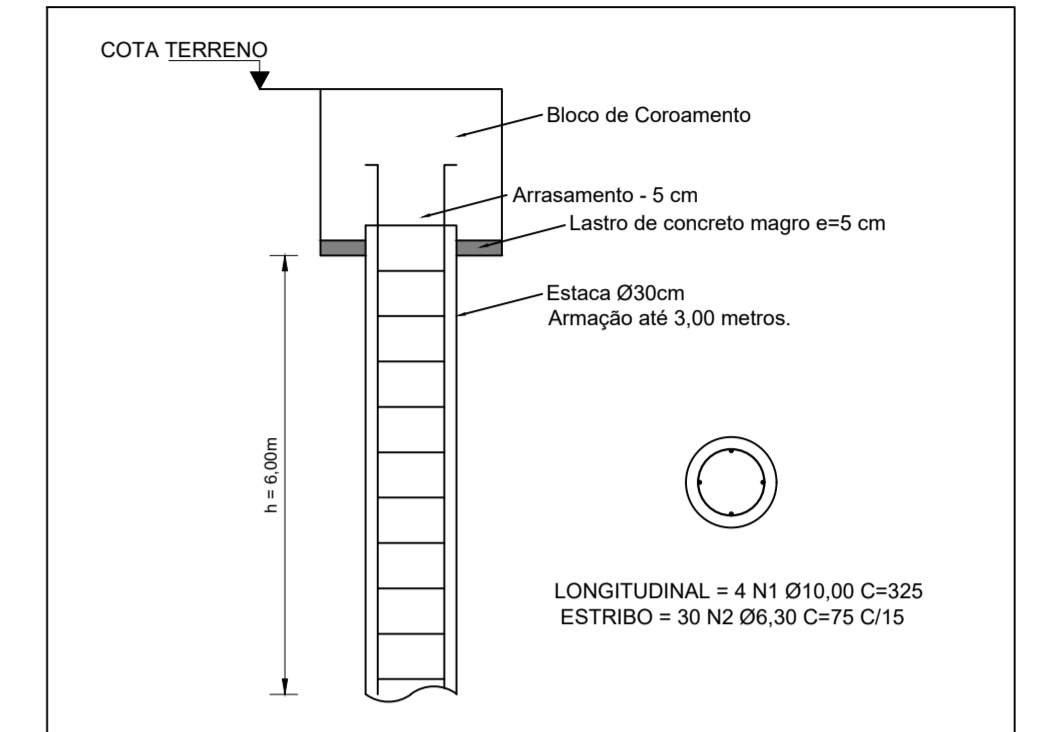
DETALHE TÍPICO DAS ESTACAS ESCALA 1:25
