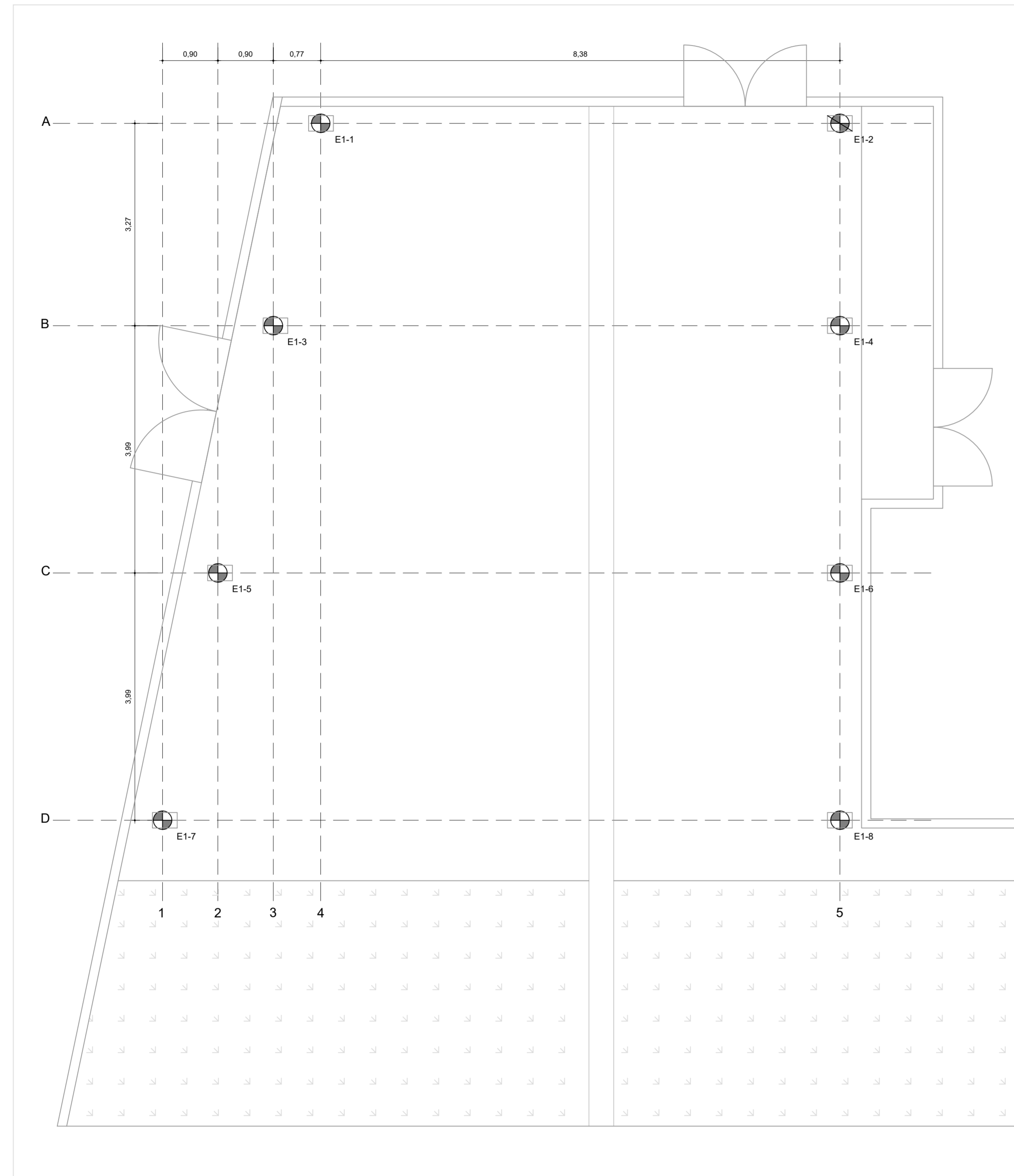
PLANTA DE LOCAÇÃO DAS ESTACAS ESCALA 1:50
