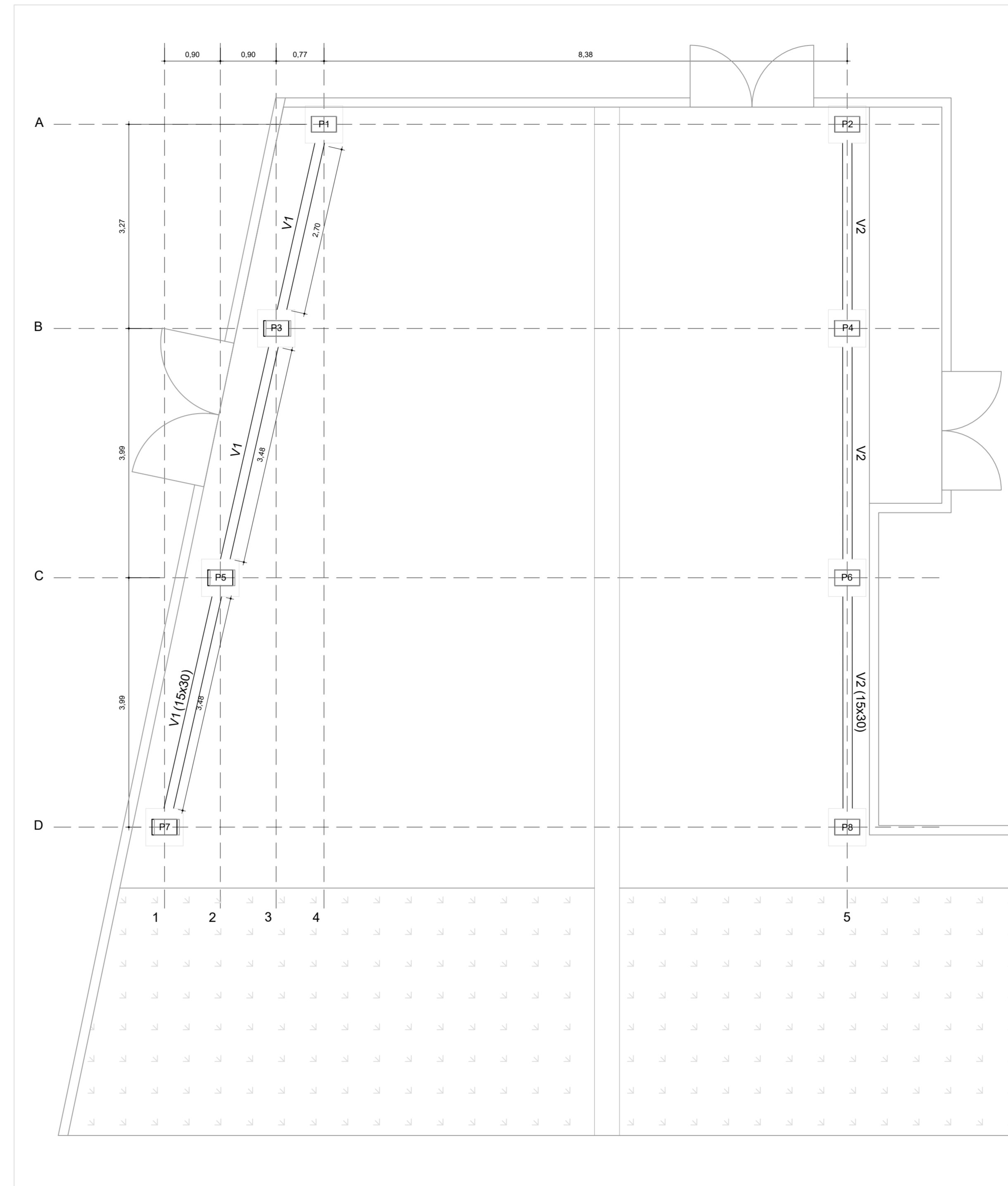
PLANTA DE LOCAÇÃO DAS CHAPAS DE BASE E VIGAS ESCALA 1:50
