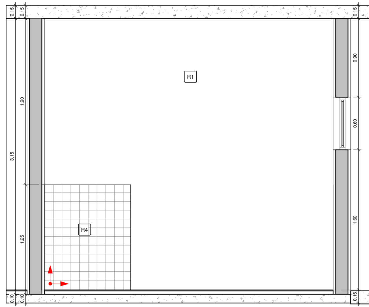
1 CONSULTÓRIO 4 VISTA 1 1 : 25
