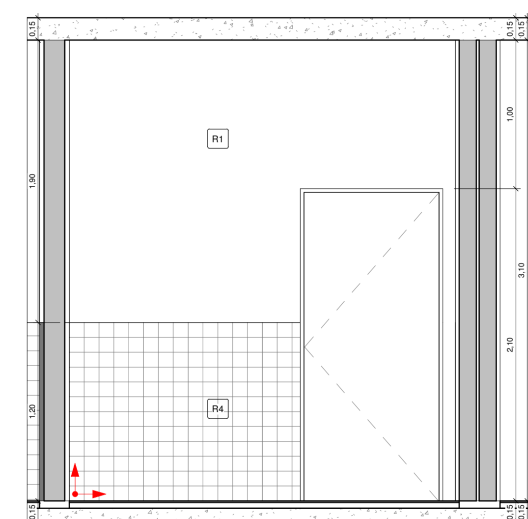
11 TRIAGEM DA UNIDADE VISTA 1 1 : 25
