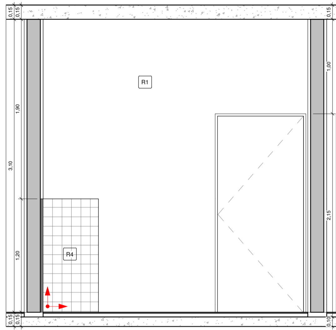
7 CONSULTÓRIO 1 VISTA 1 1 : 25
