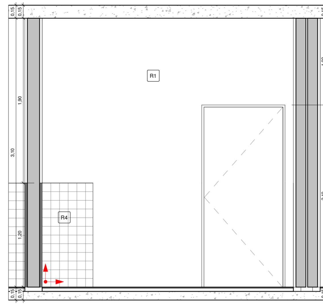
3 CONSULTÓRIO 3 VISTA 1 1 : 25
