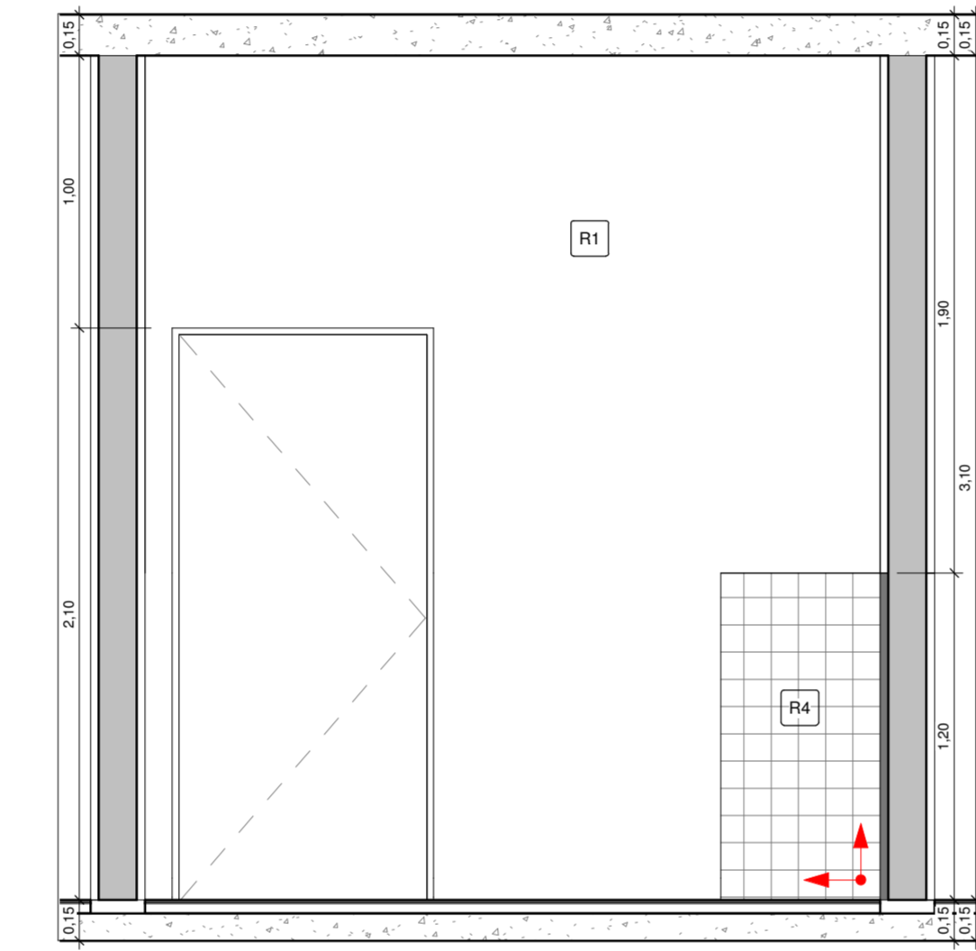
9 SALA DE CURATIVOS VISTA 1 1 : 25
