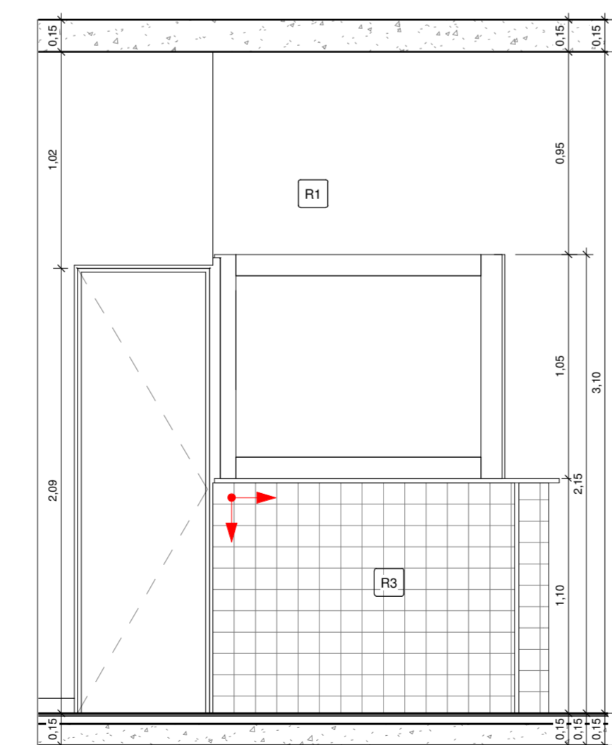
14 ESPERA/ RECEPÇÃO VISTA 1 1 : 25
