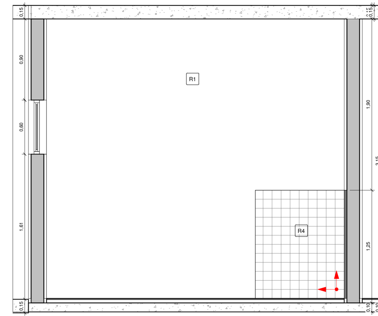
4 CONSULTÓRIO 3 VISTA 2 1 : 25
