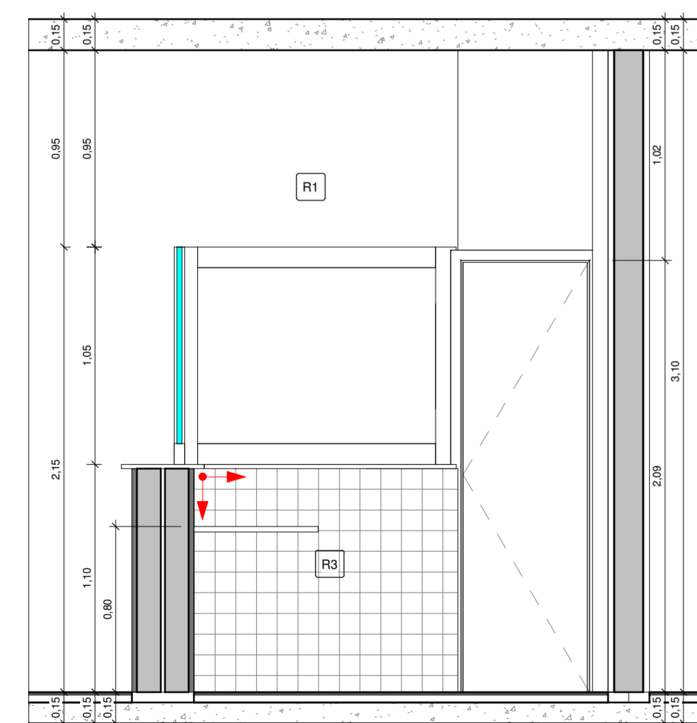
12 RECEPÇÃO VISTA 1 1 : 25
