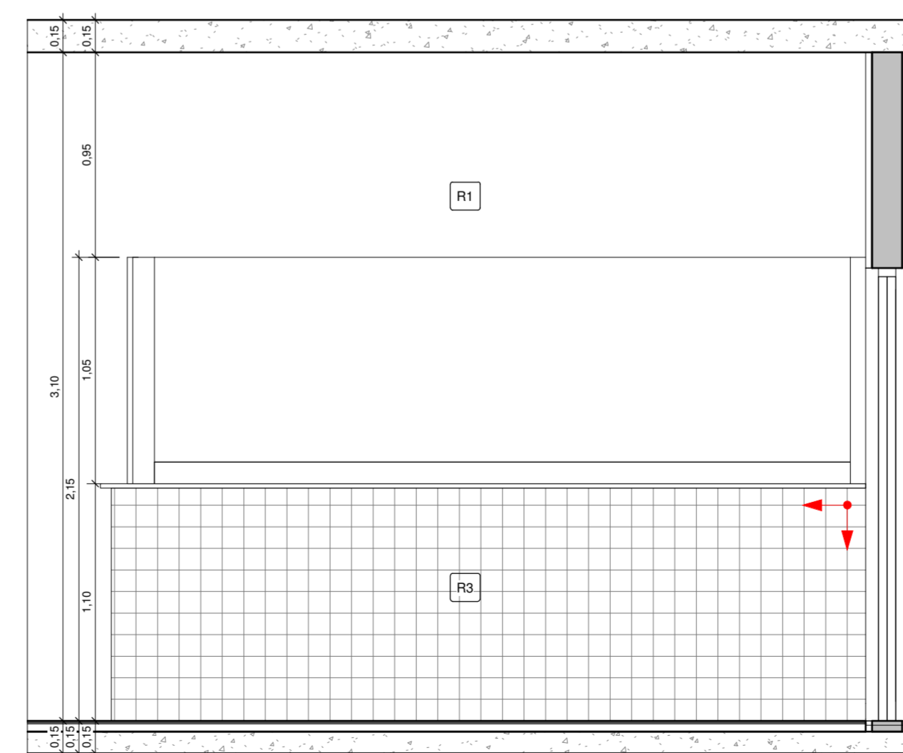
15 ESPERA/ RECEPÇÃO VISTA 2 1 : 25
