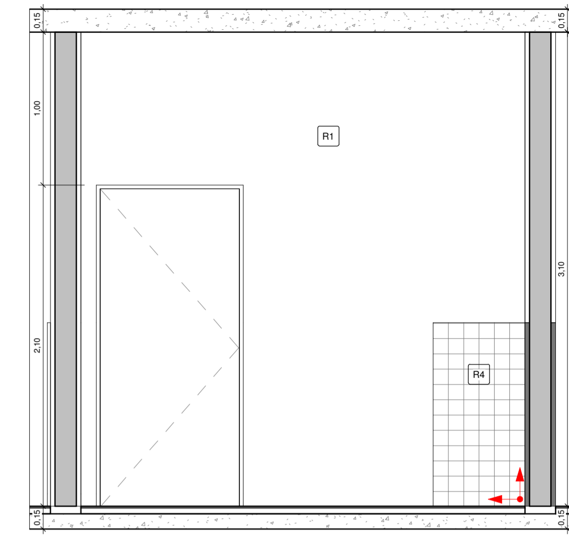
6 CONSULTÓRIO 2 VISTA 2 1 : 25
