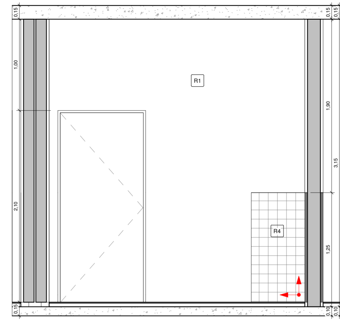
2 CONSULTÓRIO 4 VISTA 2 1 : 25
