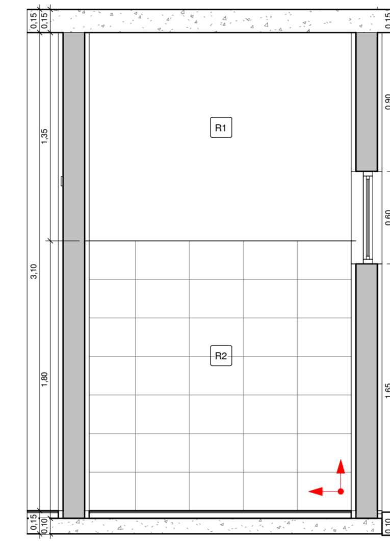
12 D.M.L. VISTA 4 1 : 25
