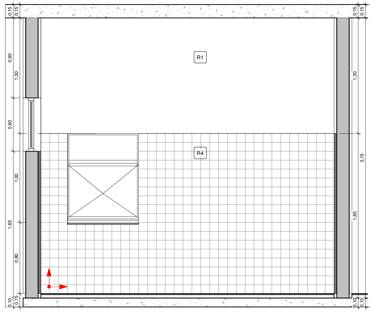
1 ESTERILIZAÇÃO VISTA 1 1 : 25
