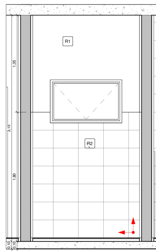
9 D.M.L. VISTA 1 1 : 25
