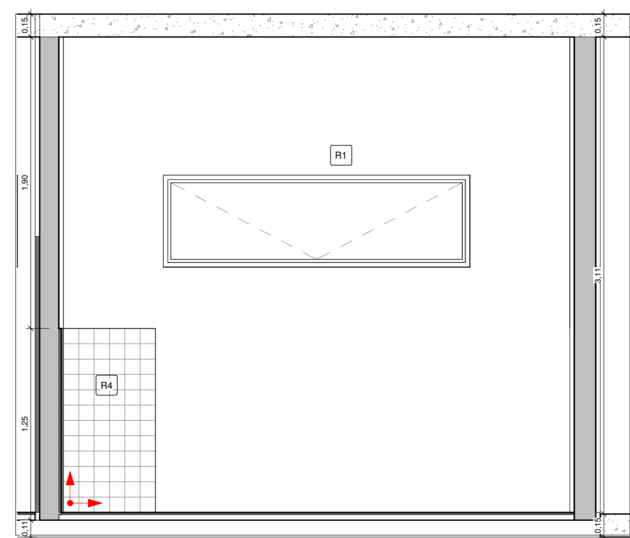
17 ODONTOLOGIA VISTA 1 1 : 25
