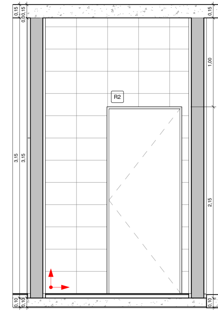
5 RESÍDUOS SÓLIDOS VISTA 1 1 : 25
