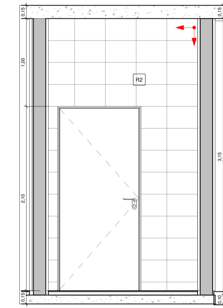
14 I.S. VISTA 2 1 : 25
