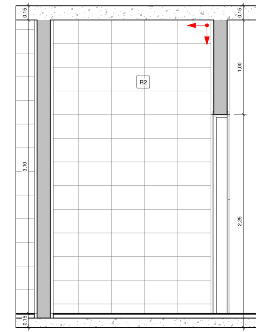
13 I.S. VISTA 1 1 : 25
