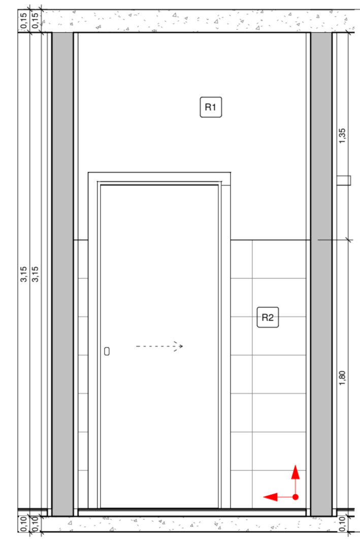
11 D.M.L. VISTA 3 1 : 25
