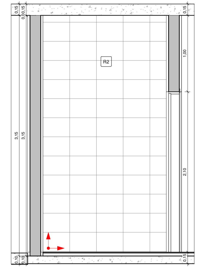
7 RESÍDUOS SÓLIDOS VISTA 3 1 : 25
