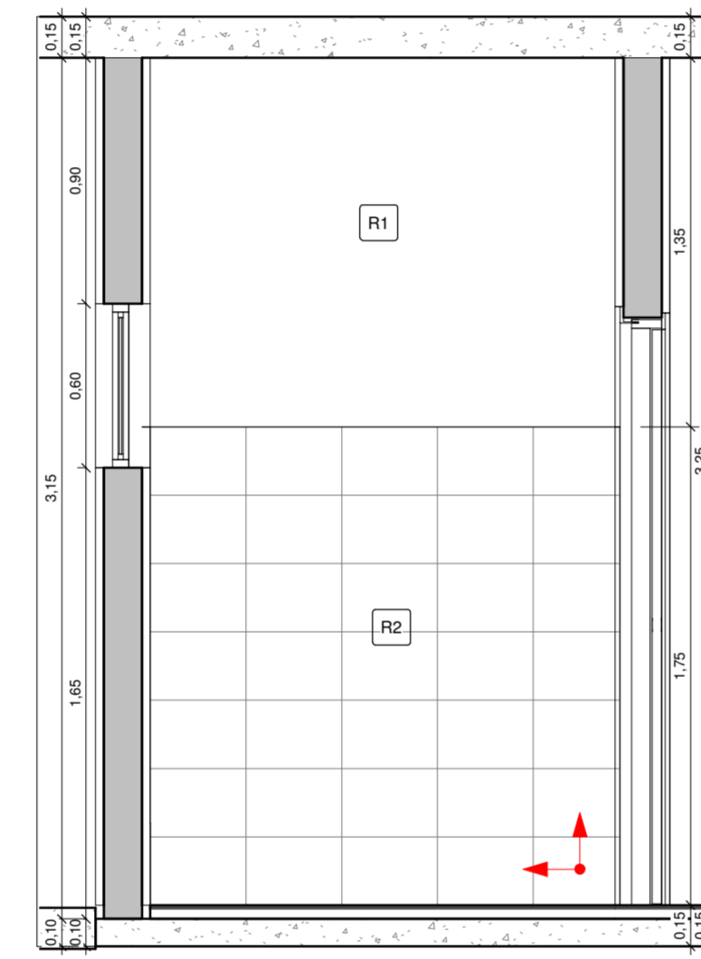
10 D.M.L. VISTA 2 1 : 25
