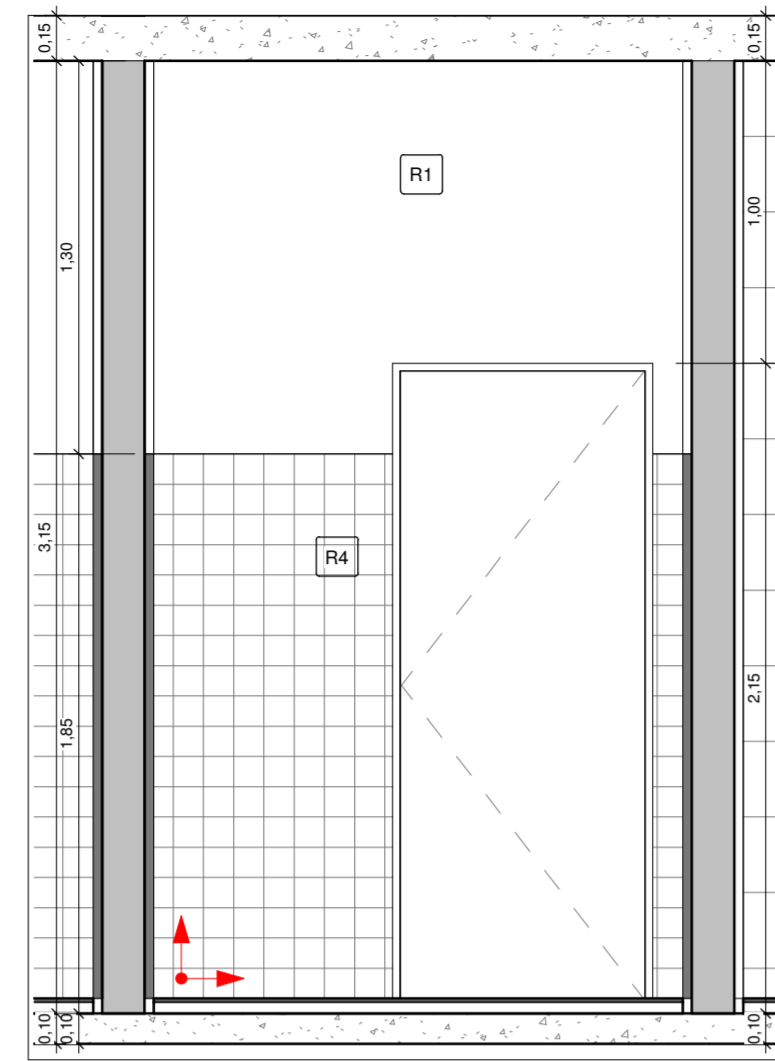
2 ESTERILIZAÇÃO VISTA 2 1 : 25
