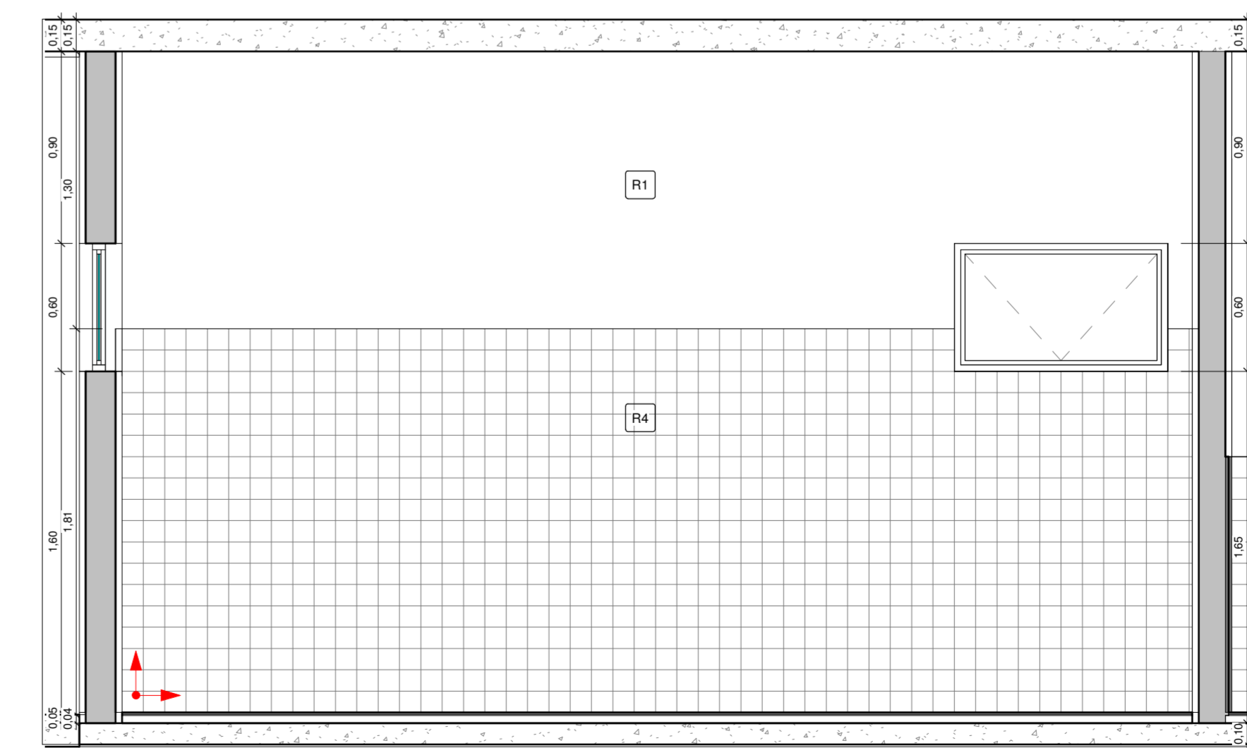
19 ESCOVÓDROMO VISTA 1 1 : 25
