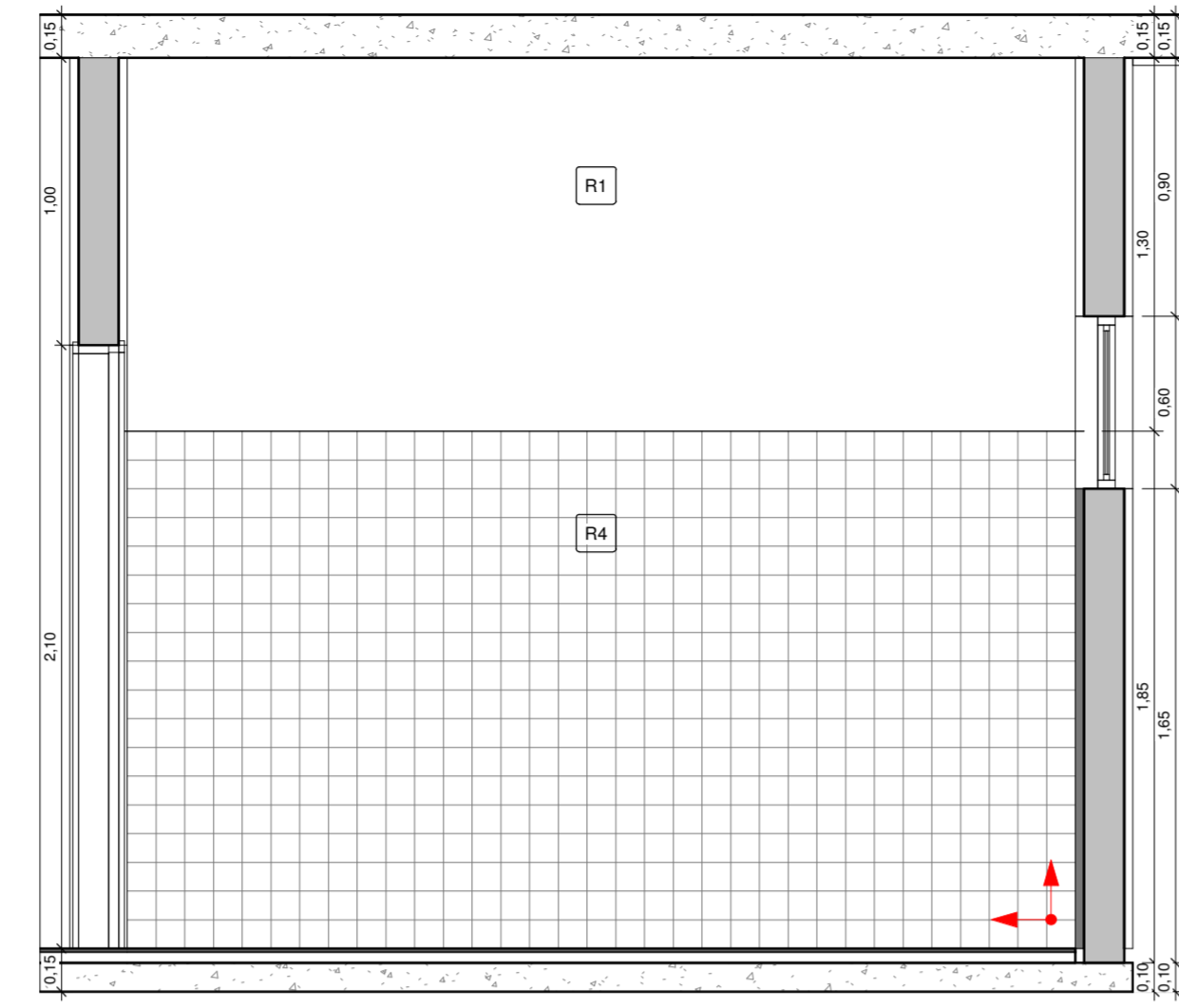
3 ESTERILIZAÇÃO VISTA 3 1 : 25
