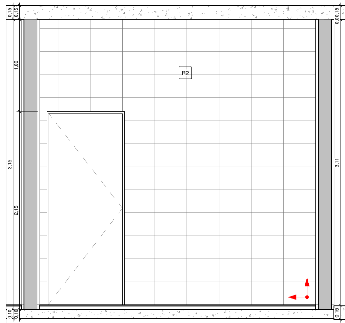
8 RESÍDUOS SÓLIDOS VISTA 4 1 : 25
