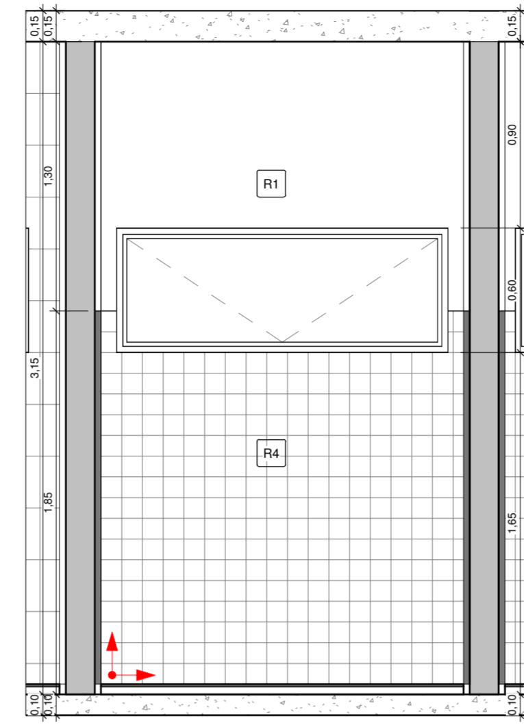
4 ESTERILIZAÇÃO VISTA 4 1 : 25
