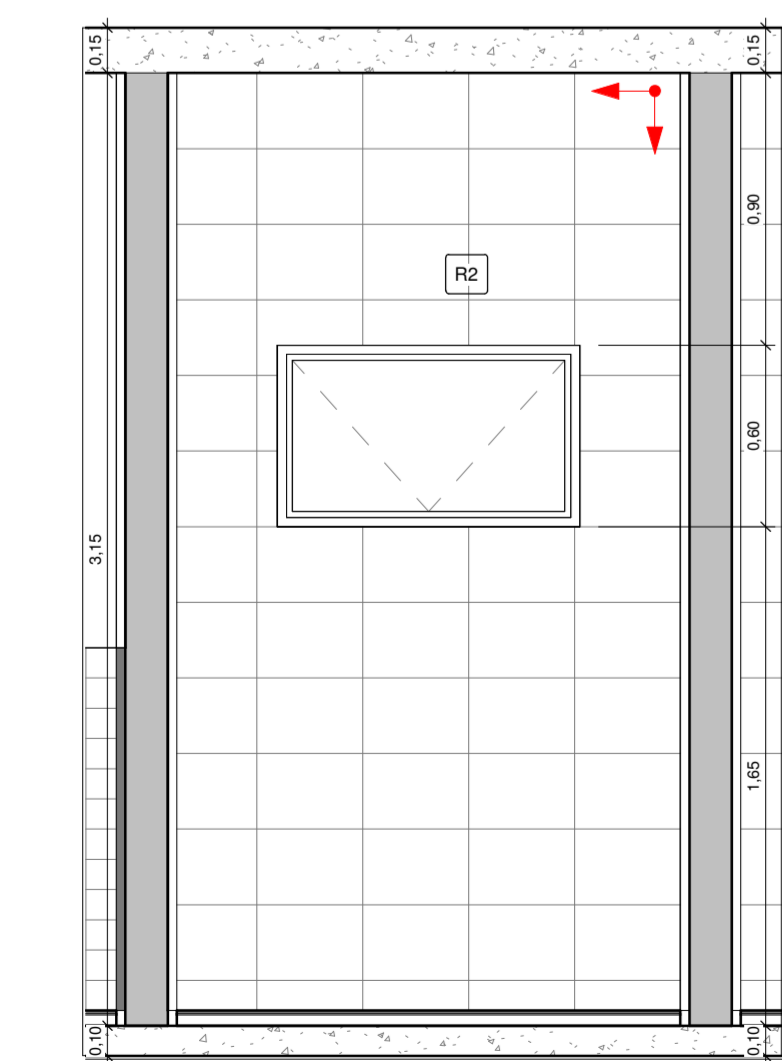
15 I.S. VISTA 3 1 : 25
