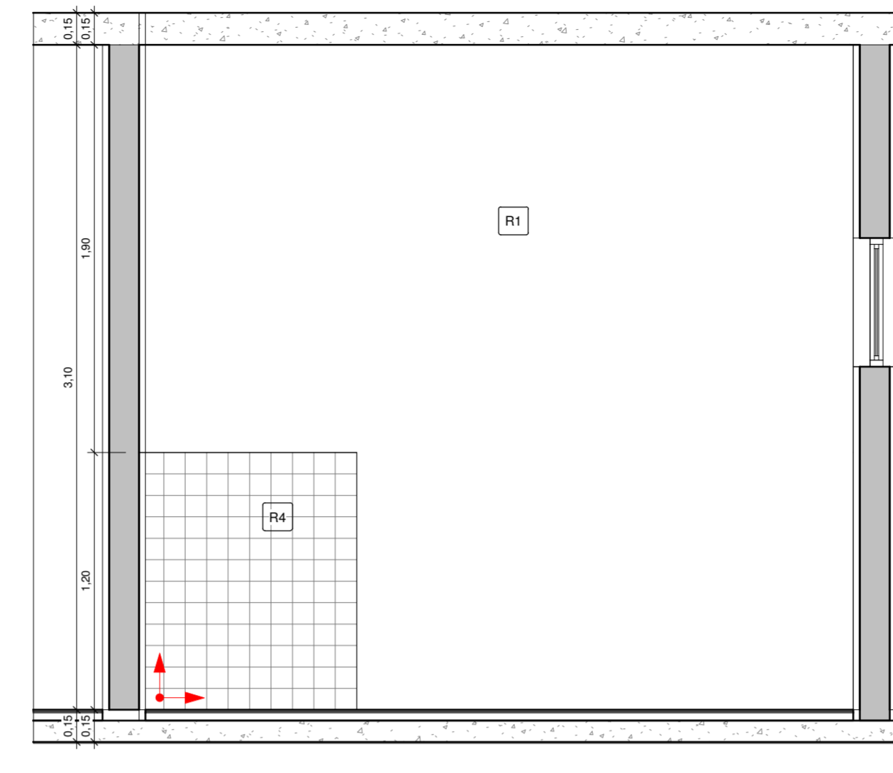
4 CONSULTÓRIO 8 VISTA 1 1 : 25
