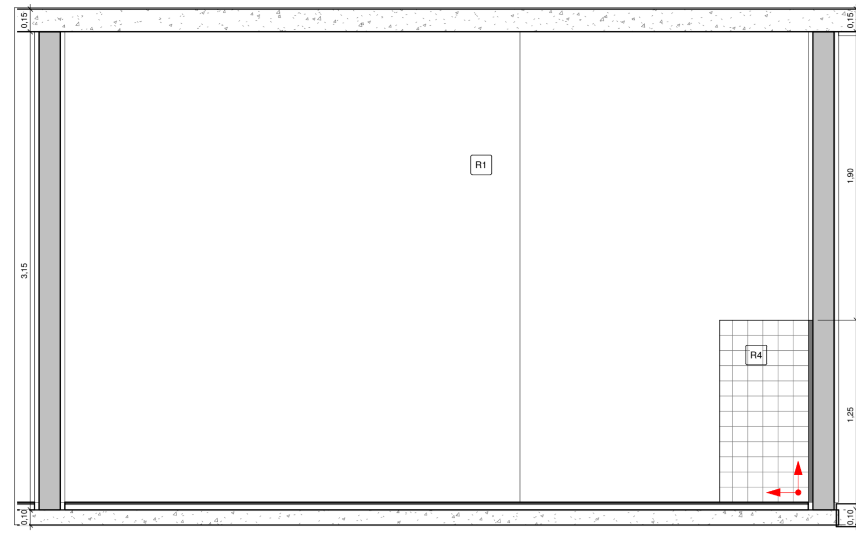
2 CONSULTÓRIO GINECOLÓGICO 01 VISTA 2 1 : 25
