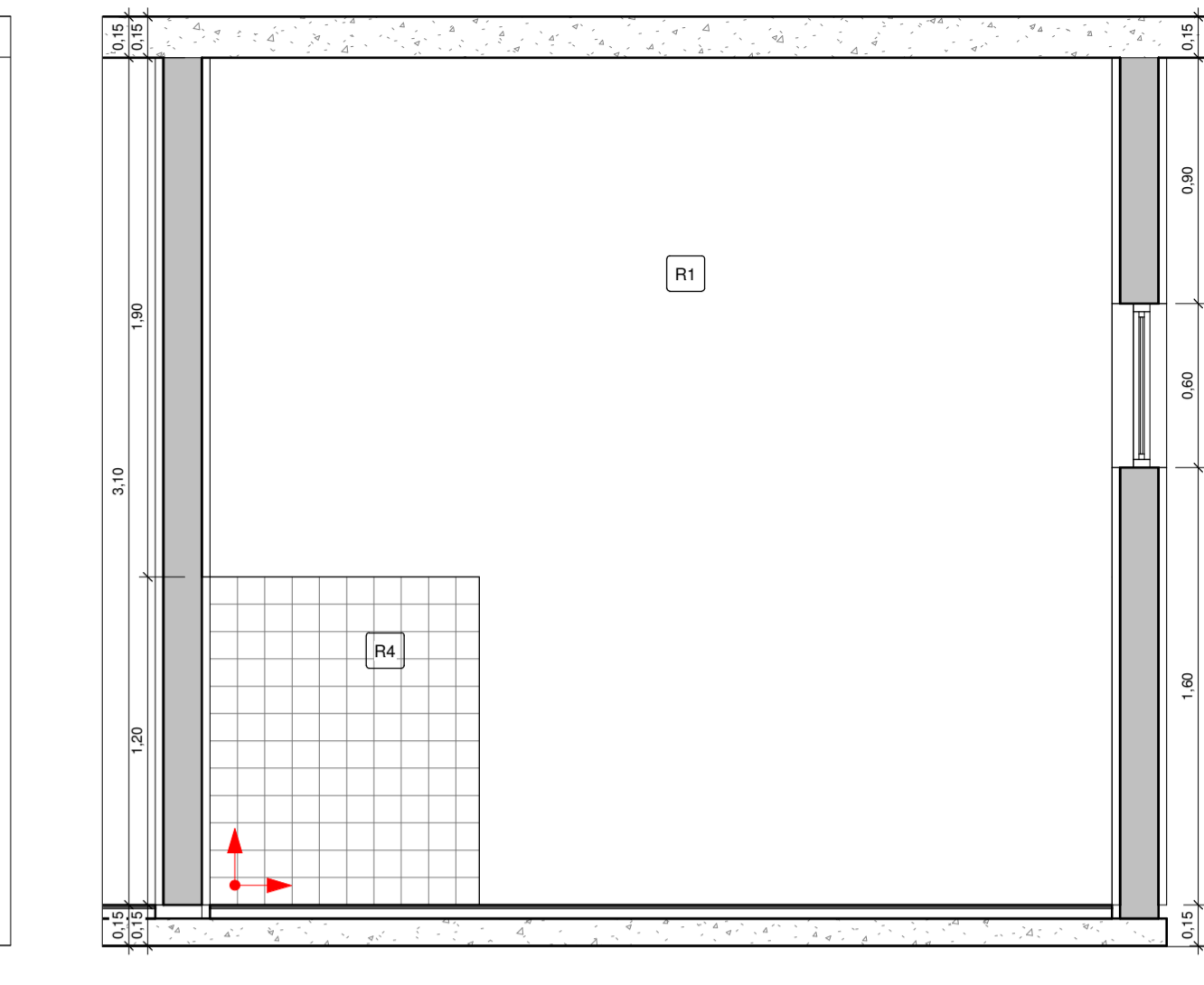
6 CONSULTÓRIO 9 VISTA 2 1 : 25
