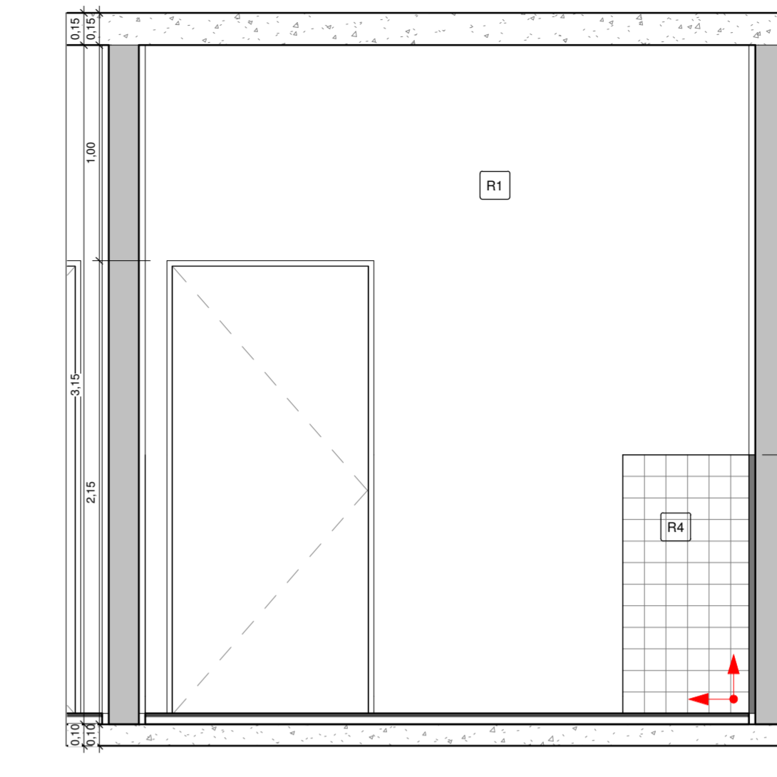
5 CONSULTÓRIO 9 VISTA 1 1 : 25
