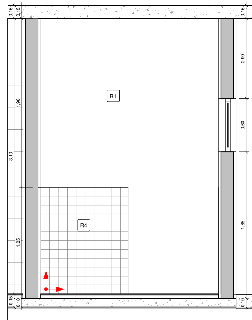
1 CONSULTÓRIO GINECOLÓGICO 01 VISTA 1 1 : 25
