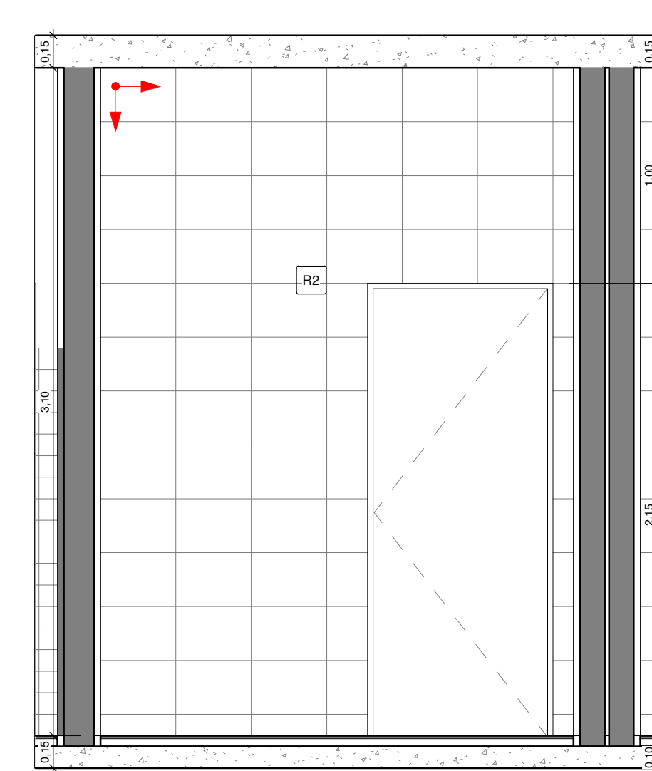
5 VEST. M. VISTA 2 1 : 25
