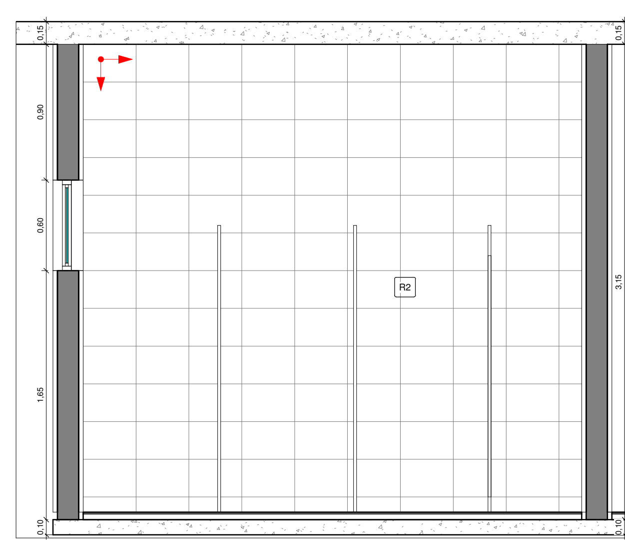
4 VEST. M. VISTA 1 1 : 25
