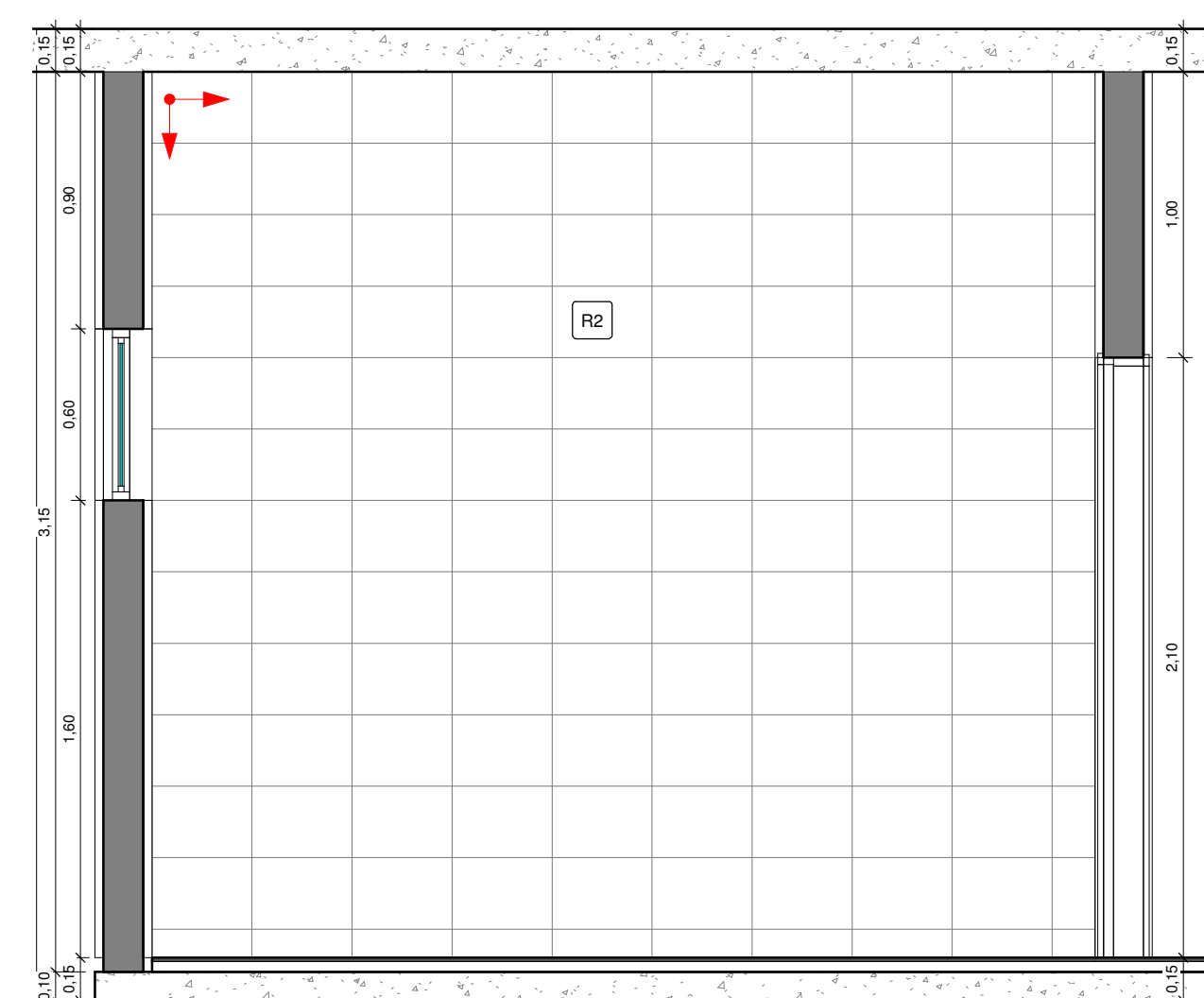
8 VEST. F. VISTA 1 1 : 25
