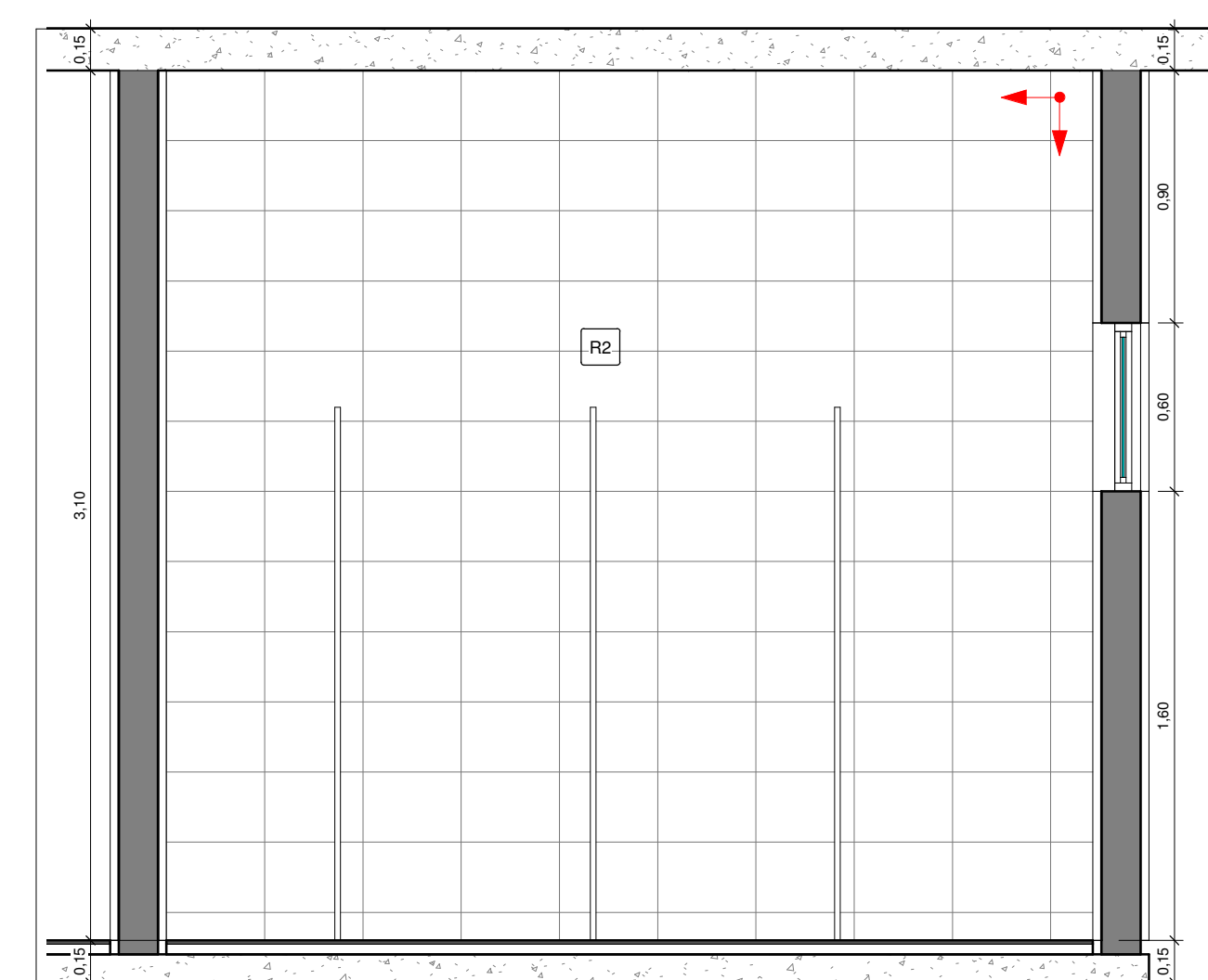
10 VEST. F. VISTA 3 1 : 25
