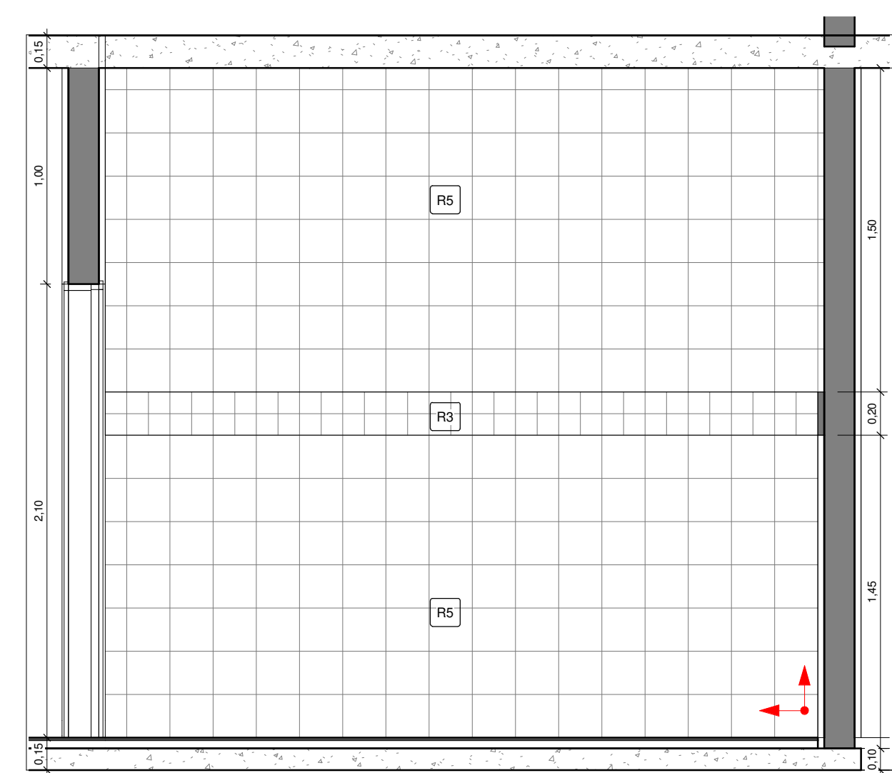
3 COPA VISTA 3 1 : 25
