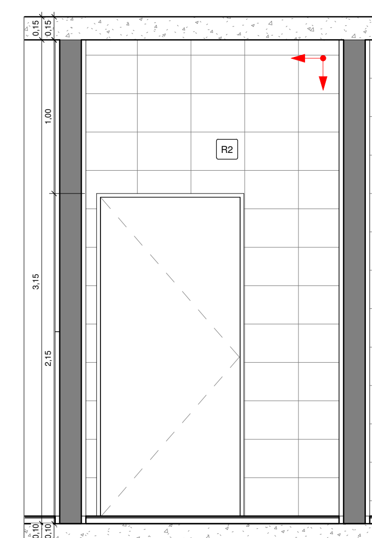
17 I.S. VISTA 6 1 : 25
