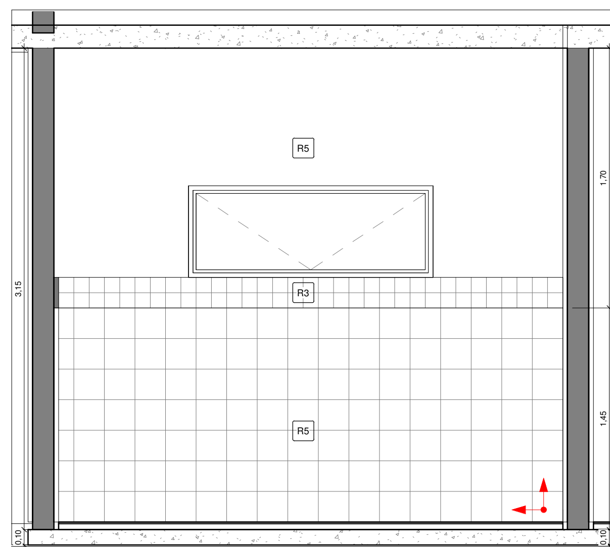
1 COPA VISTA 1 1 : 25
