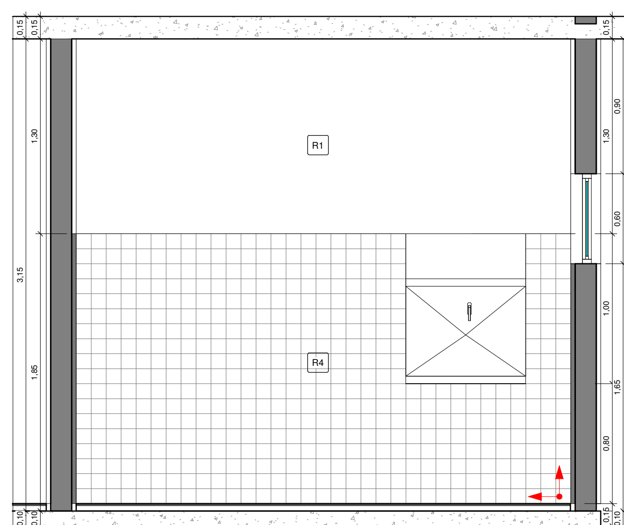
13 LAVAGEM E DESINFECÇÃO VISTA 3 1 : 25
