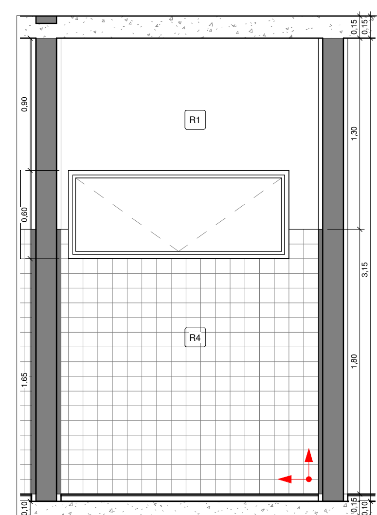
14 LAVAGEM E DESINFECÇÃO VISTA 4 1 : 25
