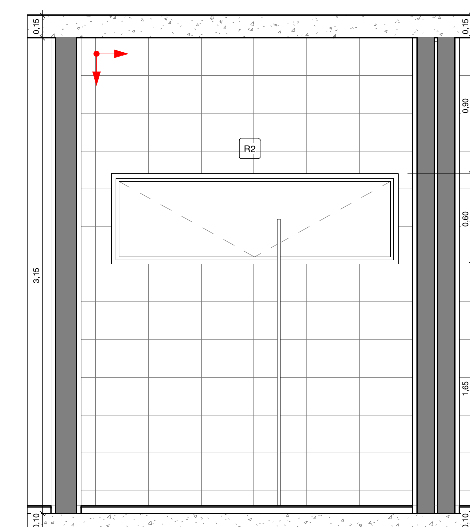
11 VEST. F. VISTA 4 1 : 25
