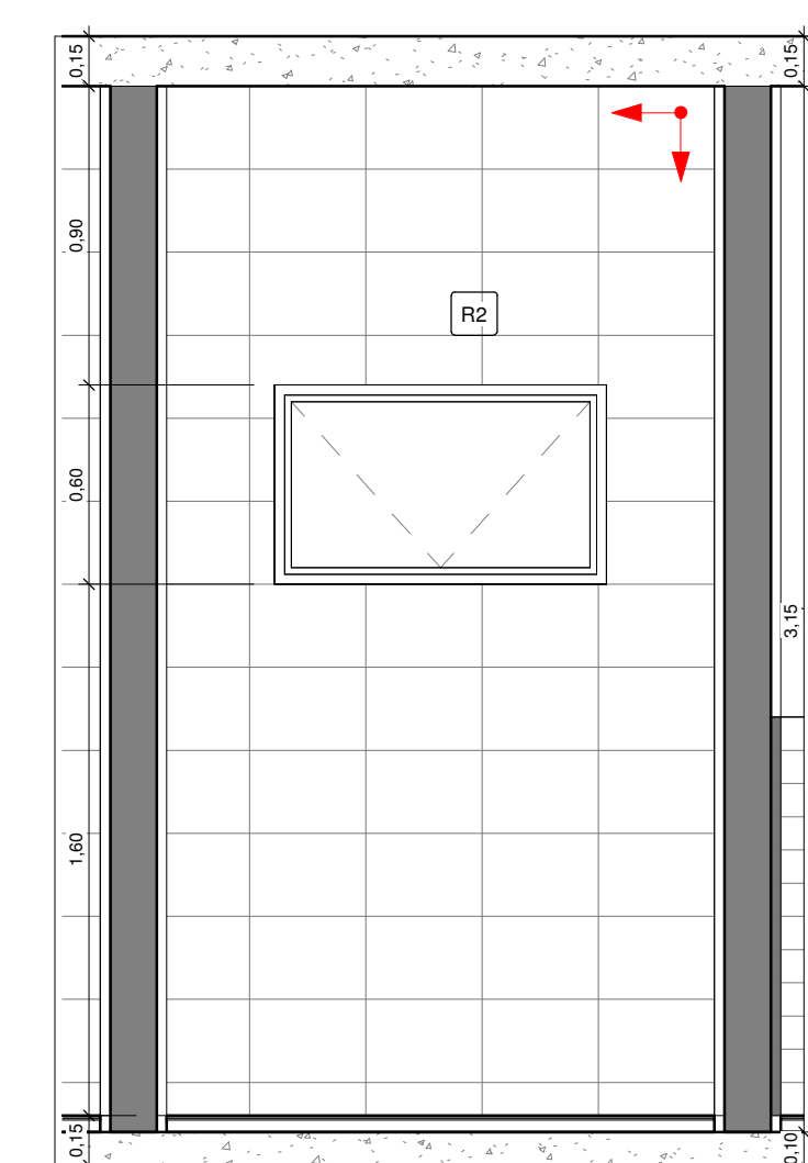
18 I.S. VISTA 7 1 : 25
