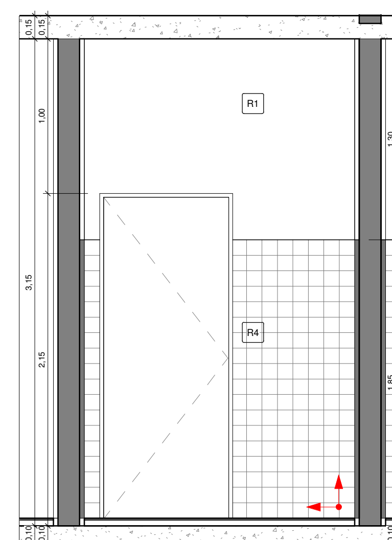
12 LAVAGEM E DESINFECÇÃO VISTA 2 1 : 25
