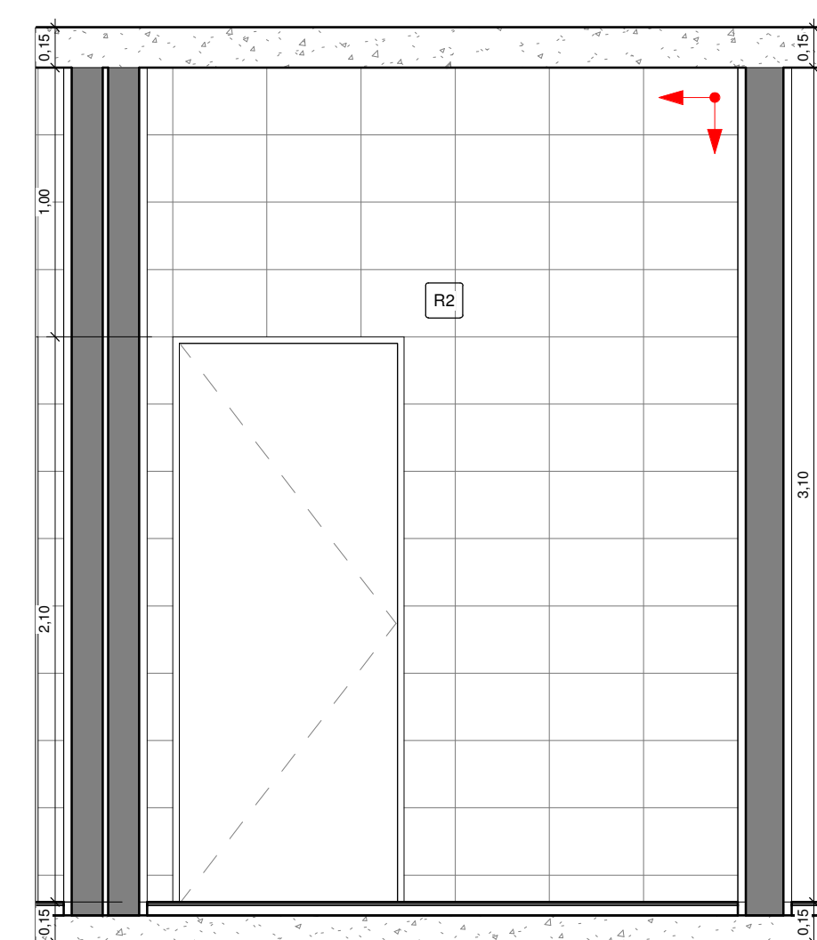
9 VEST. F. VISTA 2 1 : 25
