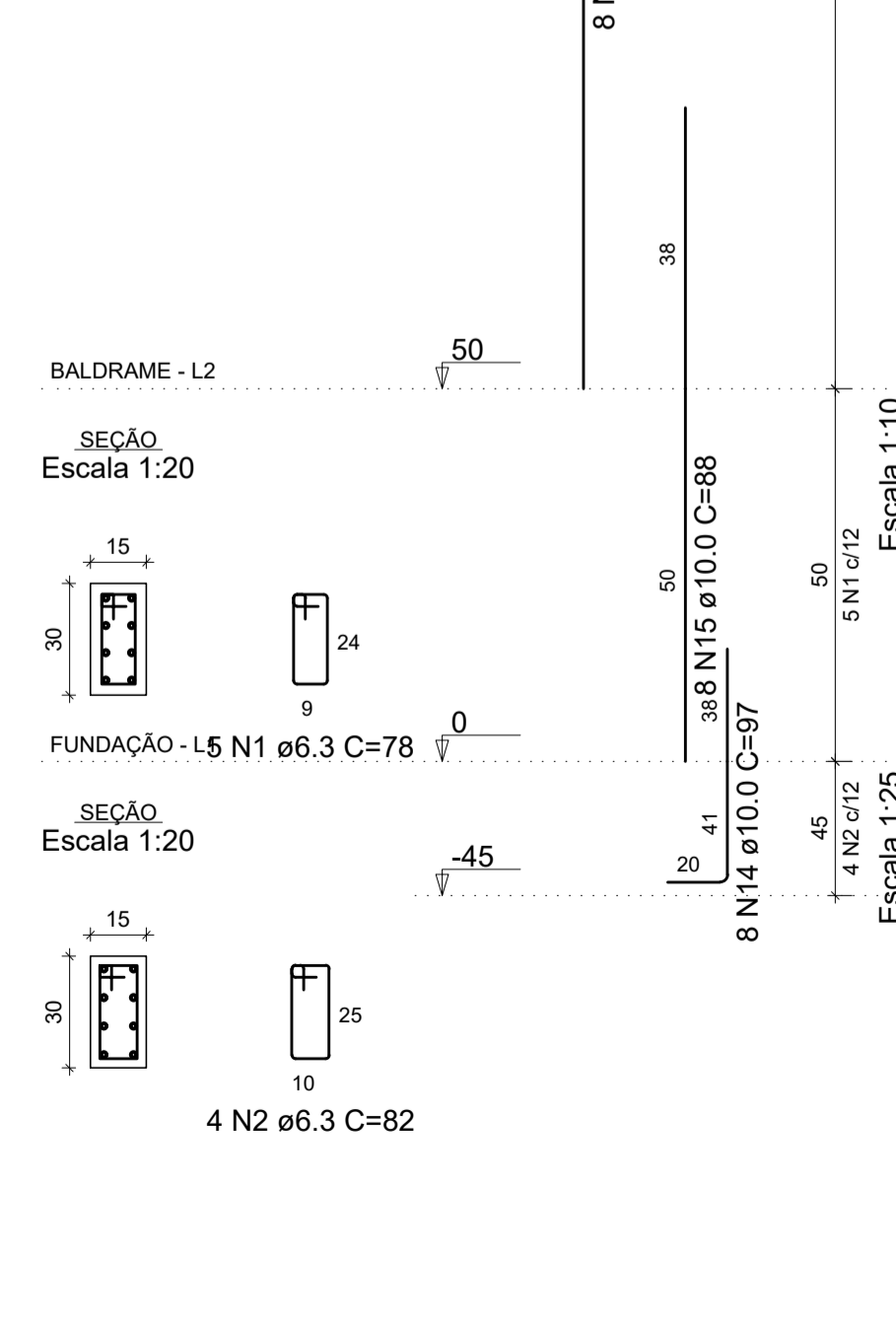
DETALHAMENTO DOS PILARES Escala INDICADA
