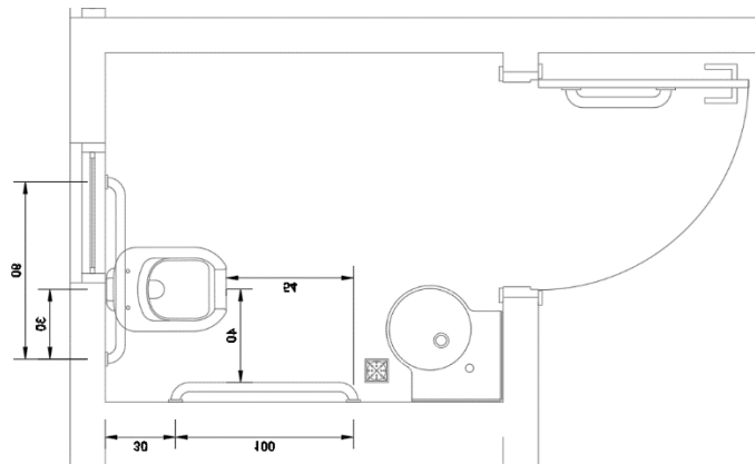
Figura 15 - Detalhamento Barras de Apoio
