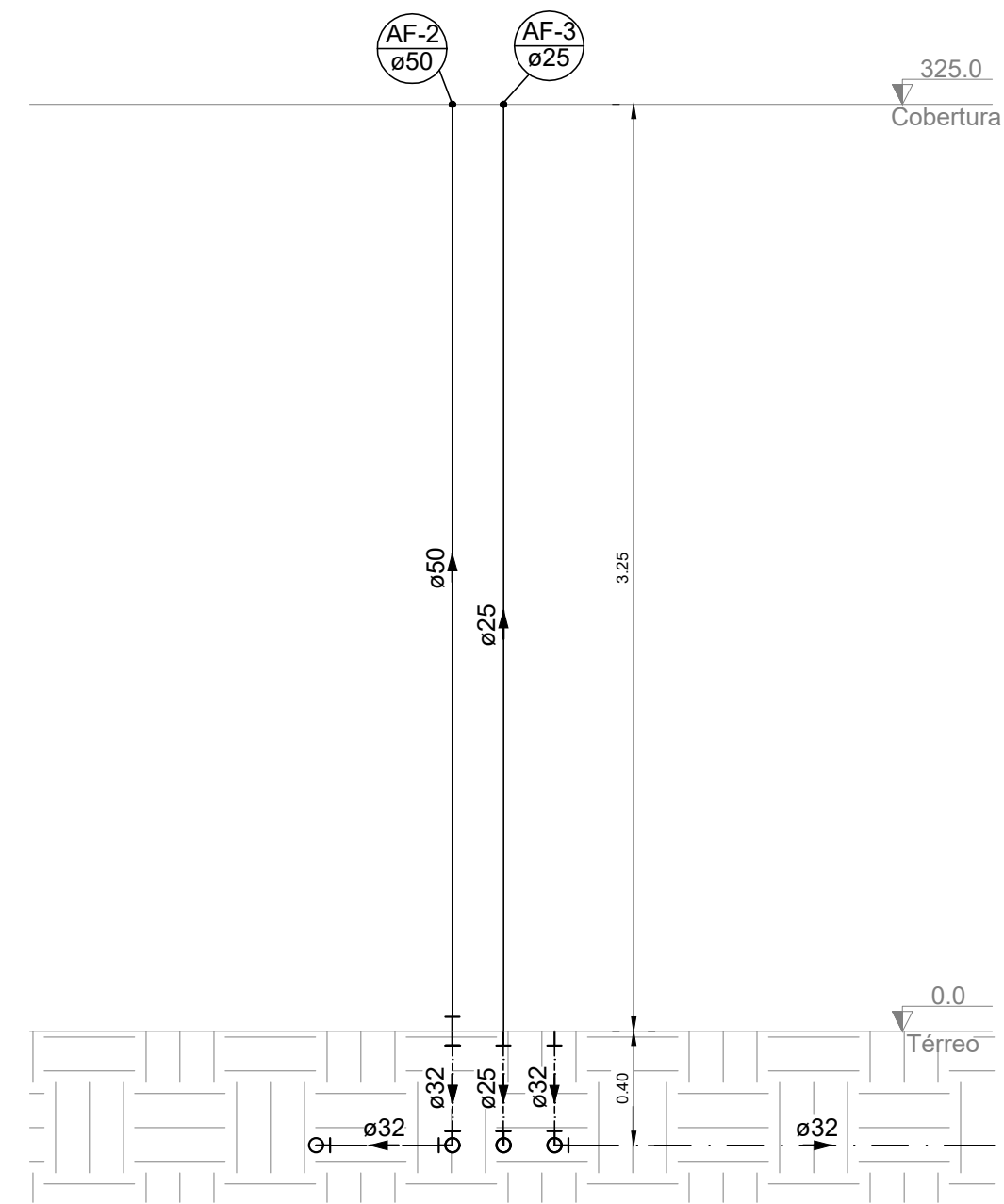
DETALHE HID-1 ESCALA 1:25
