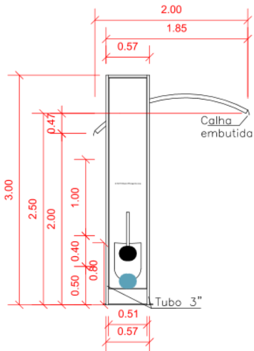
VISTA LATERAL
