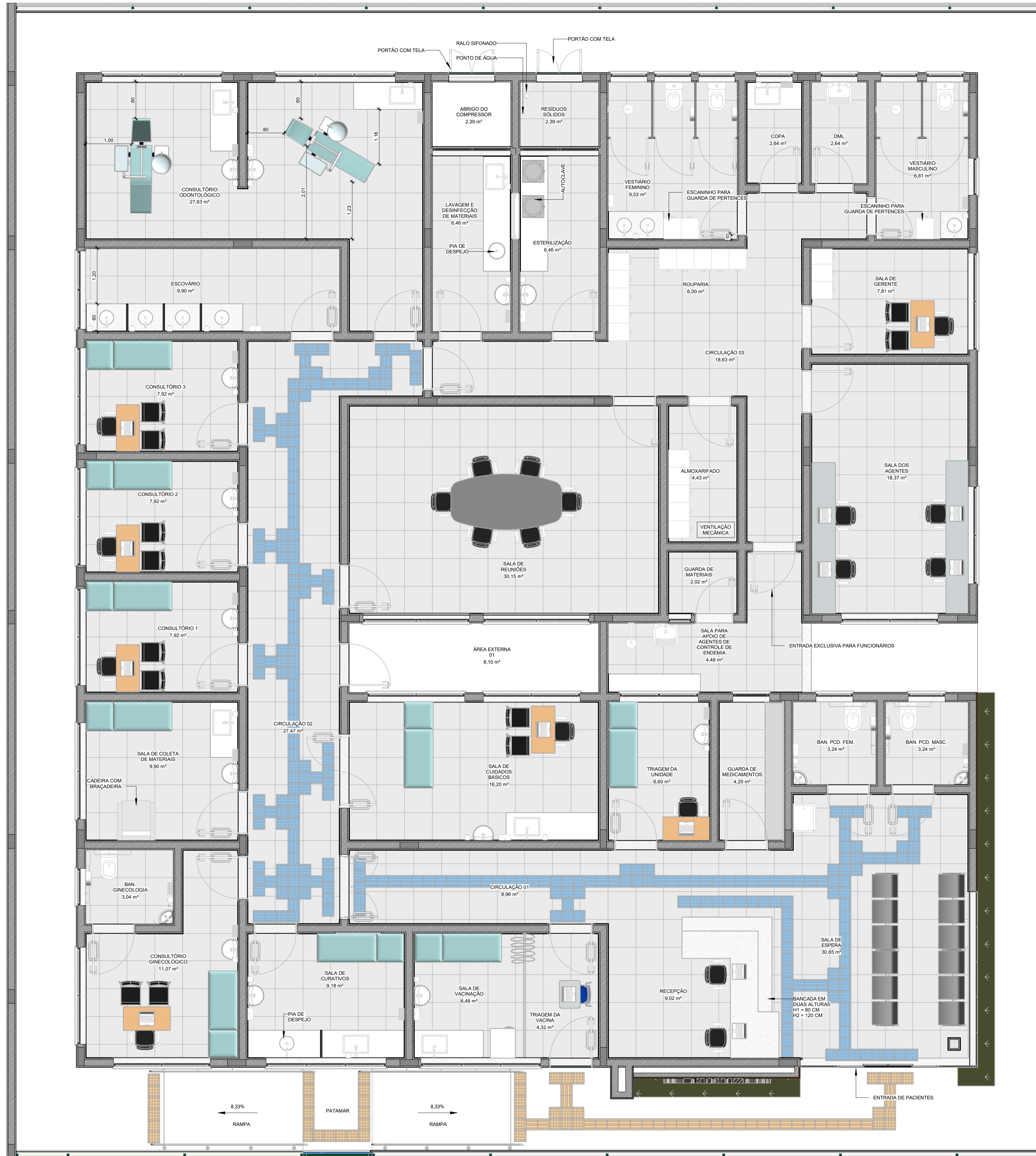
1 PLANTA DE LAYOUT 1 : 50
