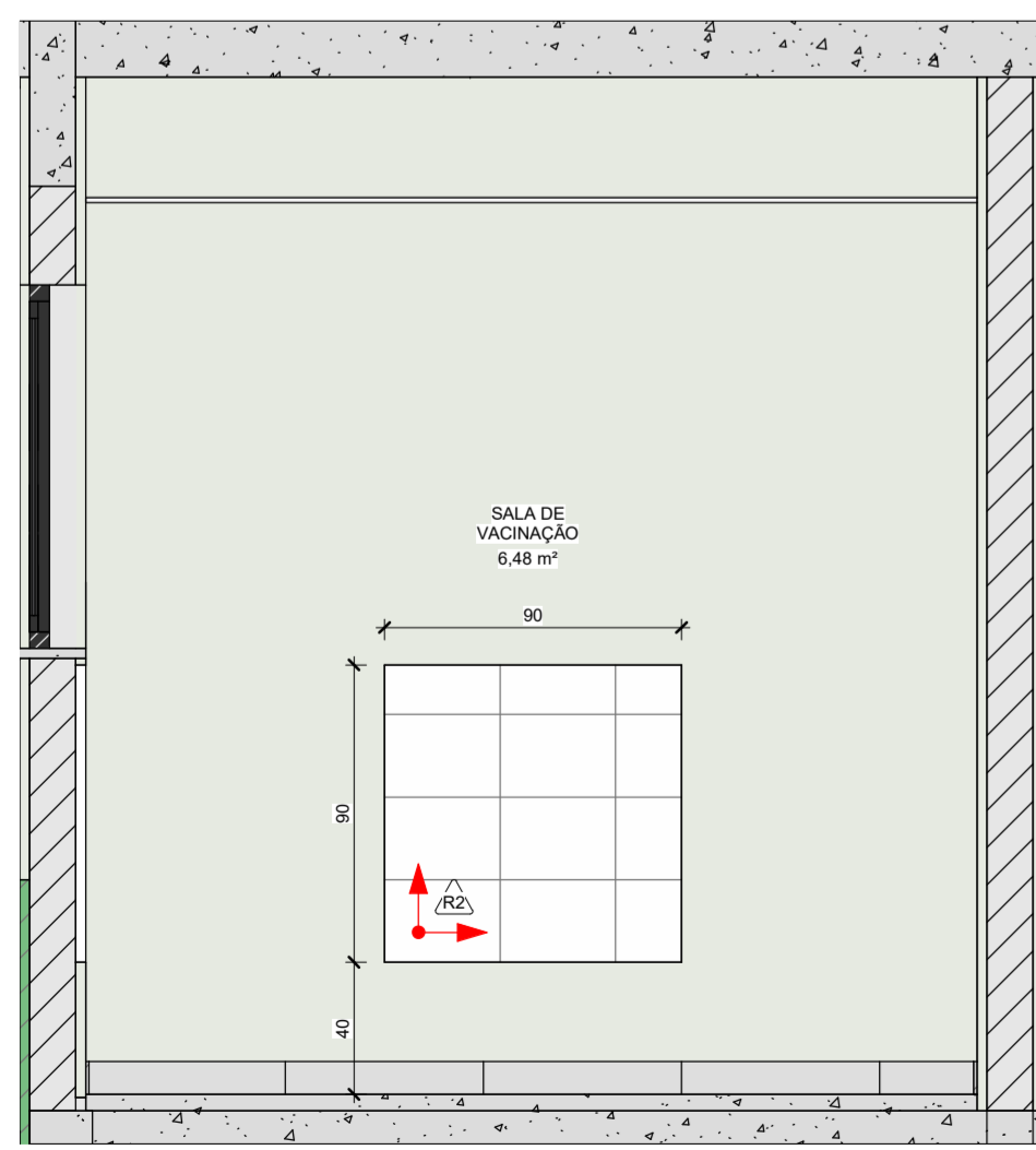
17 PAGINAÇÃO SALA DE VACINAÇÃO (1) 1 : 25
