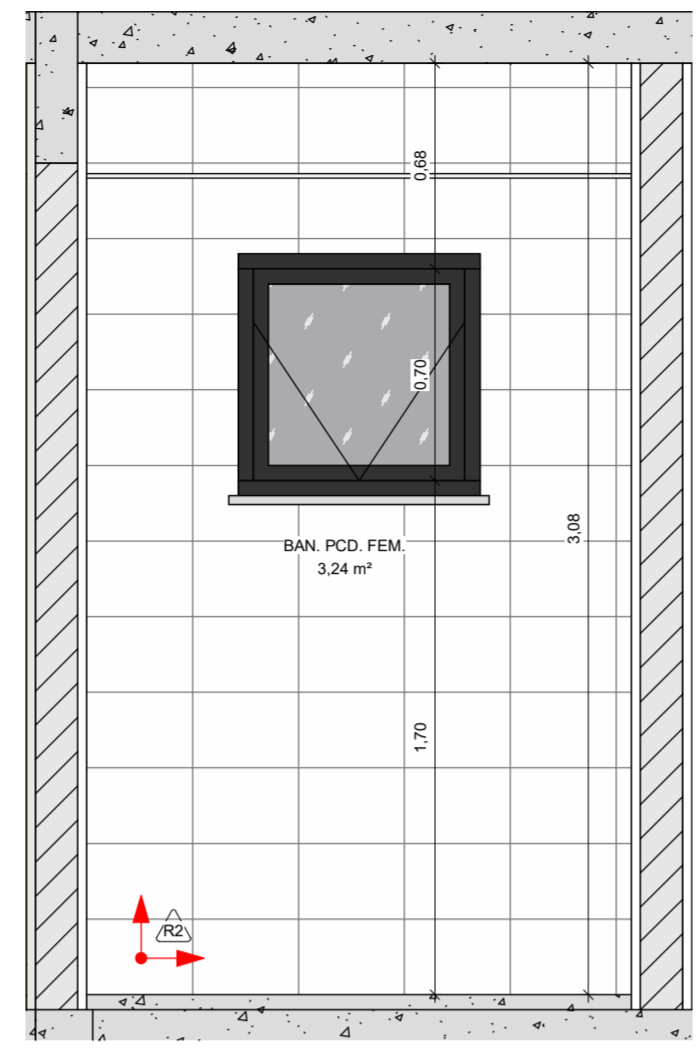
5 PAGINAÇÃO BAN. PNE. FEM. (1) 1 : 25
