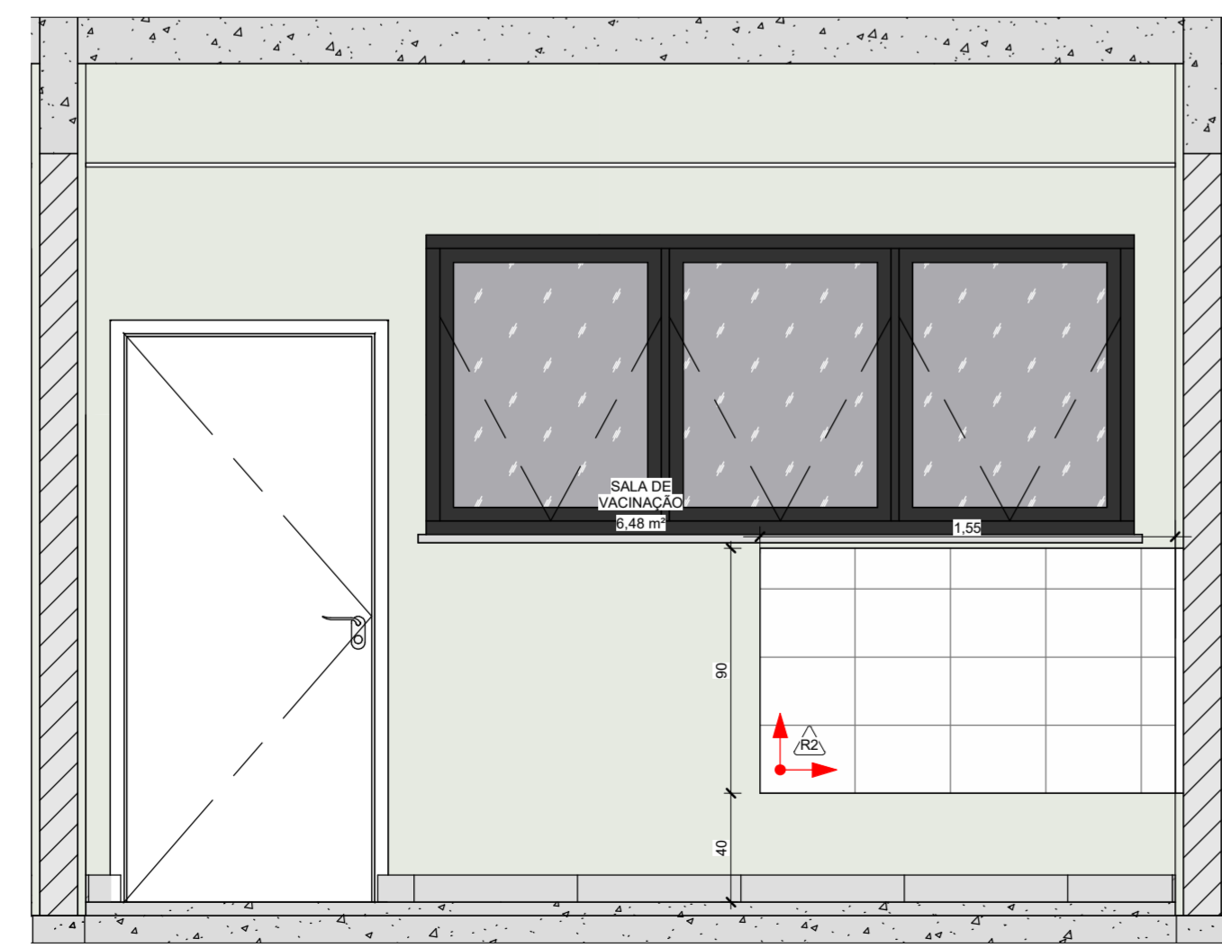
18 PAGINAÇÃO SALA DE VACINAÇÃO (2) 1 : 25
