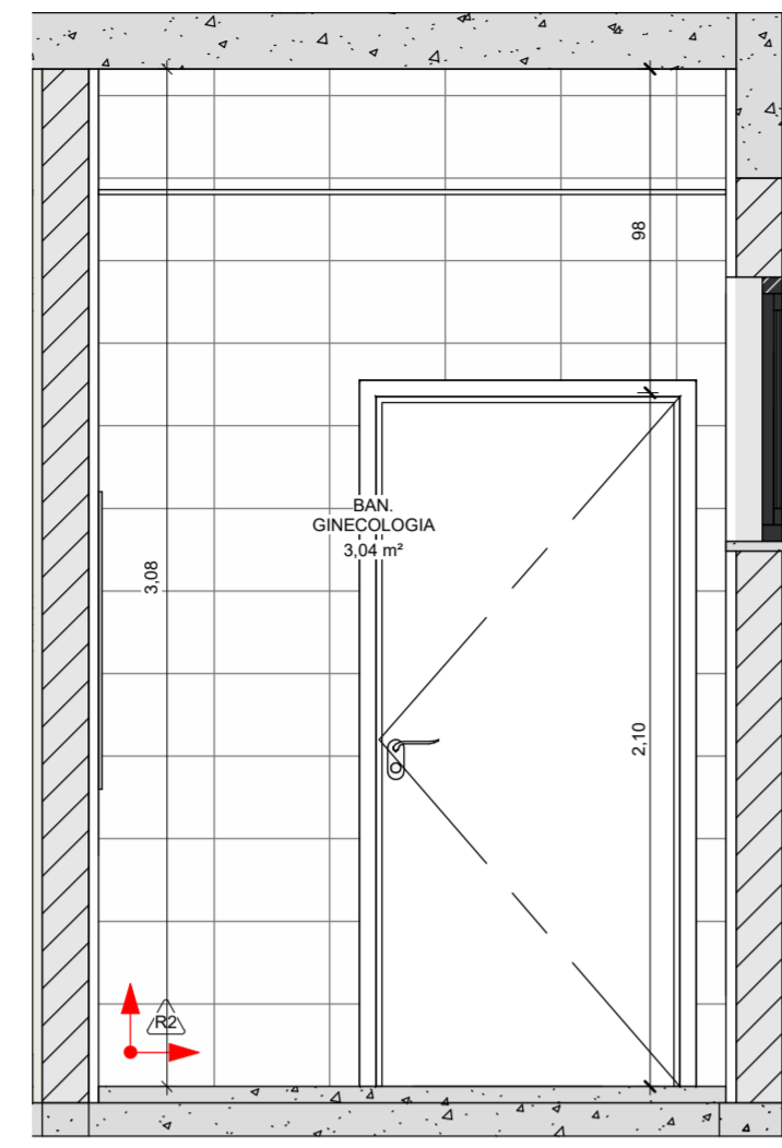
3 PAGINAÇÃO BAN. GINECOLOGIA (3) 1 : 25
