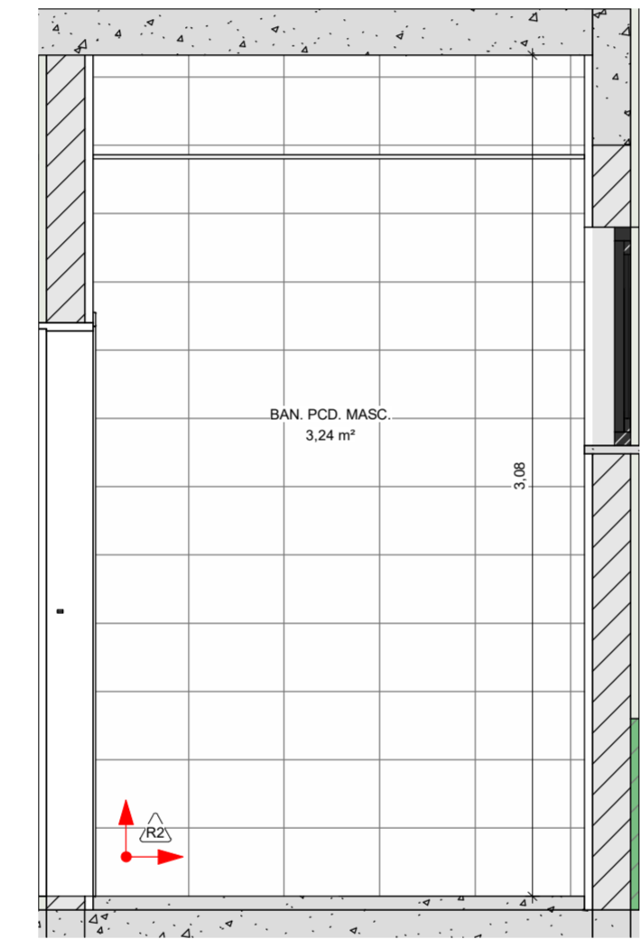
12 PAGINAÇÃO BAN. PNE. MASC. (4) 1 : 25
