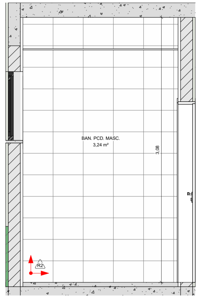
10 PAGINAÇÃO BAN. PNE. MASC. (2) 1 : 25
