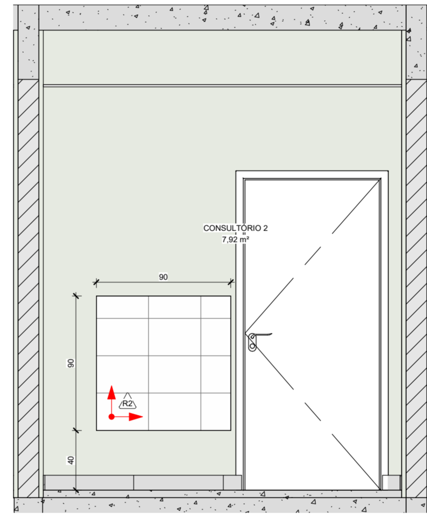
14 PAGINAÇÃO CONSULTÓRIO 2 1 : 25
