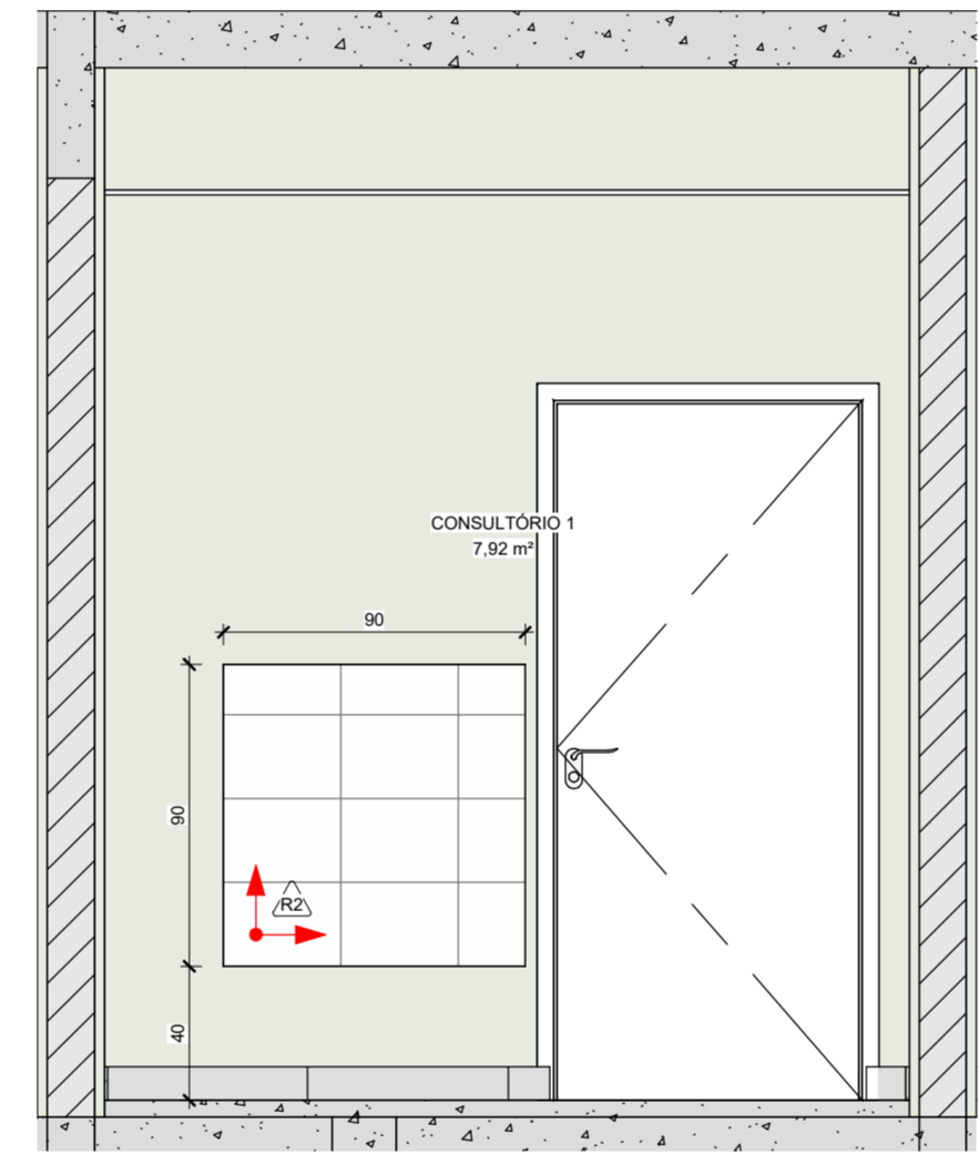
13 PAGINAÇÃO CONSULTÓRIO 1 1 : 25
