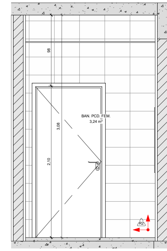
7 PAGINAÇÃO BAN. PNE. FEM. (3) 1 : 25
