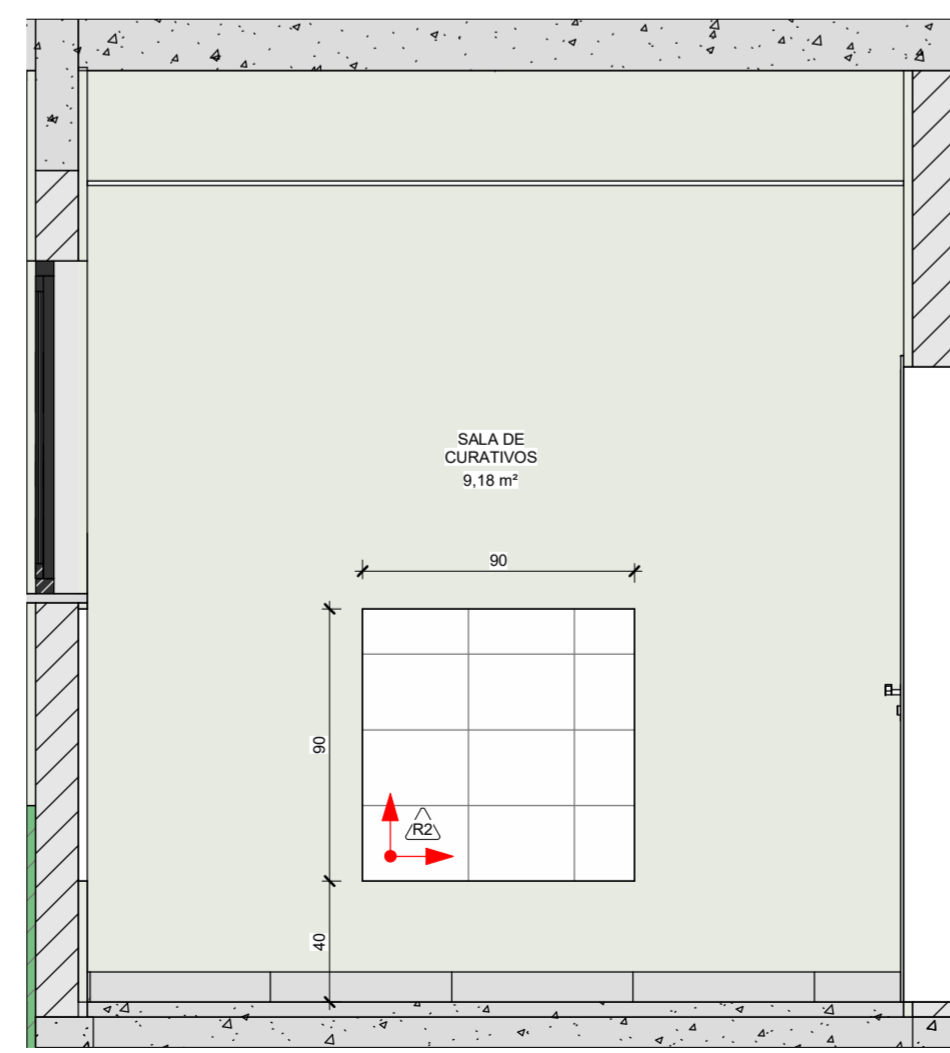
19 PAGINAÇÃO SALA DE CURATIVOS (1) 1 : 25
