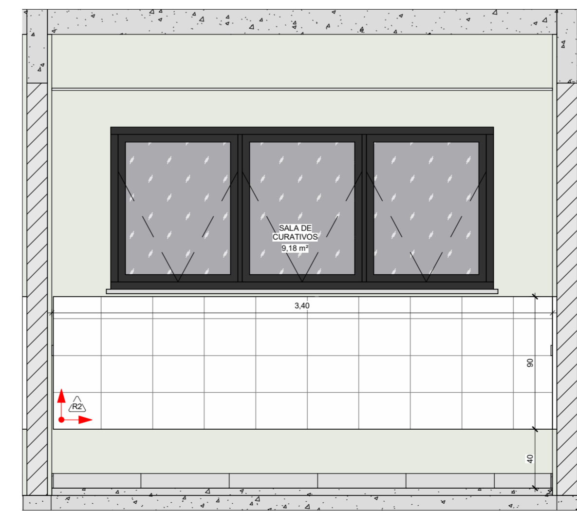
20 PAGINAÇÃO SALA DE CURATIVOS (2) 1 : 25
