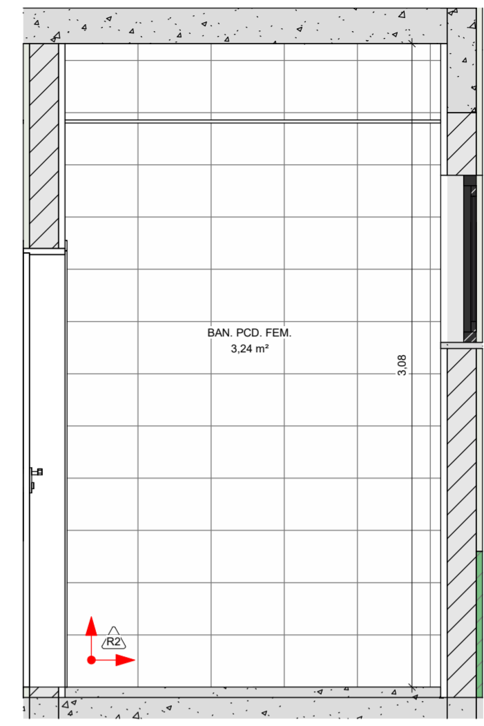
8 PAGINAÇÃO BAN. PNE. FEM. (4) 1 : 25
