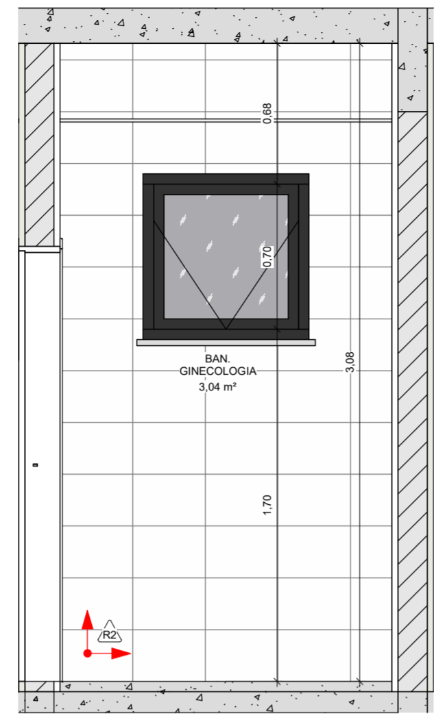
4 PAGINAÇÃO BAN. GINECOLOGIA (4) 1 : 25
