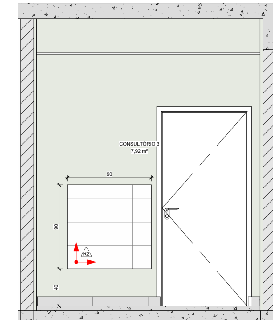
15 PAGINAÇÃO CONSULTÓRIO 3 1 : 25
