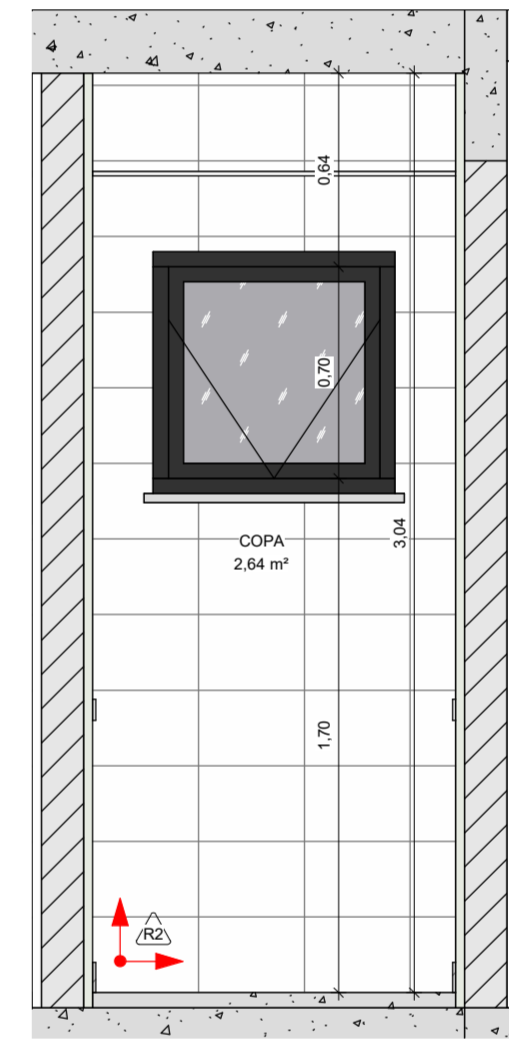
16 PAGINAÇÃO COPA 1 : 25
