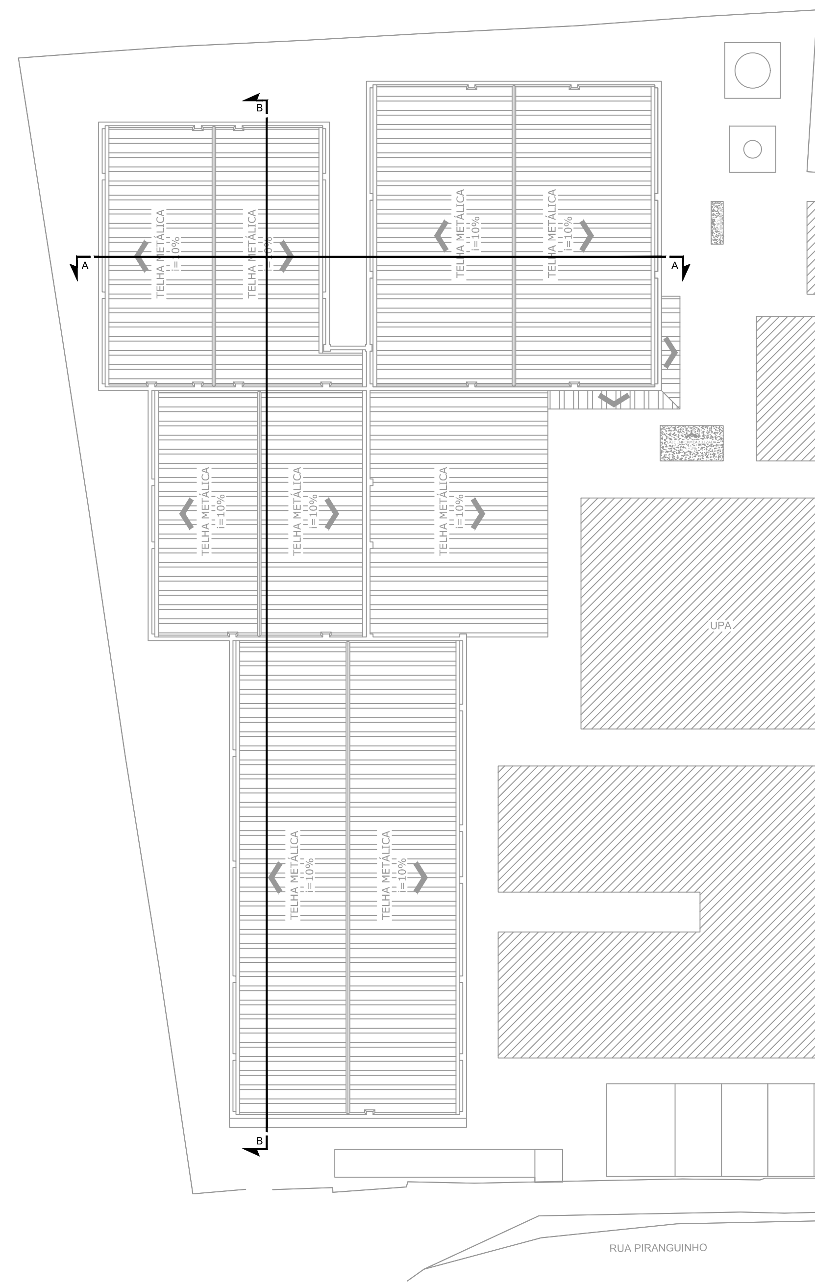
PLANTA BAIXA COBERTURA Escala: 1:200
